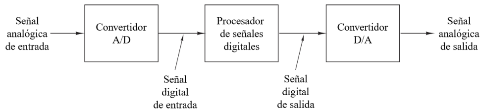
Figura 3. Diagrama de bloques de un sistema de tratamiento digital de señales. [4]
