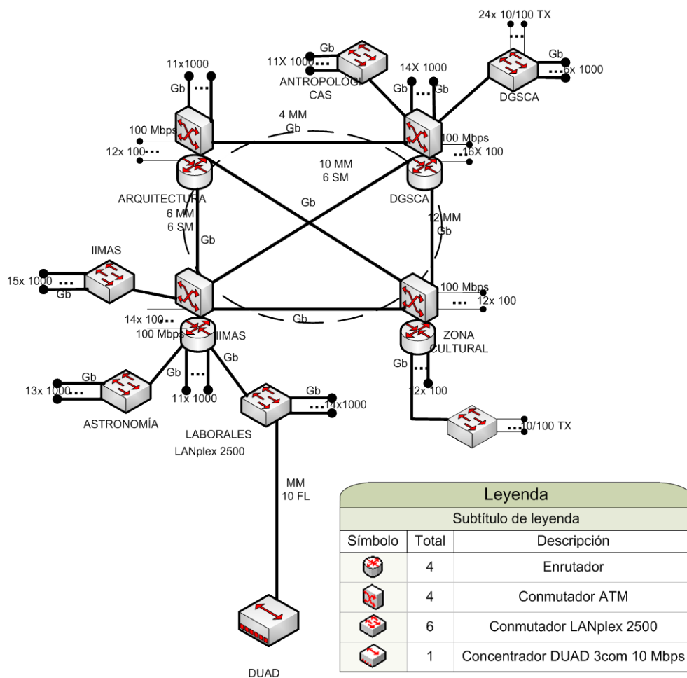
Figura 4.5 Esquema general de la red de cómputo de la DUAD
