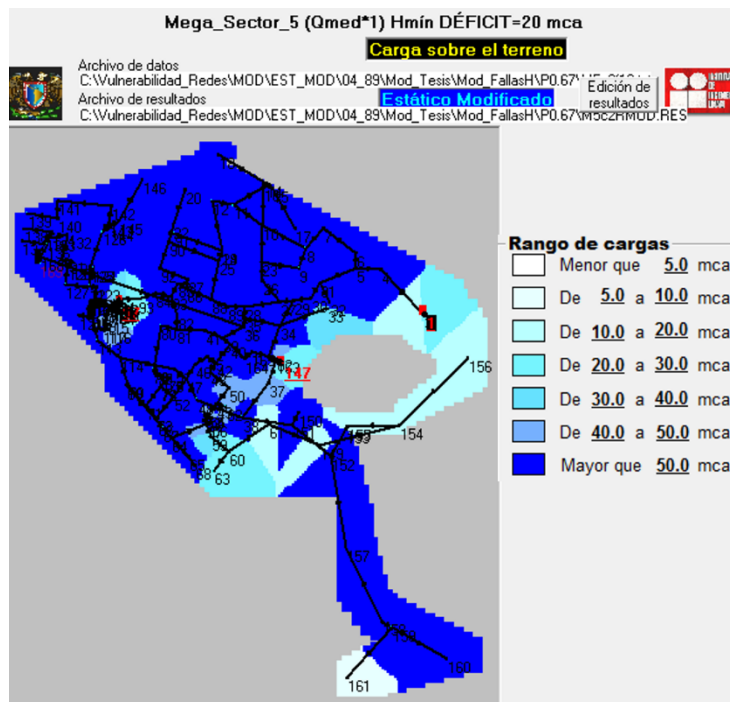
Figura 5-27.- Representación de carga de presión del Megasector 5, con 20 fallas par el sismo de 1989
