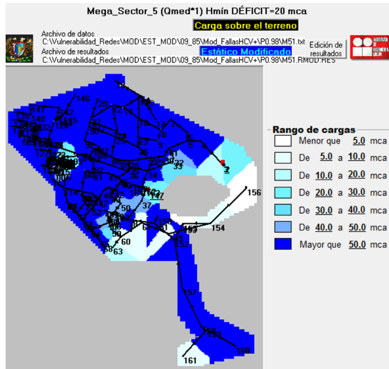
Figura 5-21.- Representación de carga de presión del Megasector 5, sin ninguna falla.
