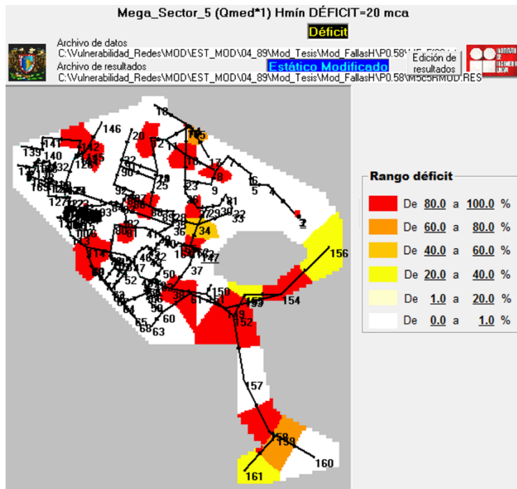
Figura 5-32.-Representación de déficit para el Megasector 5, con 34 fallas por el sismo de 1989.
