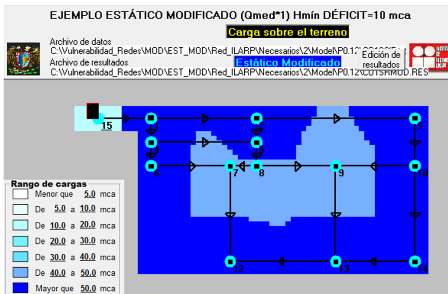
Figura 4-30.-Carga de presión en la red eliminando 2 tuberías y con 5 fugas, combinación de suelo 2.
