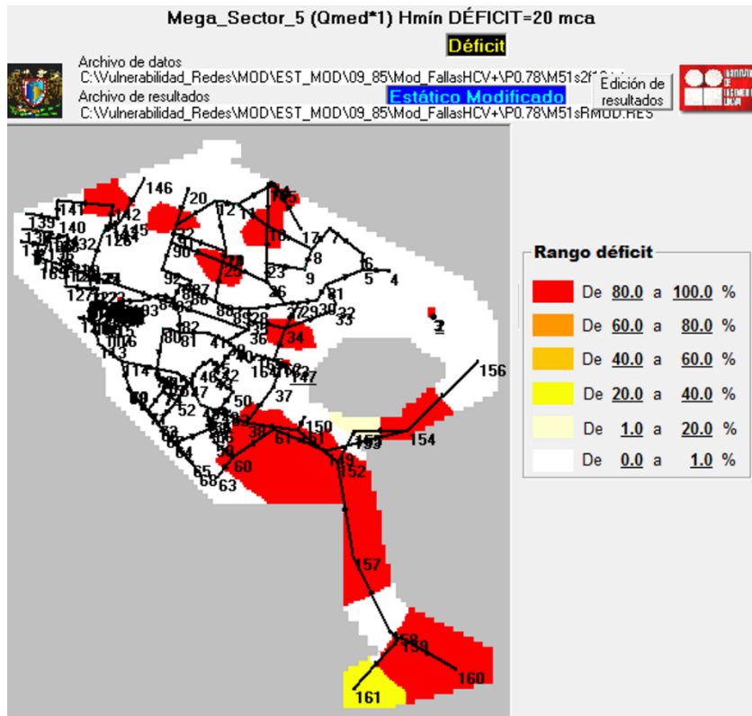
Figura 5-15.- Representación de déficit en el Megasector 5, sin 2 tuberías y 18 fugas.
