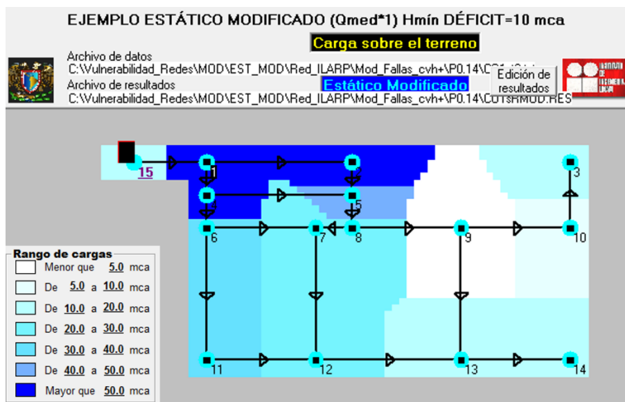
Figura 4-17.- Carga de presión en la red, eliminado 2 tuberías, combinación de suelo 1.
