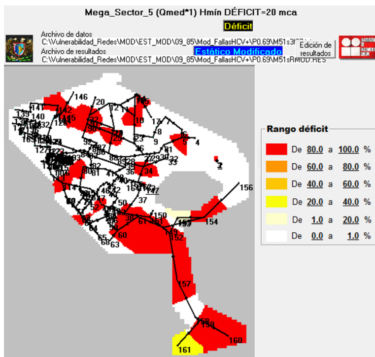
Figura 5-17.- Representación de déficit en el Megasector 5, sin 3 tuberías y 27 fugas
