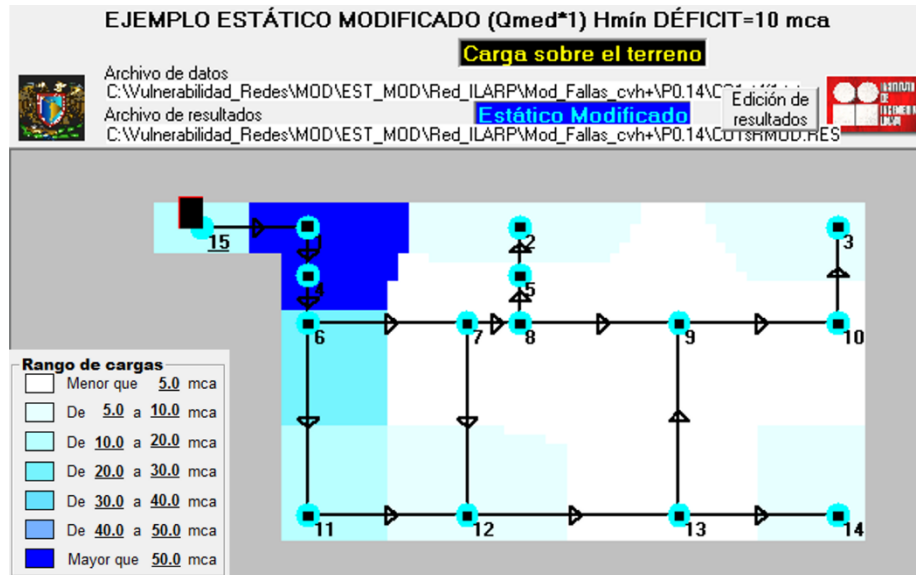
Figura 4-19.-Carga de presión en la red, eliminado 4 tuberías y representando una fuga, combinación de suelo 1.
