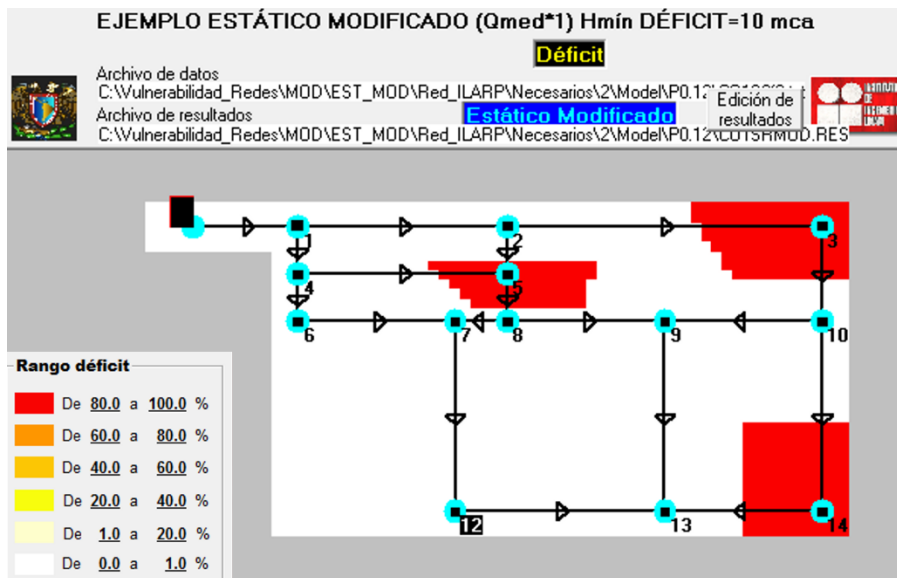
Figura -4-29.-Representación de déficit en la red eliminando 2 tuberías y con 3 fugas, combinación de suelo 2.
