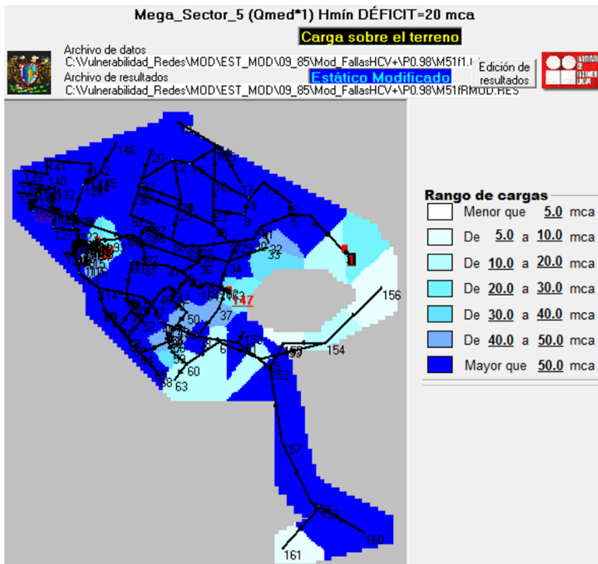
Figura 5-10.- Representación de cargas de presión en el Megasector 5, con una fuga.
