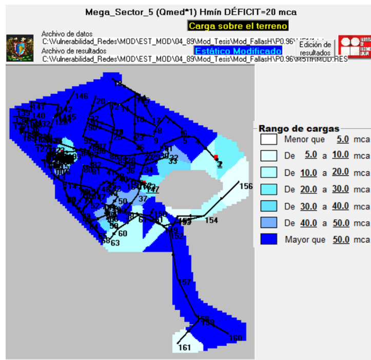
Figura 5-23.- Representaciones de carga de presión del Megasector 5, con una falla por el sismo de 1985
