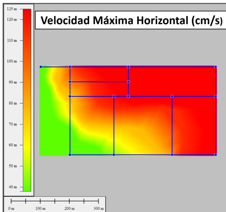
Figura -4-9.- Mapas de velocidad máxima horizontal del suelo para la combinación del suelo 1 en la red de Rosales (2012).
