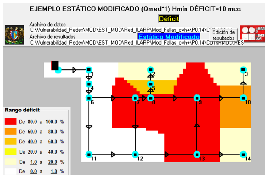
Figura 4-20.-Representación del déficit, eliminado 4 tuberías y representando una fuga, combinación de suelo 1.
