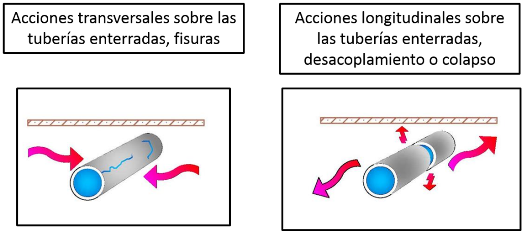
Figura 2-2.-Representación de los movimientos que son resultado de acciones sísmicas
