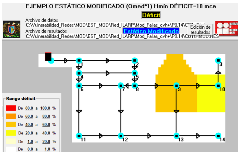
Figura 4-18.- Representación del déficit, eliminando 2 tuberías, combinación de suelo 1.
