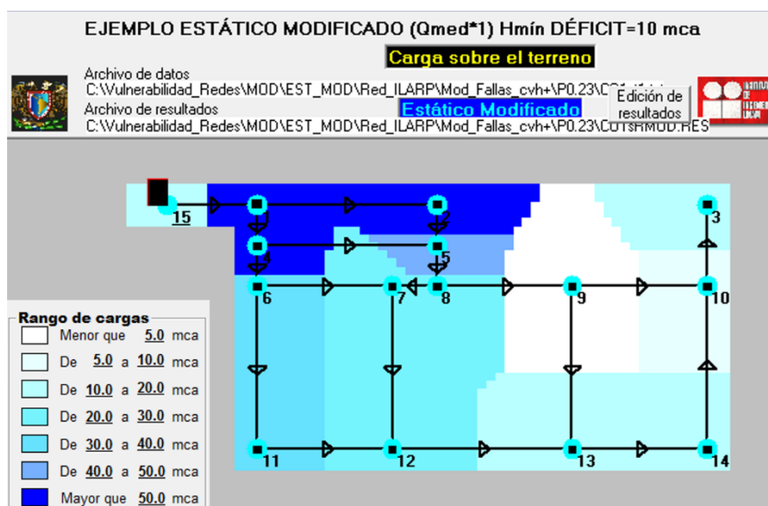
Figura 4-15.- Carga de presión en la red eliminando una tubería, combinación de suelo 1.
