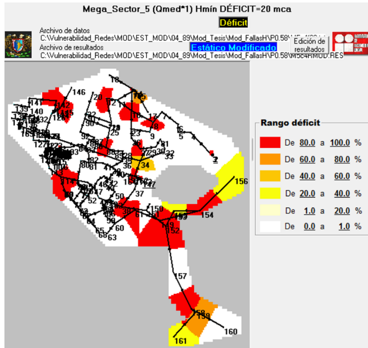
Figura 5-30.- Representación de déficit para el Megasector 5, con 30 fallas por el sismo de 1989.
