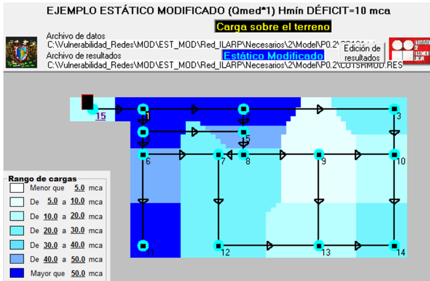
Figura -4-26.-Carga de presión en la red eliminando una tubería, combinación de suelo 2.
