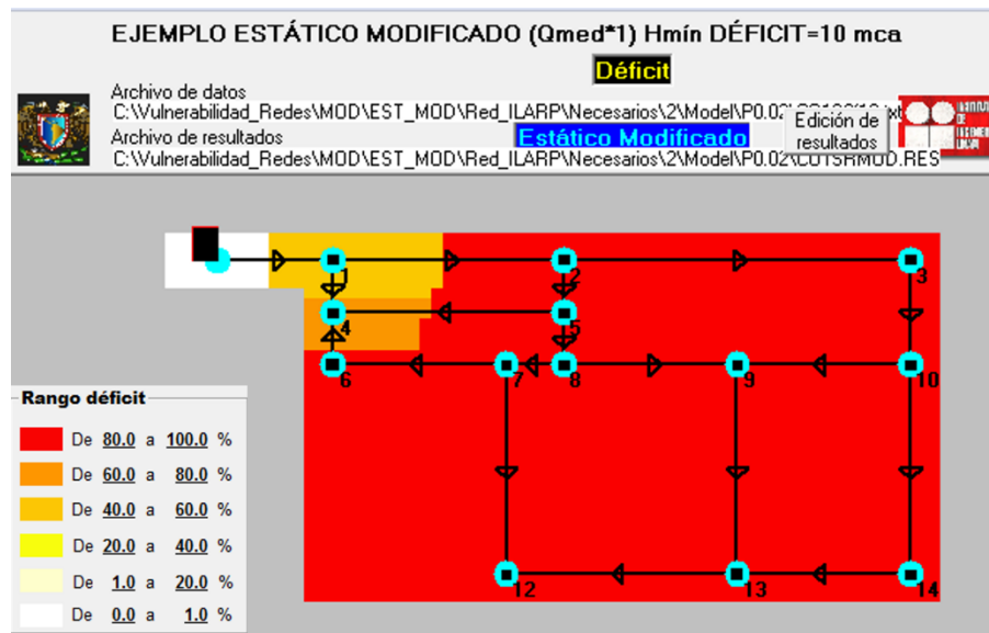
Figura 4-35.-Representación de déficit en la red eliminando 2 tuberías y con 18 fugas, combinación de suelo 2.
