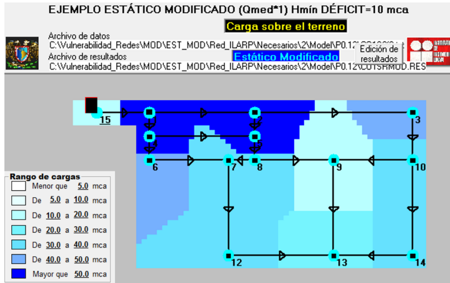
Figura -4-28.-Carga de presión en la red eliminando 2 tuberías y con 3 fugas, combinación de suelo 2.
