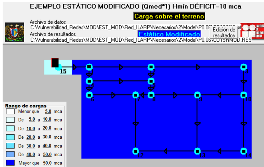
Figura-4-32.-Carga de presión en la red eliminando 2 tuberías y con 13 fugas, combinación de suelo 2.
