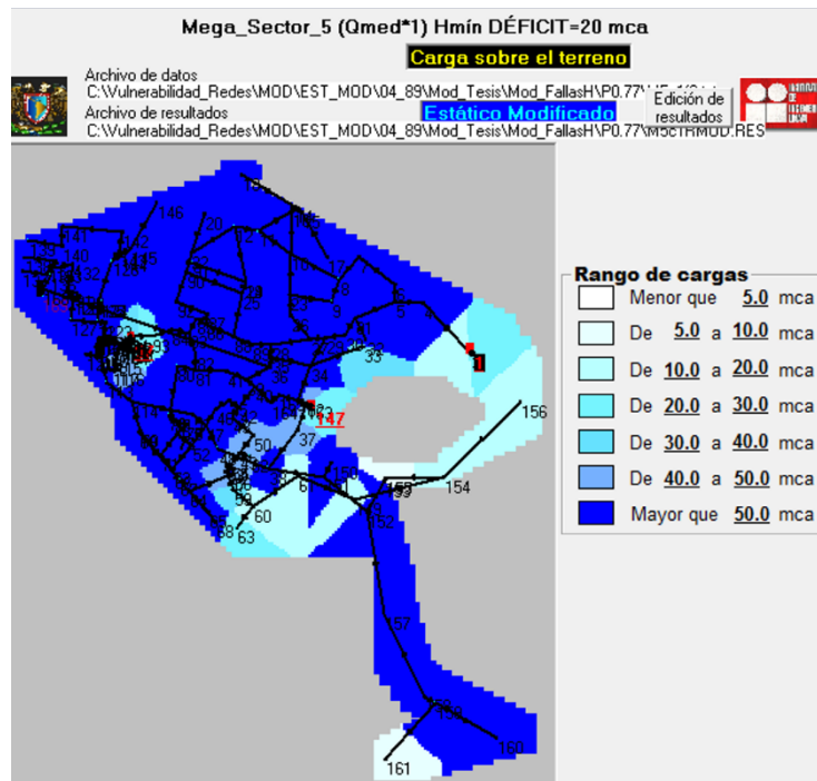
Figura 5-25.-Representación de carga de presión del Megasector 5, con 10 fallas para el sismo de 1989
