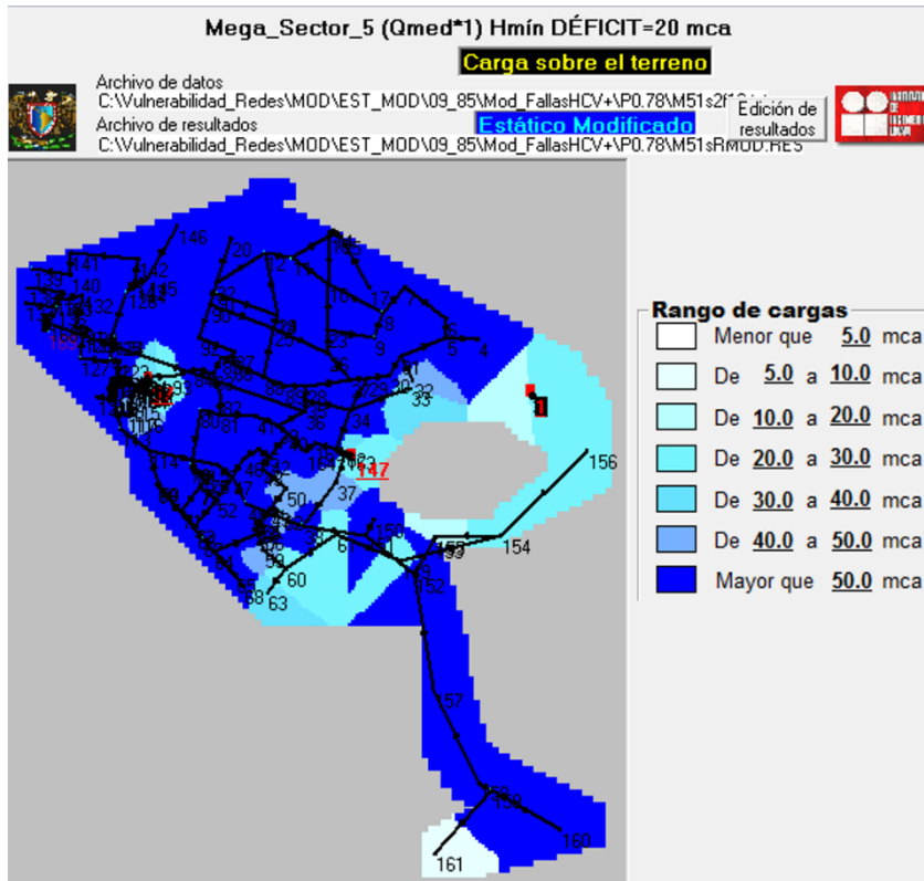
Figura 5-14.- Representación de la representación de carga en el Megasector 5, sin 2 tuberías y 18 fugas.
