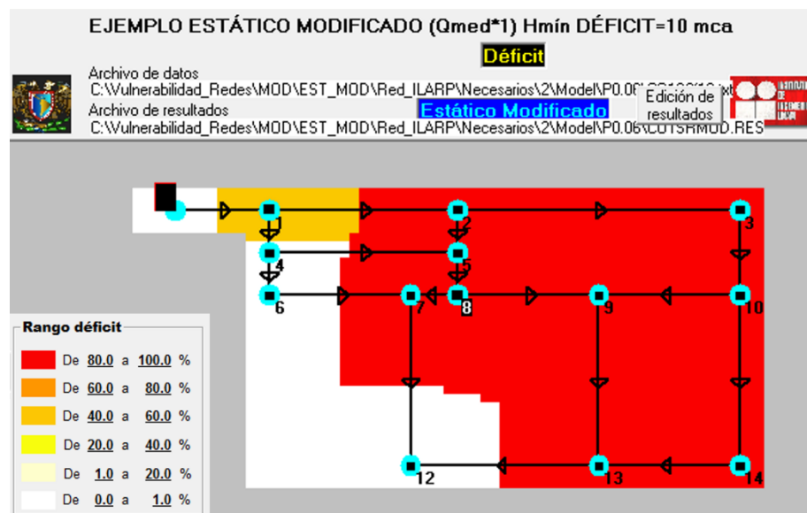
Figura 4-33.-Representación de déficit en la red eliminando 2 tuberías y con 13 fugas, combinación de suelo 2.
