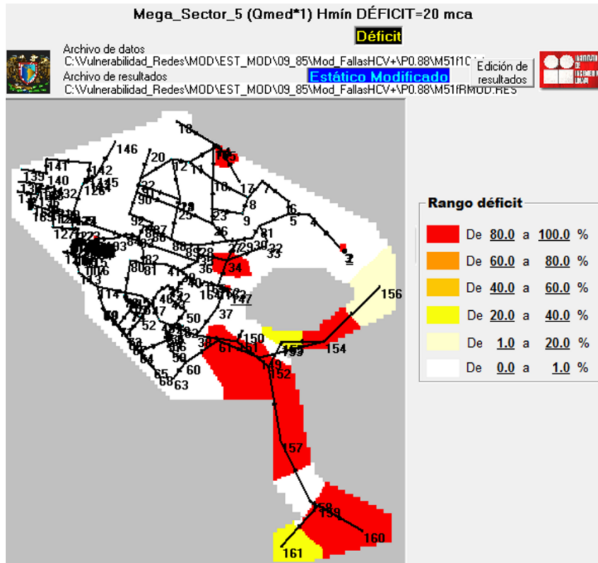
Figura 5-13.- Representación de déficit en el Megasector 5, con 10 fugas.
