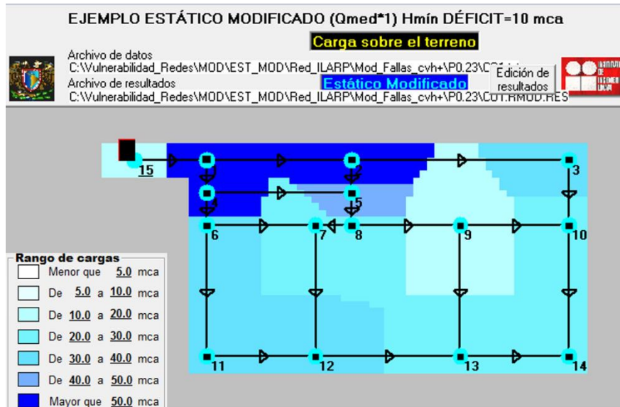
Figura 4-13.- Cargas de presión sobre el terreno en la Red.
