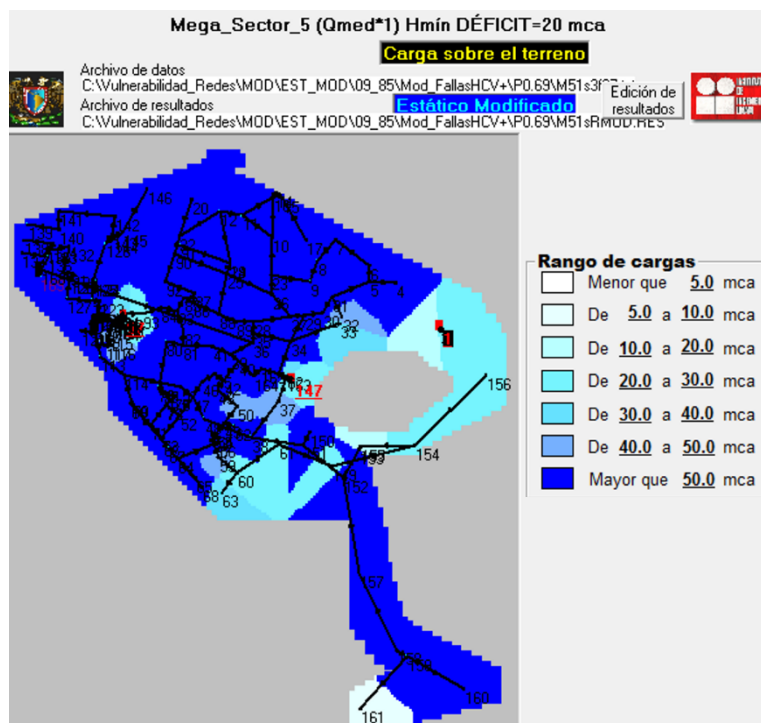
Figura 5-16.- Representación de carga de presión en el Megasector 5, sin 3 tuberías y 27 fugas.
