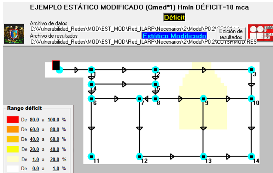
Figura 4-27.-Representación de déficit en la red eliminando una tubería, combinación de suelo 2
