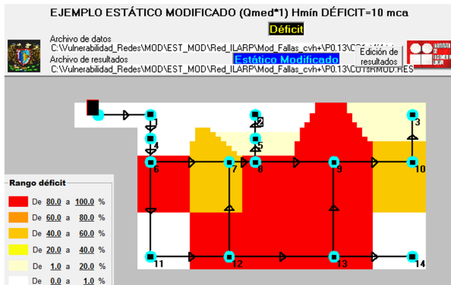
Figura 4-22.-Representación del déficit, eliminado 4 tuberías y representando 4 fugas, combinación de suelo 1.
