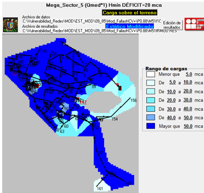
Figura 5-12.-Representación de cargas de presión en el Megasector 5, con 10 fugas.
