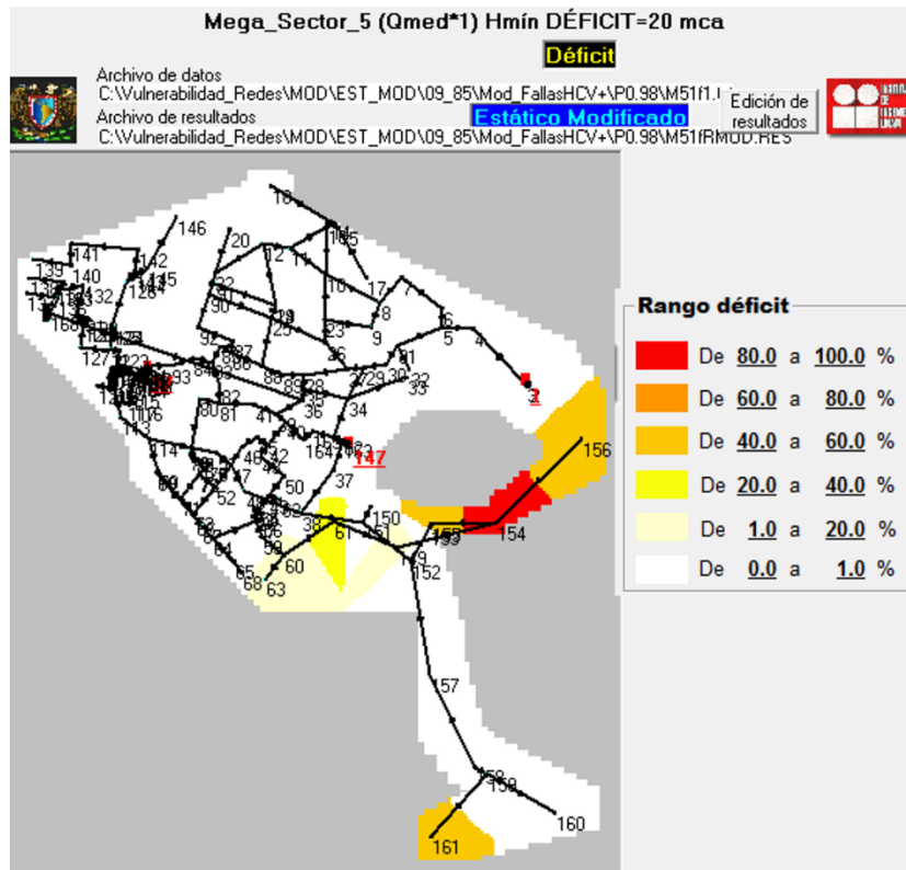
Figura 5-11.- Representación de déficit en el Megasector 5, con una fuga.
