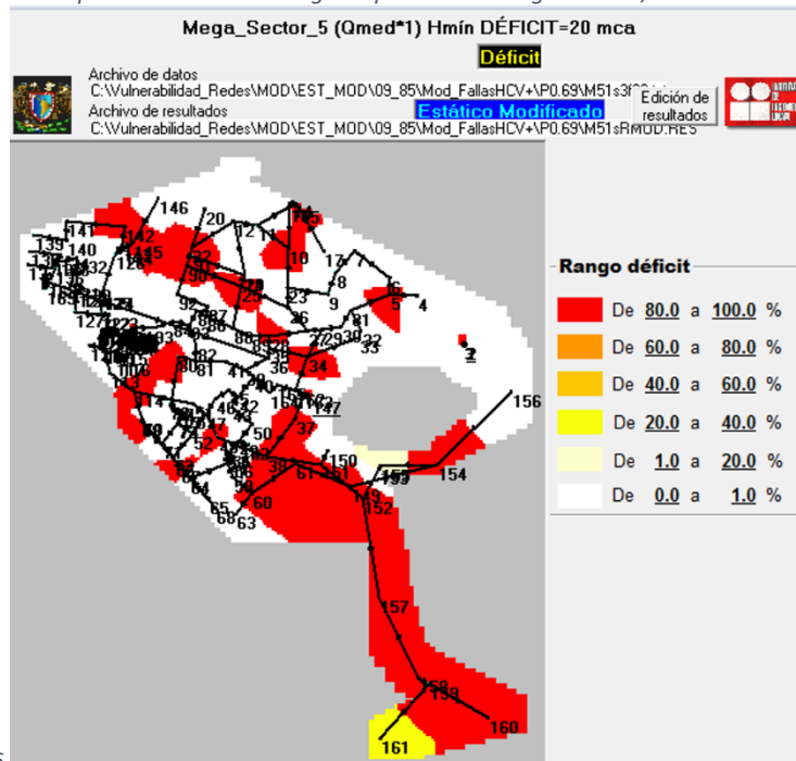
Figura 5-18.- Representación de la carga de presión del Megasector 5, sin 5 tuberías y 35
