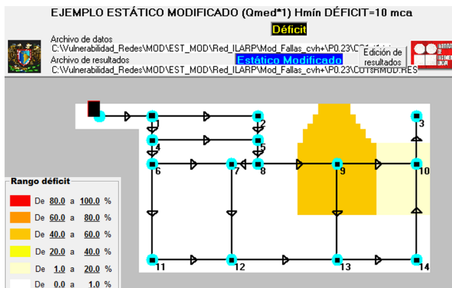
Figura 4-16.-Representación del déficit en la red, eliminando una tubería, combinación de suelo 1.
