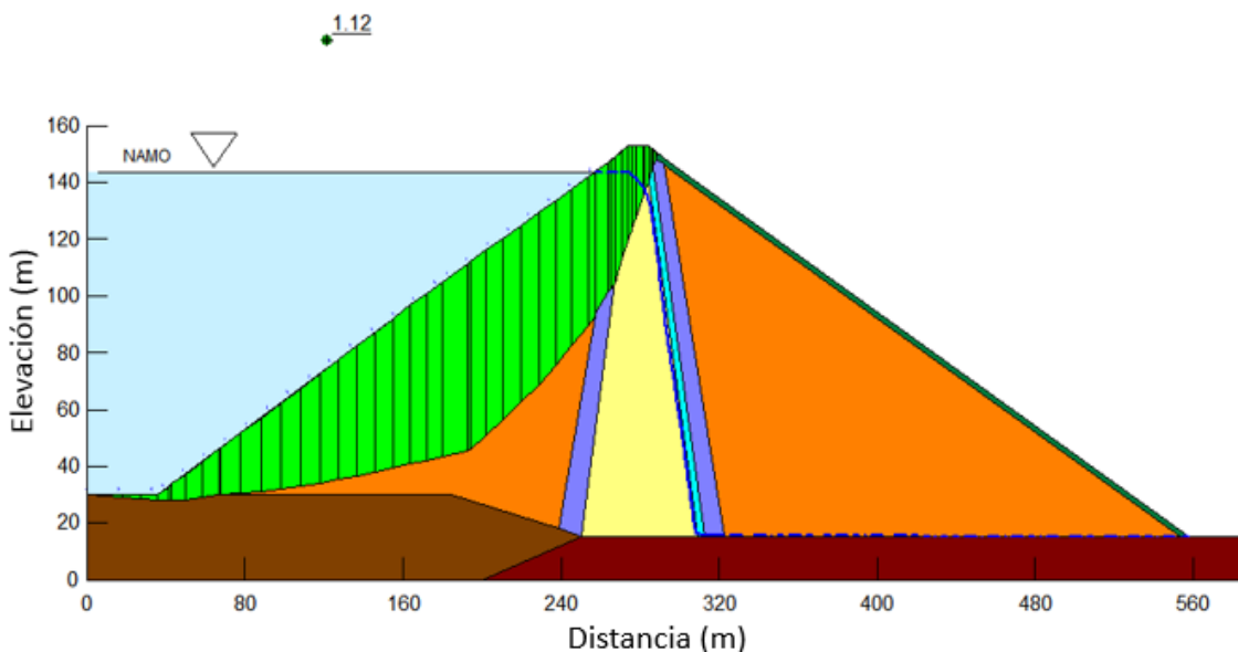
Figura 6.50 Envolvente de falla talud aguas arriba por el método de M-P con flujo establecido en el NAMO (análisis pseudo-estático)
