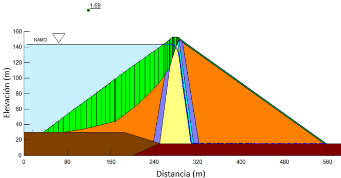
Figura 6.49 Envolvente de falla talud aguas arriba por el método de M-P con flujo establecido en el NAMO (análisis estático)
