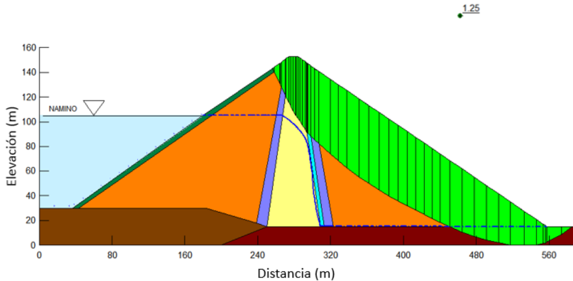
Figura 6.52 Envolvente de falla talud aguas abajo por el método de M-P con flujo establecido en el NAMINO (análisis seudo-estático)
