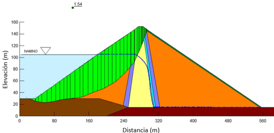
Figura 6.53 Envolvente de falla talud aguas arriba por el método de M-P con flujo establecido en el NAMINO (análisis estático)
