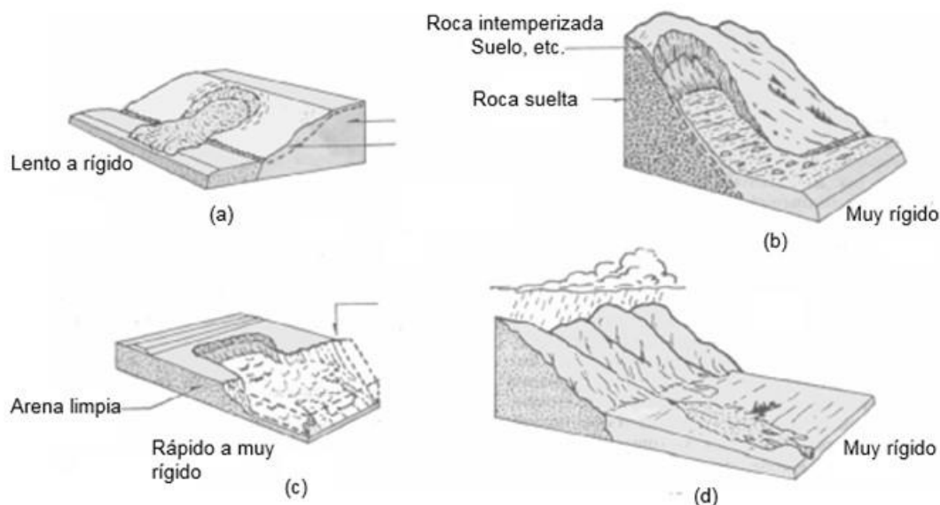
Figura 4.7 Falla por flujo (Rico, 2000)
