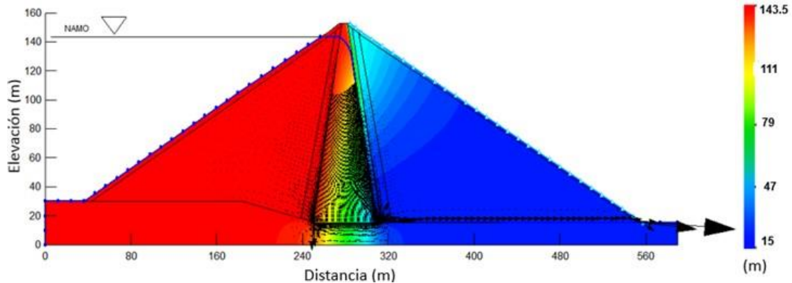
Figura 6.23 Distribución de las fuerzas de filtración en el cuerpo de la cortina de la presa (a la altura del NAMO)
