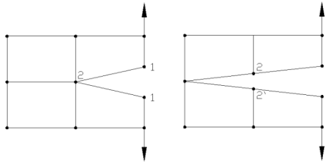
Fig. 2.3 Modelo de grieta discreta
