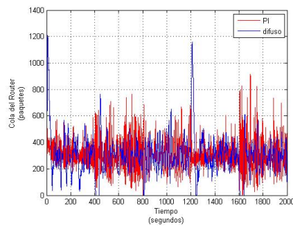
(f) Respuesta del PI para \tau = 0,8
