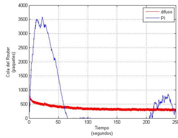
(e) Controlador diseñado para \tau = 0,8
