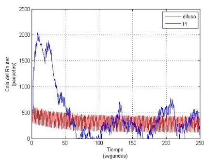
(d) Controlador diseñado para \tau = 0,7
