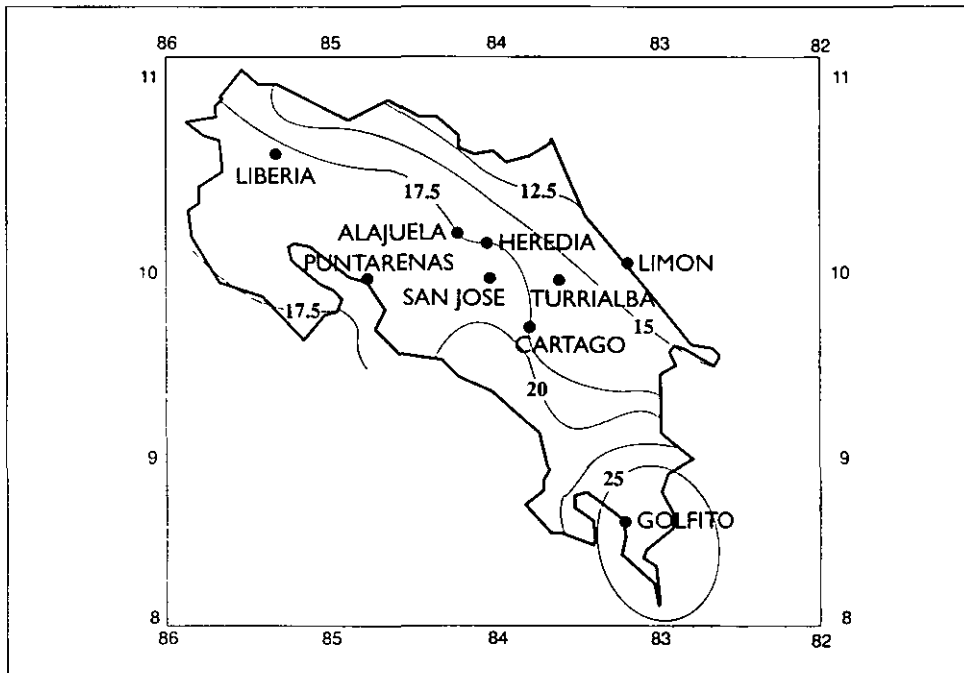
Figura A2 Isoaceleraciones para periodo de retorno de 100 años
