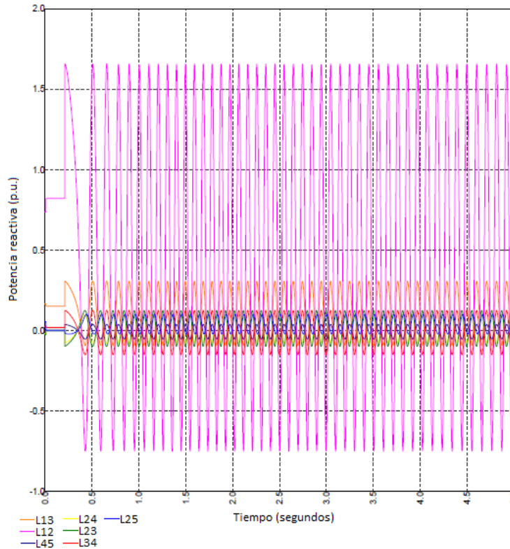
Figura 4.12: Flujos de potencia reactiva a través de las líneas de transmisión, falla liberada a 0.2 segundos.
