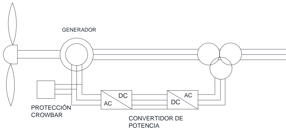
Figura 2.1: Generador de inducción doblemente alimentado.
