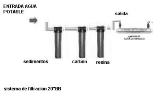
Figura 38. Sistema de filtración 20" BB (H2OZONI, 2023).
