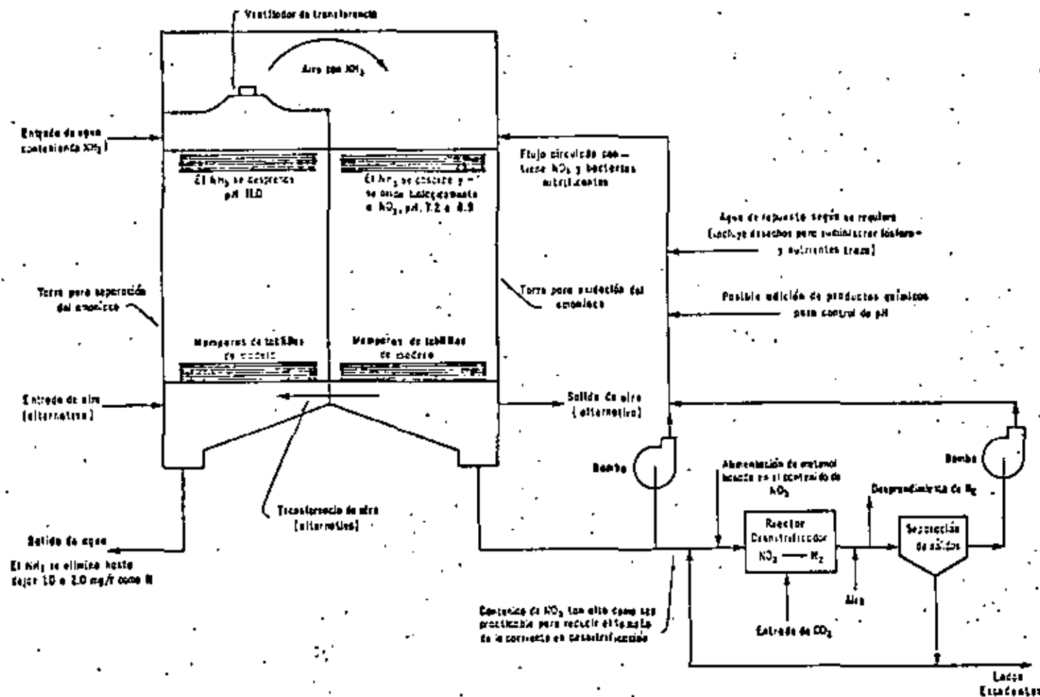
Fig 8 Sistema de eliminación de amoníaco
