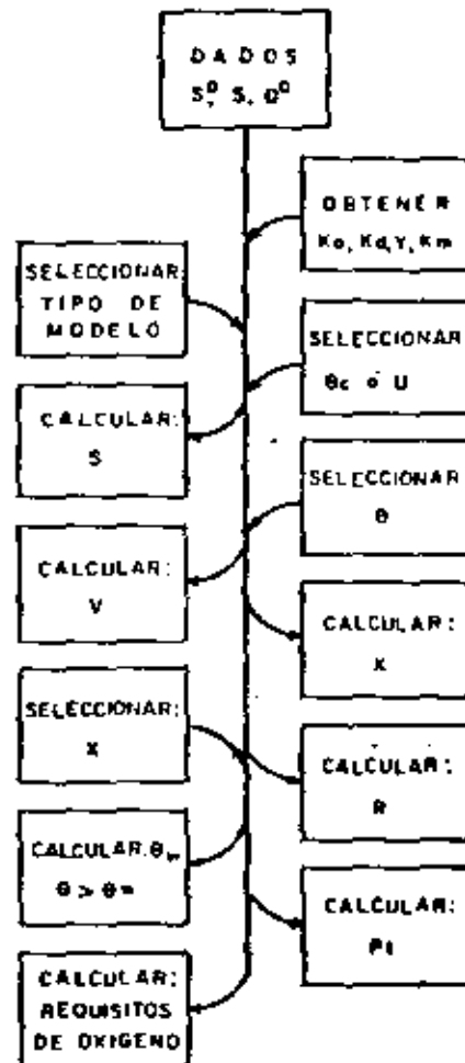
RESUMEN DE DISEÑO BASADO EN EDAD DE LODOS
