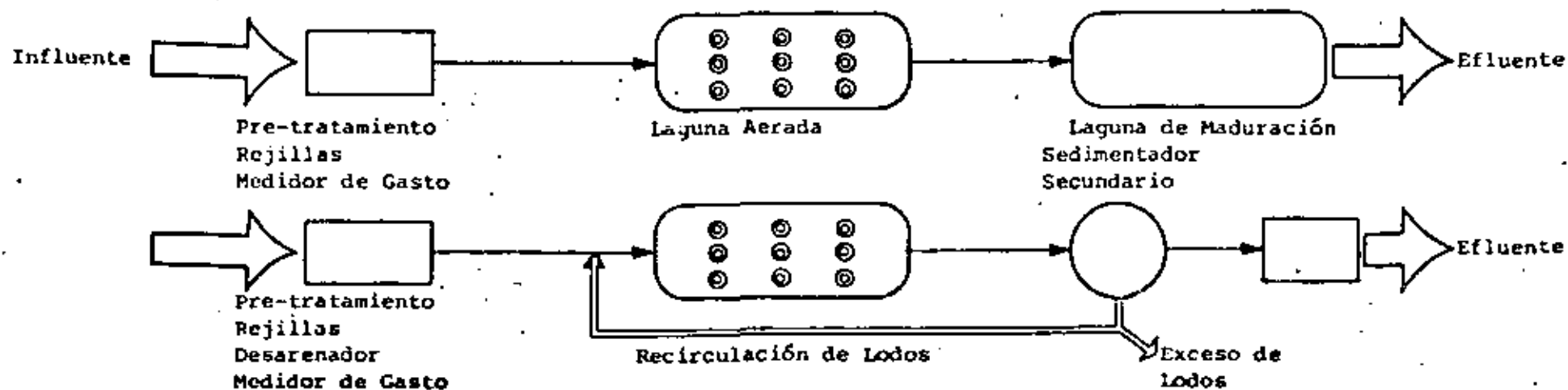
Fig. 2 VARIANTES DEL SISTEMA DE LAGUNAS AERADAS
