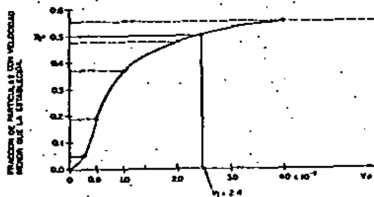
Fig. 4- CURVA ANALITICA DE VELOCIDADES DE SEDIMENTACIÓN.
