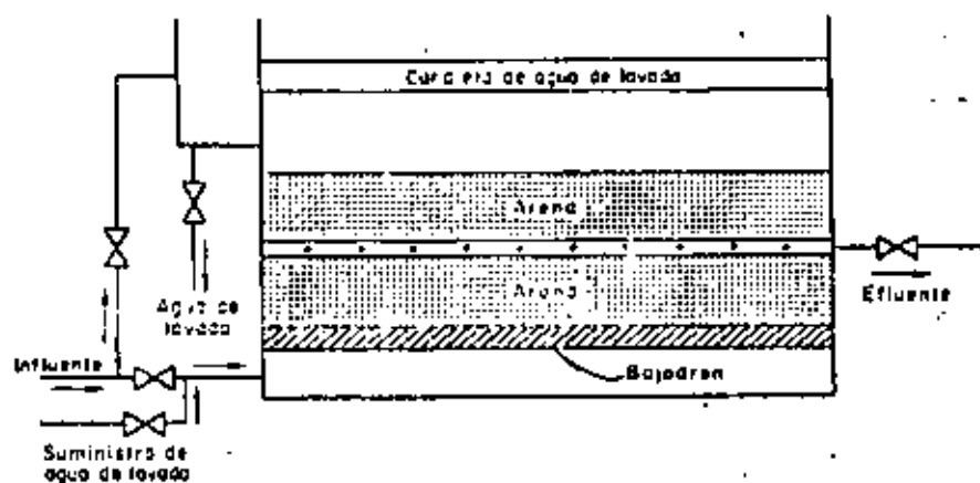
Filtro con doble flujo. Medio único
