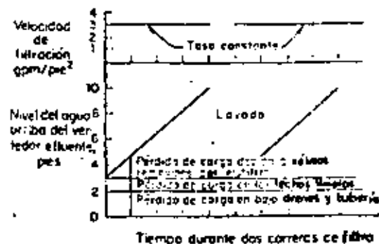
Tasa de filtración, nivel del agua y pérdida de carga durante dos carreras de filtración
