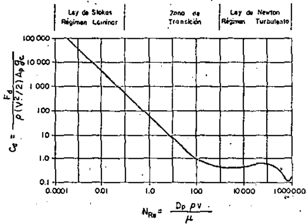
Fig. 1:- COEFICIENTE DE ARRASTRE, C_d , PARA PARTICULAS ESFÉRICAS.
