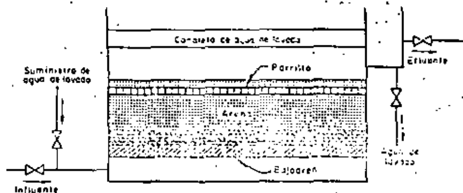
Filtro flujo ascendente con parrilla
