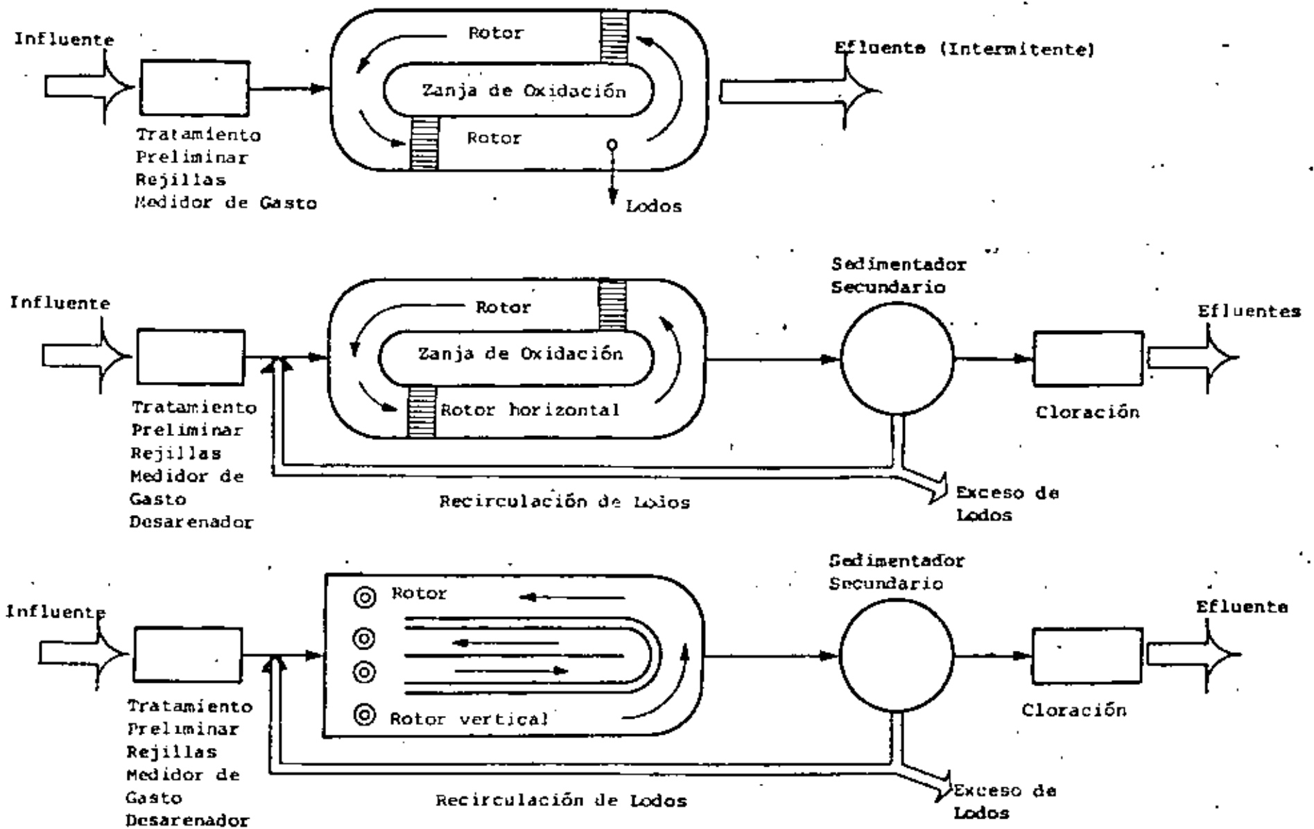
Fig. 3 ESQUEMAS DE SISTEMAS DE ZANJAS DE OXIDACION
