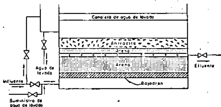
Filtro con doble flujo. Dos medios
