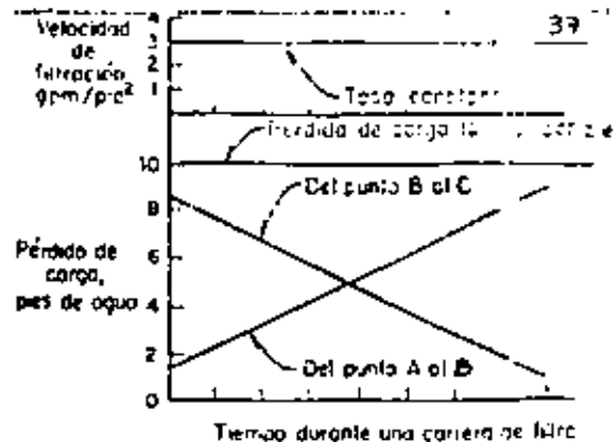
Tasa de filtración y pérdida de carga durante una carrera de filtro
