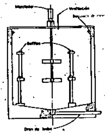
Fig. 3.1- MEZCLADOR TÍPICO USADO EN PLANTAS DE TRATAMIENTO DE AGUAS NEGRAS.
