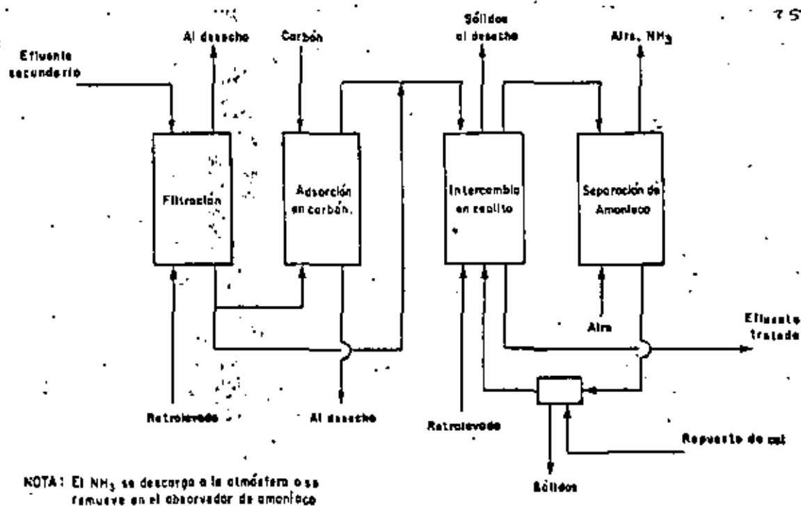
Fig 8 Sistema de eliminación de amoníaco
