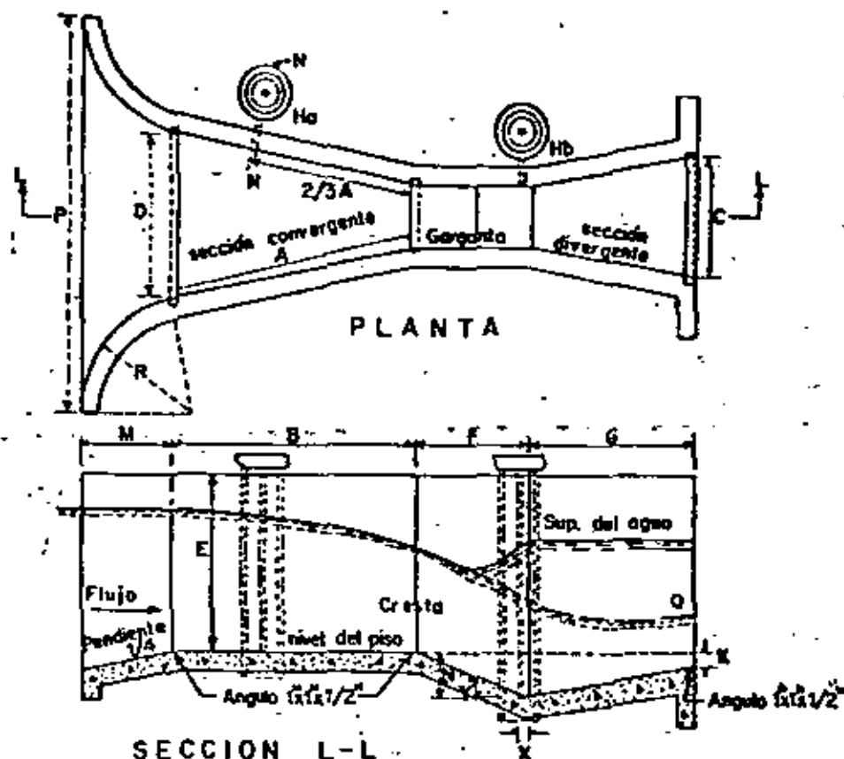
FIG. N° 7-DIMENSIONES Y MEDIDAS DEL MEDIDOR PARSHALL PARA VARIOS TAMAÑOS DE GARGANTAS, W
