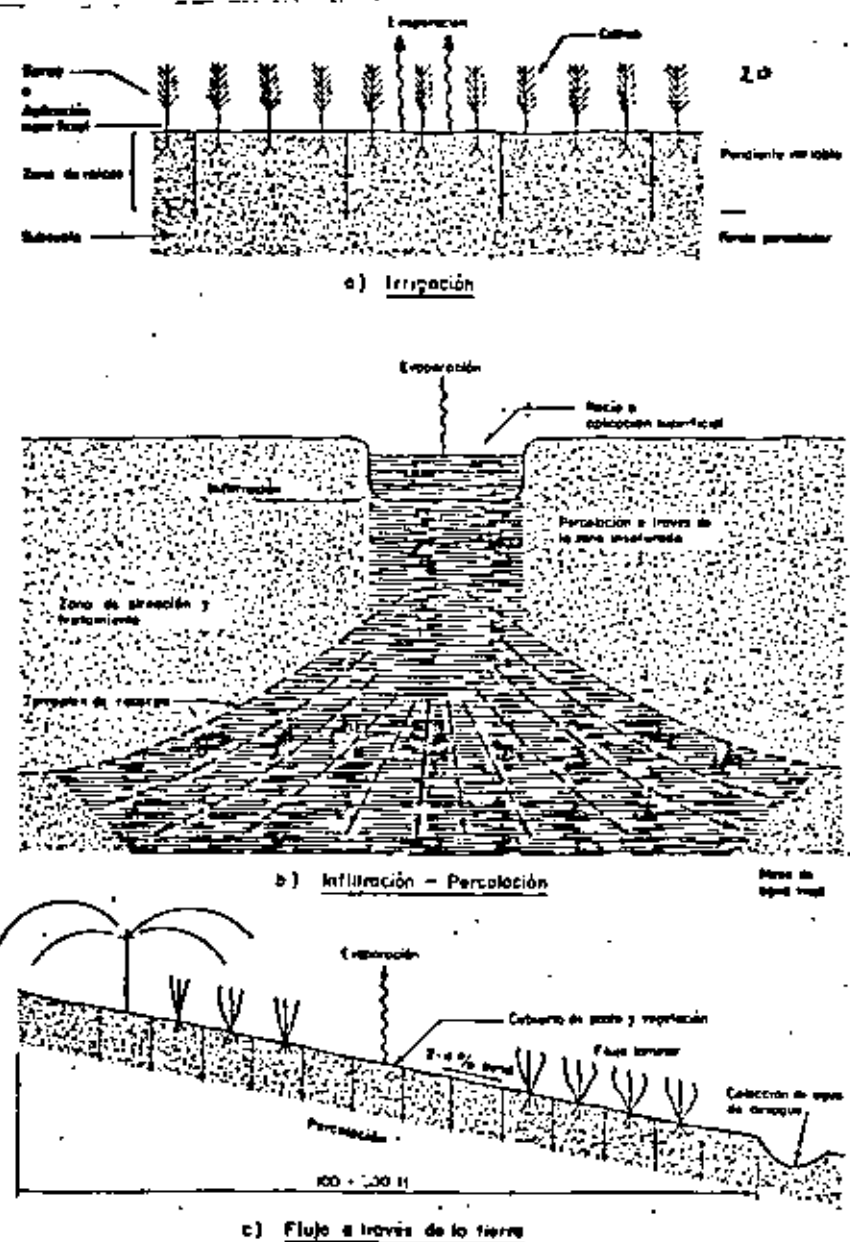
Fig. 1- METODOS DE DISPOSICION EN TIERRA DE AGUAS RESIDUALES.
