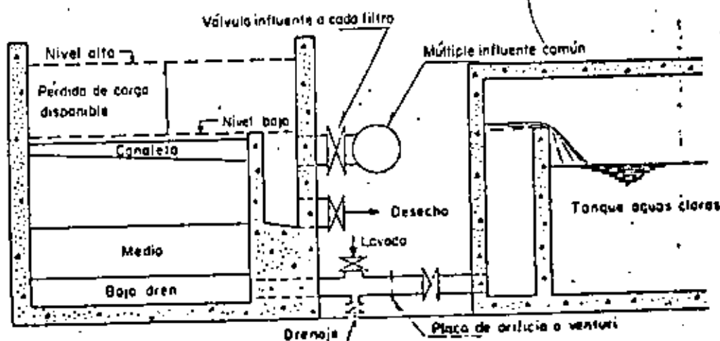
Filtro para operación con tasa variable descendente
