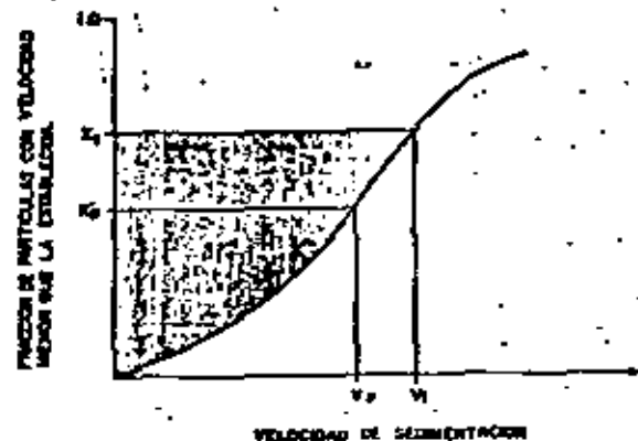
Fig. 3- CURVA DE VELOCIDADES DE SEDIMENTACIÓN PARA PARTICULAS DISCRETAS.
