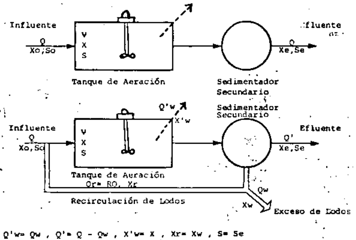
Fig. 4 DIAGRAMAS DE SISTEMAS AEROBICOS COMPLETAMENTE MEZCLADOS SIN Y CON RECIRCULACION DE LODOS
