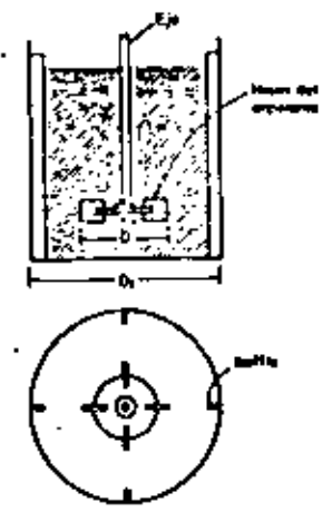
Fig. 3.2- MEZCLADOR DE TURBINA Y TANQUE CON 'BAFFLES'.
