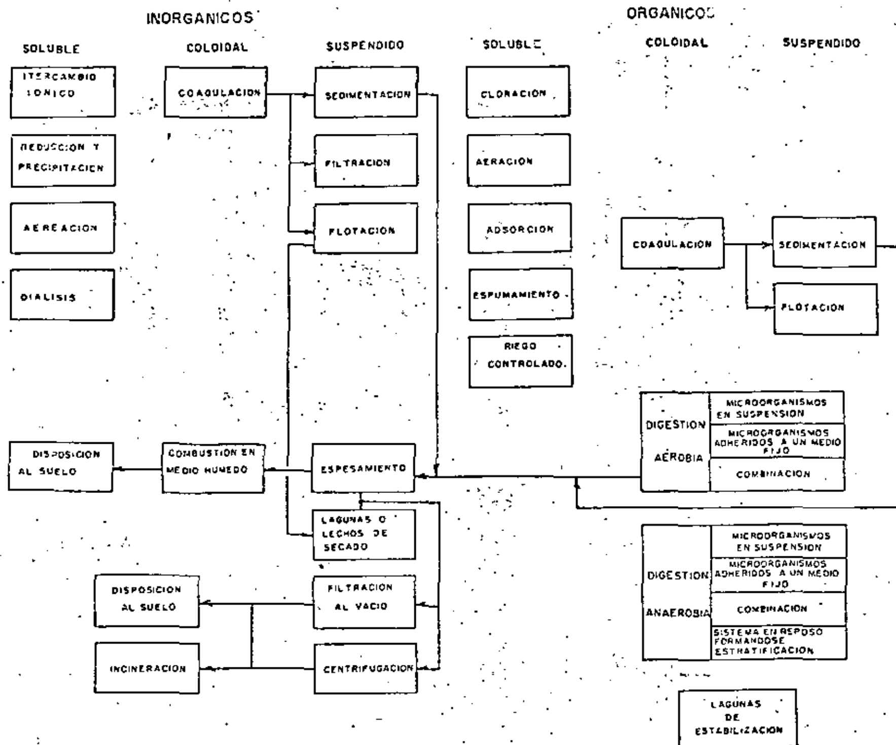
FIGURA 1.- SISTEMAS DE TRATAMIENTO DE ACUERDO CON EL CONTAMINANTE A REMOVER.
