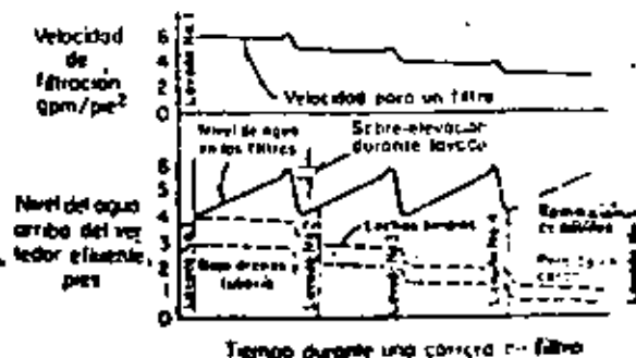
Tasa de filtración, pérdida de carga y nivel del agua durante una carrera de filtro en una planta con 4 filtros
