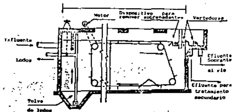
Figura 1. Tanque de Sedimentación Primaria Rectangular
