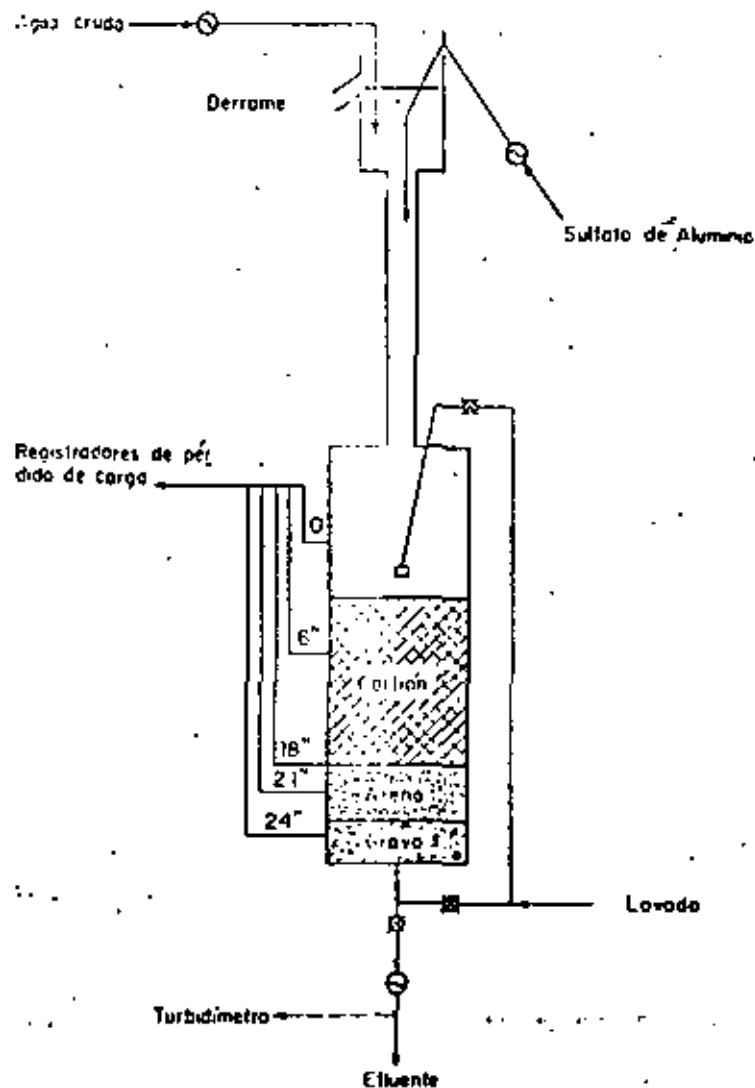
Detalles de un filtro experimental
