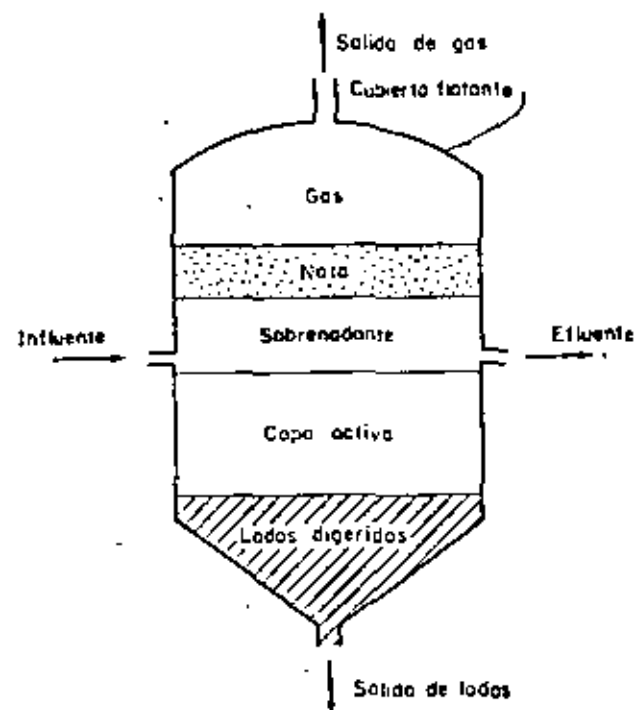
Fig. 3-5 Esquema de un proceso de digestión anaerobia de baja eficiencia o Standard-rate
