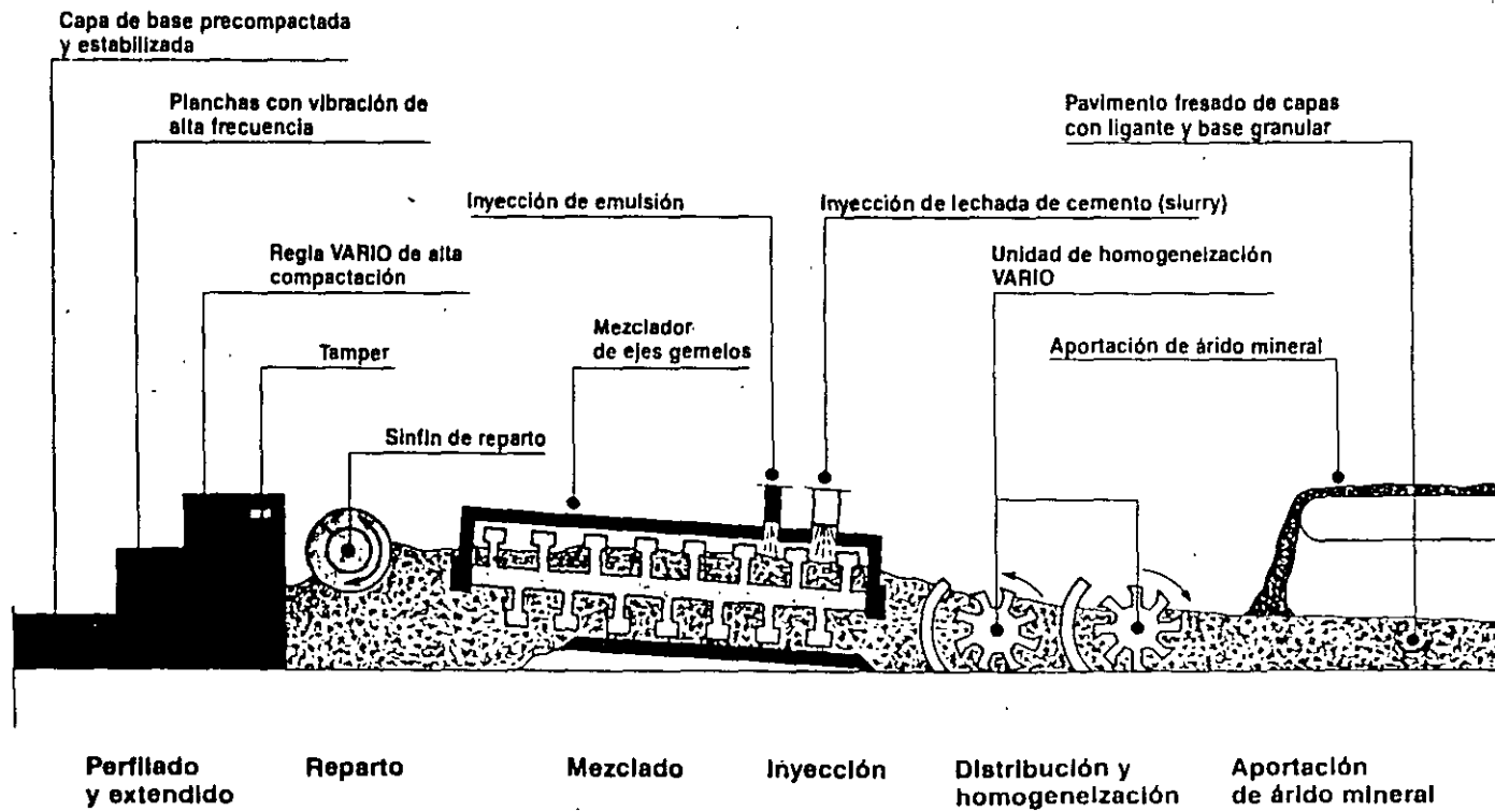
Principio de trabajo del proceso tal como lo realiza la recicladora en frío CR 4500.
