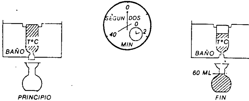
VISCOSIDAD SAYBOLT-FUROL 160 SEG. A T°C
