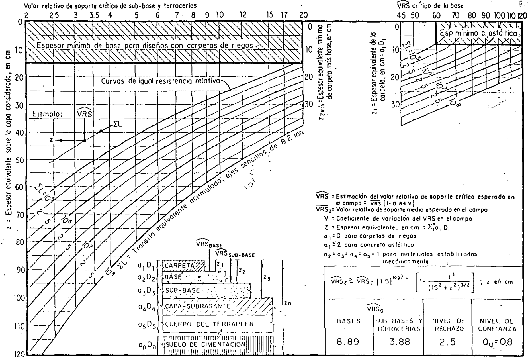
Fig A6. Gráfica para el diseño estructural de carreteras con pavimento flexible
