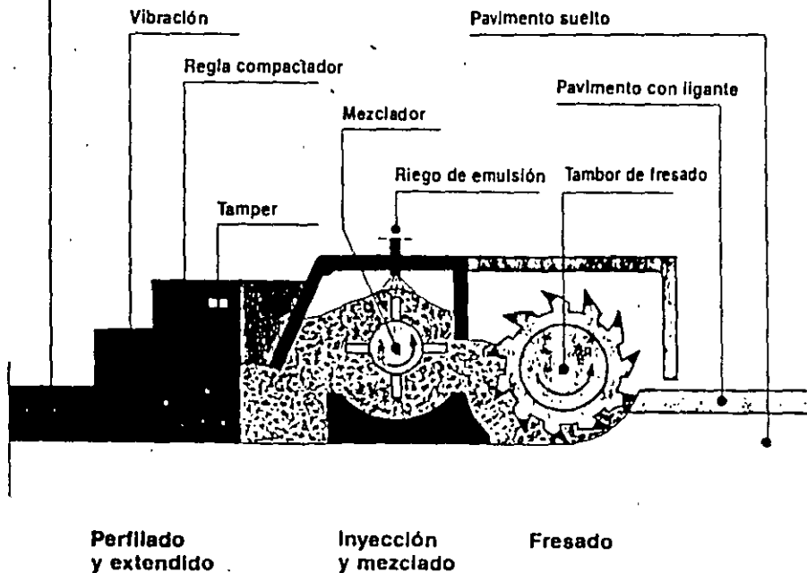
Principios de funcionamiento de la recicladora en frío 1000 CR.
