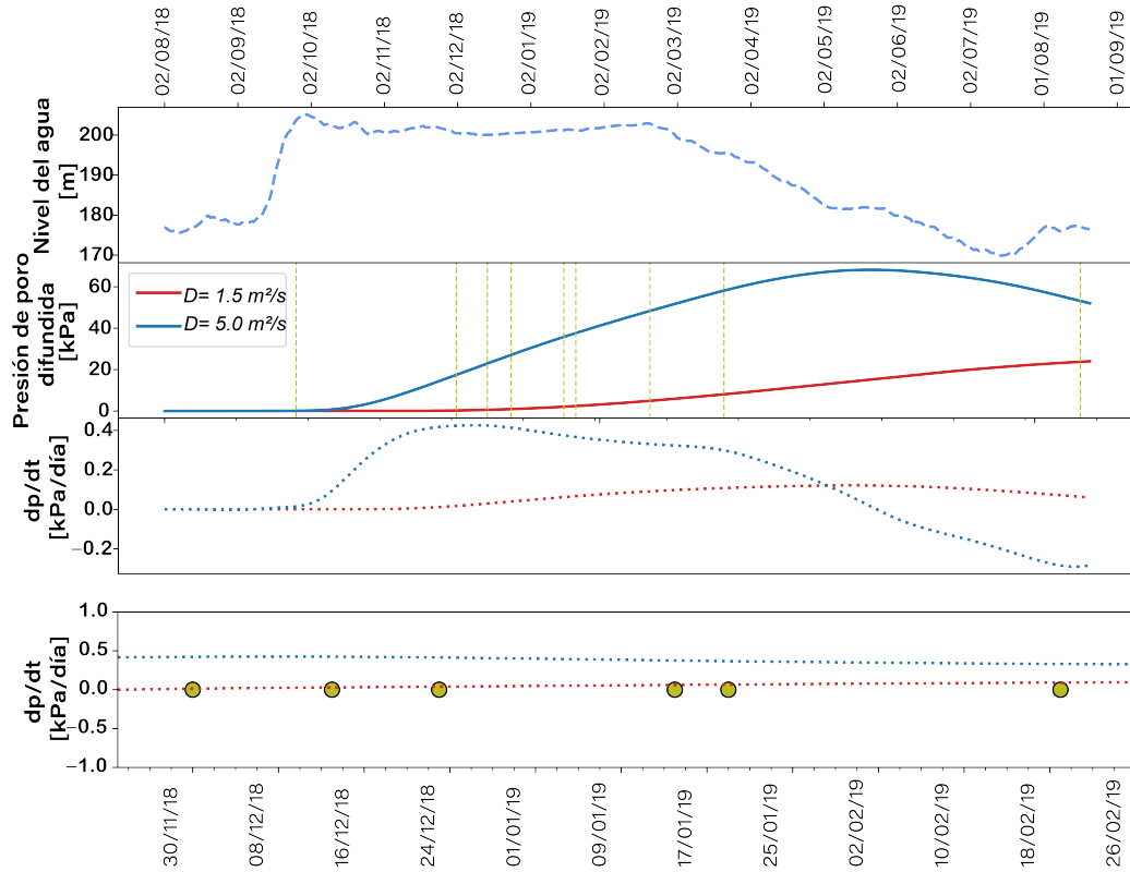
Figura 5.13: Análisis de presión de poro a 15 km de la presa La Yesca, para valores de difusividad hidráulica 1.5 (rojo) y 5.0 \text{m}^2/\text{s} (azul). En el primer panel se muestra la historia de llenado de la presa; en el segundo, la presión de poro; en el tercero, la derivada de la presión de poro; y en el cuarto, la sección de la curva en la etapa de mayor actividad sísmica, diciembre de 2018-abril de 2019. Las líneas y círculos color olivo marcan el día en que ocurrieron los eventos seleccionados (Tabla 4.2).
