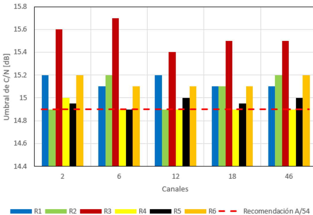
Figura 4.4: Resultados de prueba de Umbral de C/N [dB] con una potencia de recepción débil, -68 dBm.
