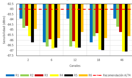
Figura 1. Sensibilidad de los receptores para cada uno de los canales de evaluación.
