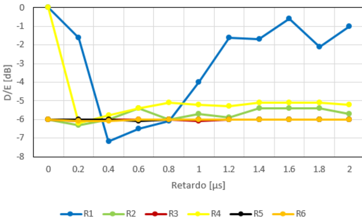
Figura 4.8: Tolerancia entre una señal principal y un Eco Dinámico a 1 Hz en un rango de 0-2 \mu s.
