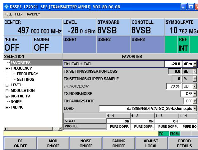
Figura 3.2: Panel principal de operación del equipo generador SFE de R&S®.
