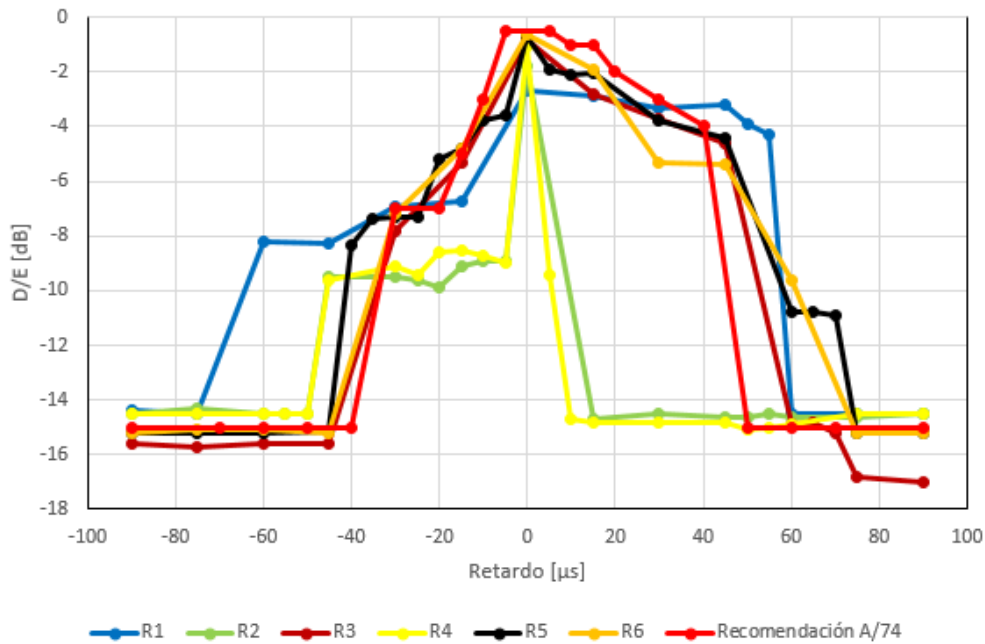
Figura 4.25: Respuesta de los receptores ante un eco desplazado 120 km/h.
