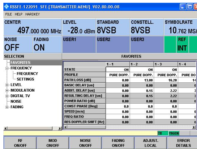
Figura 3.3: Tabla de paths del equipo generador SFE de R&S®.
