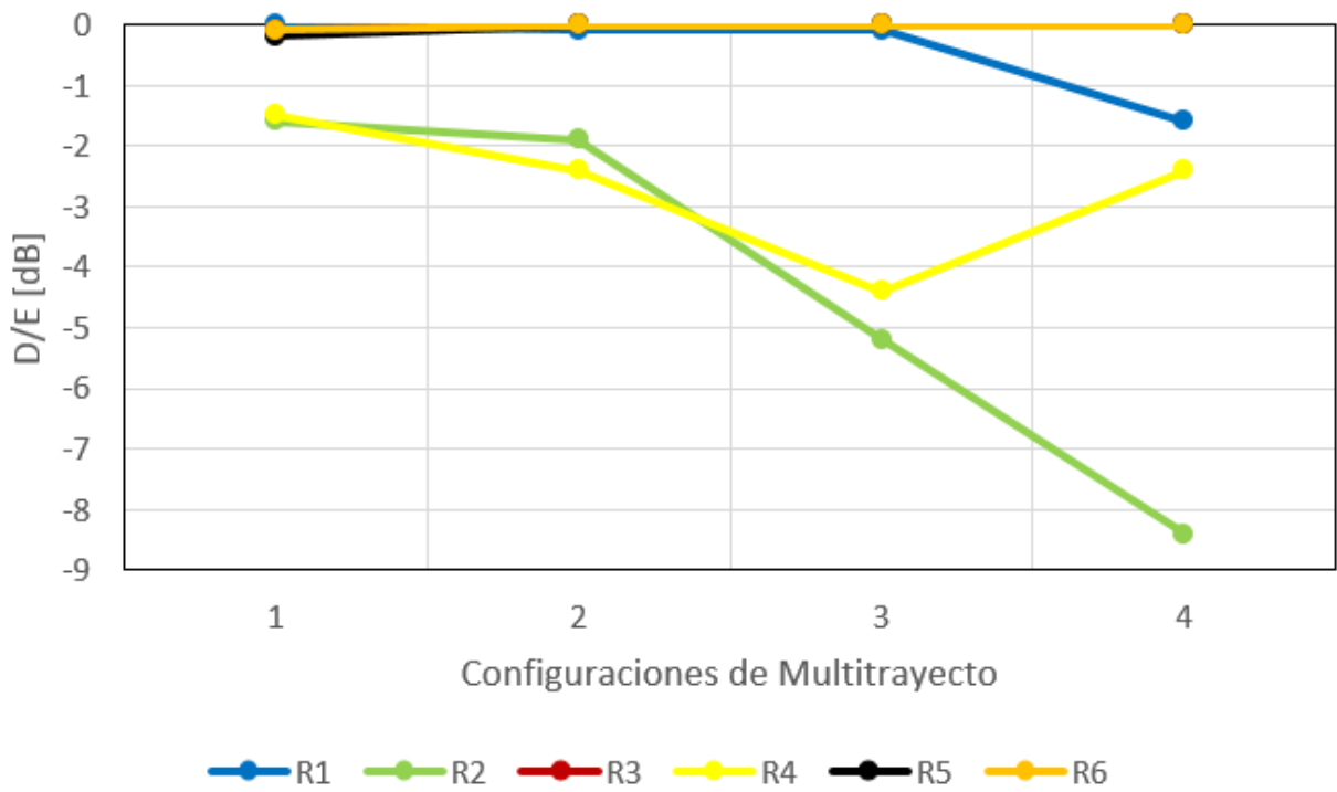
Figura 4.13: Tolerancia a Múltiples Ecos Dinámicos (Path 5 a 1 Hz).
