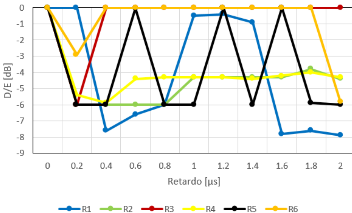
Figura 4.7: Tolerancia entre una señal principal y un Eco Dinámico a 0.5 Hz en un rango de 0-2 \mu s.
