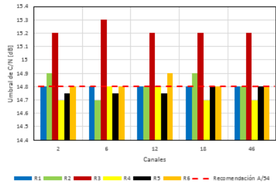
Figura 3. Umbral de C/N para -53 dBm de potencia.
