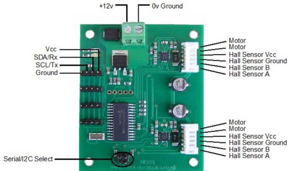
Figura 3.7 Tarjeta MD25
