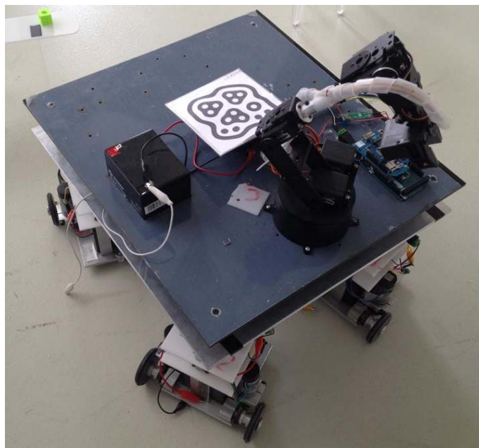
Figura 5.13 Manipulador Móvil Omnidireccional Redundante
