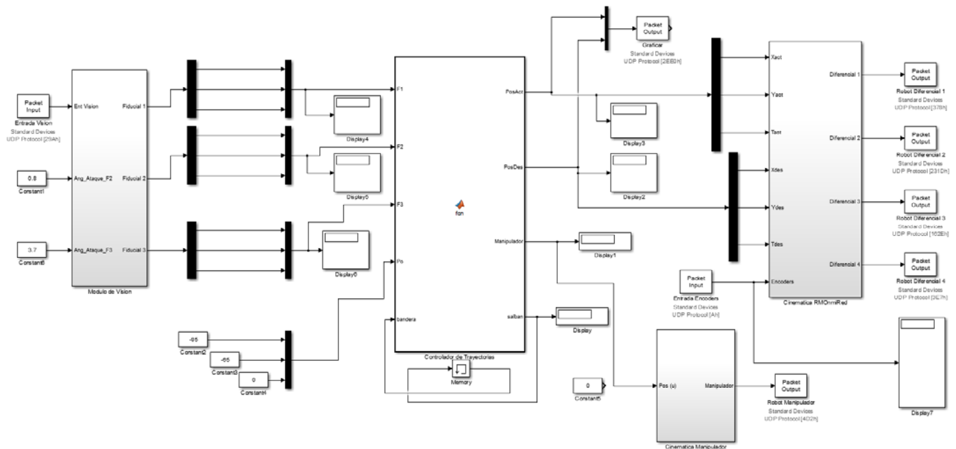
Figura 5.10 Modelo del Sistema de Pruebas en Simulink
