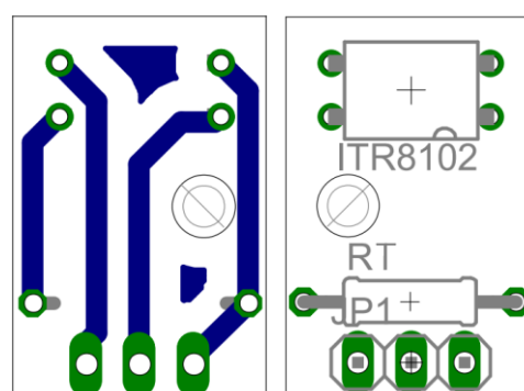
PCB optointerruptor izquierdo
