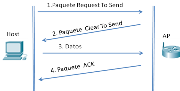
Figura 2.12 Proceso del protocolo CSMA/CA.
