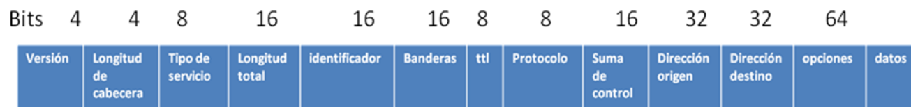
Figura 2.2 Encabezado de paquete IPv4.
