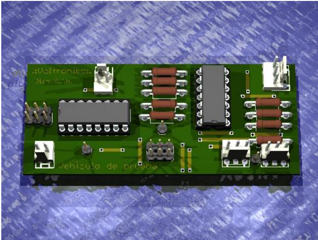
Figura 4.14 PCB principal.
