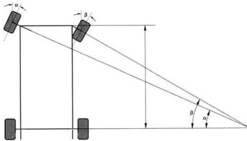
Figura 2.16 Sistema Ackerman.
