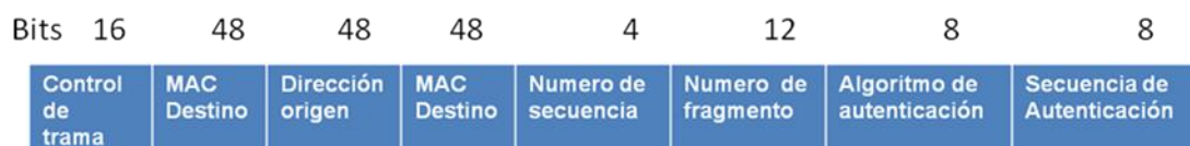
Figura 2.9 Estructura de trama Authentication.
