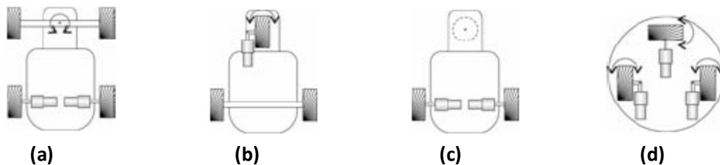
Figura 2.17 Diagrama de diferentes configuraciones de las ruedas en robots móviles.
