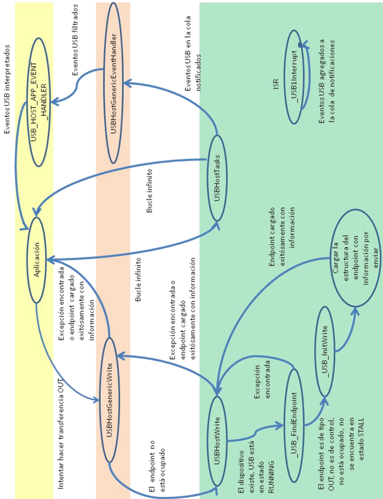
Figura 2.24 Máquina de estados simplificada de un proceso típico de una transferencia OUT con un controlador genérico por eventos.
