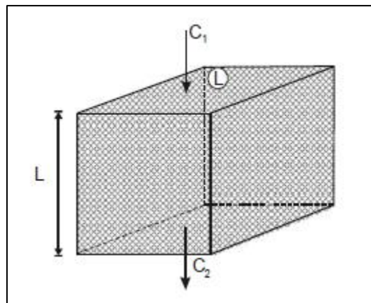
Figura 1.8 Elemento de lecho filtrante (Maldonado, 2004)
