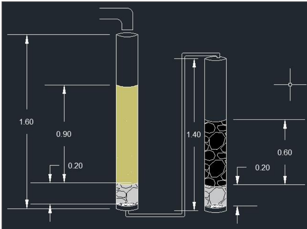
Figura 1.7 Esquema del sistema de filtros de arena (izq.) y carbón activado (der.) descrito en Zipf et al (2016) (Medidas en m) (Elaboración propia, 2019)
