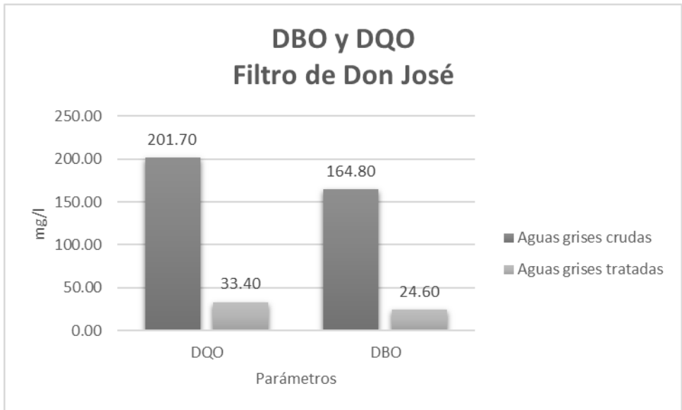
Figura 4.22 Gráfico de los valores paramétricos DBO y DQO de las aguas grises crudas y tratadas del filtro de Don José (Análisis Cántaro Azul, 2019)
