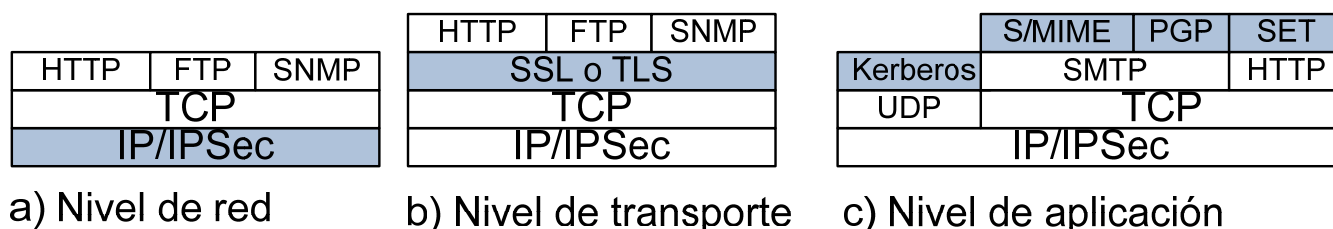
Figura 3. 4 Ubicación relativa de las herramientas de seguridad en la pila de protocolos TCP/IP.
