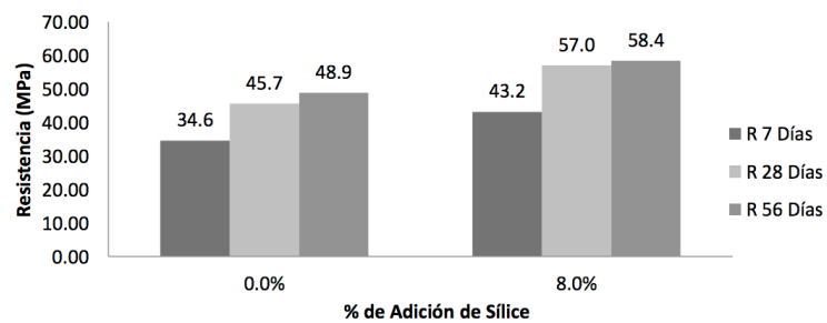
Imagen 14.- Comparativa de resistencia a la compresión en concretos con 0% y 8% de sílice. (O. Barón González, Y. Mercado Quiroz, 2012).
