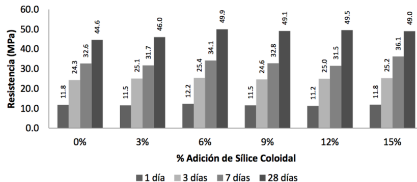
Imagen 15.- Resistencia a compresión en morteros adicionados con sílice (O. Barón González, Y. Mercado Quiroz, 2012).
