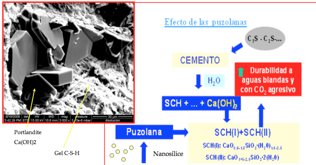
Imagen 4.- Efecto químico: mayor producción de gel CSH. Efecto puzolánico.
