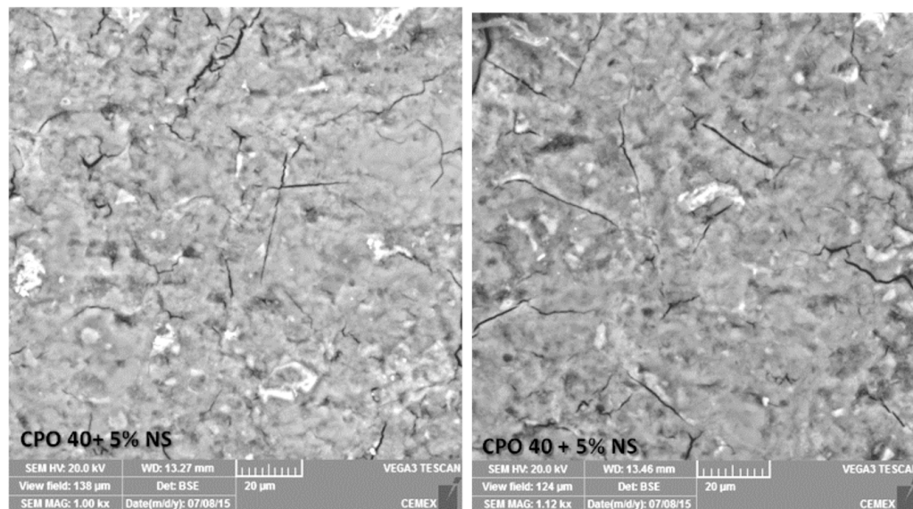
Imagen 12.- Micrografías del cemento CPO con 5% de nanosílice a 1500 y 2500 x a 1300 días de exposición al ataque por sulfatos (C. Enrique Castillo, 2015).
