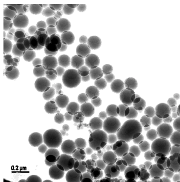
Imagen 8.- Partículas de sílice coloidales amorfas ultra-finas observadas en microscopio electrónico de transmisión (Andri Vital; EMPA Mat'ls Testing and Research, Laboratory for HighPerformance Ceramic, Duebendorf, Switzerland.).
