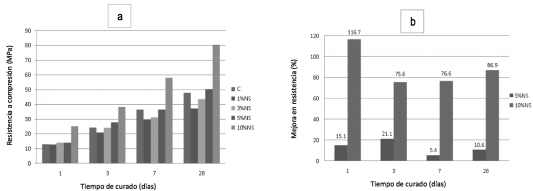
Imagen 13.- Resistencia a compresión de morteros adicionados con nanosílice (a) y porcentaje de mejora en resistencia (b). (Tobon Ji et al., 2011).
