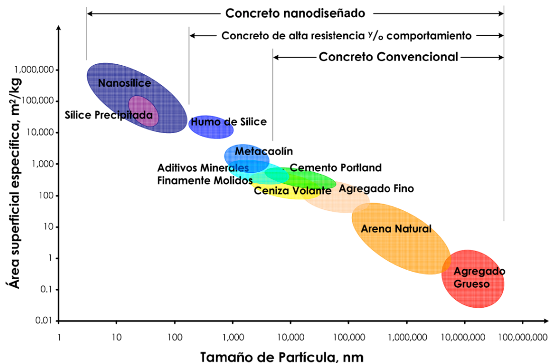
Imagen 2.- Tamaño de partículas y área superficial específica aproximada de los materiales de concreto (K. Sobolev, 2005).
