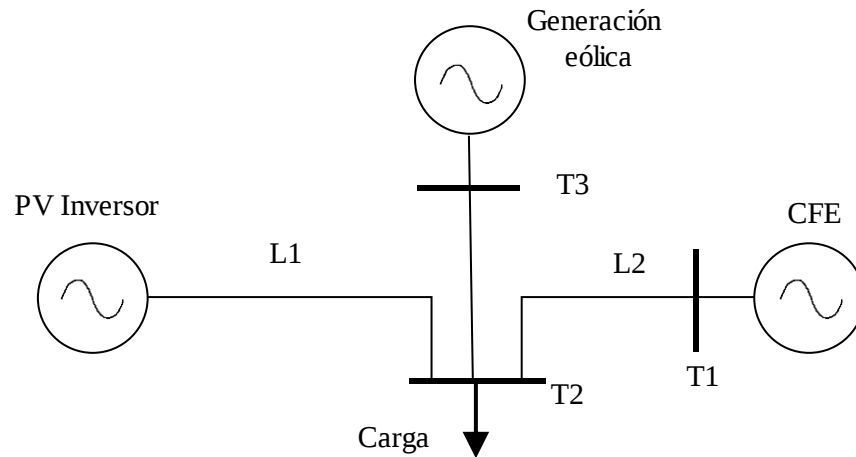
Fig. 4.9. Integración de generación eólica.
