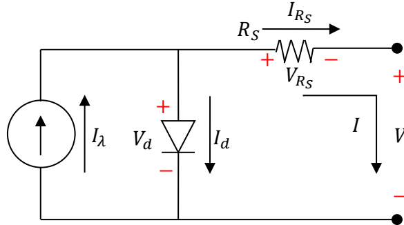
Fig. 2.8. Simplificación de circuito de la celda fotovoltaica con R_{sh} = \infty .
