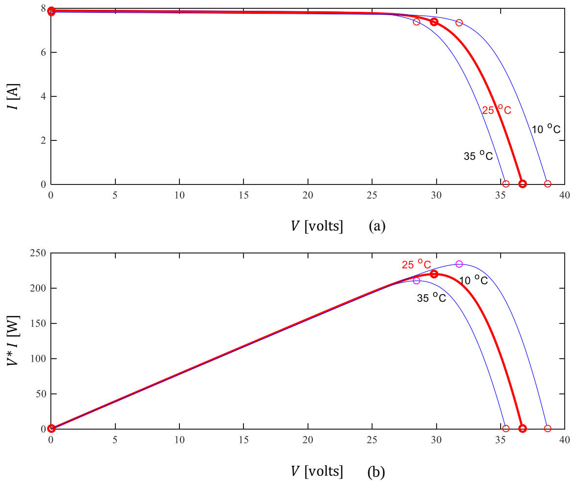
Fig. 2.10. Comportamiento de panel fotovoltaico para corriente (a) y potencia (b), al variar la temperatura en 35, 25 y 10^\circ\text{C} , a irradiancia constante de 1000 \text{ W/m}^2 .
