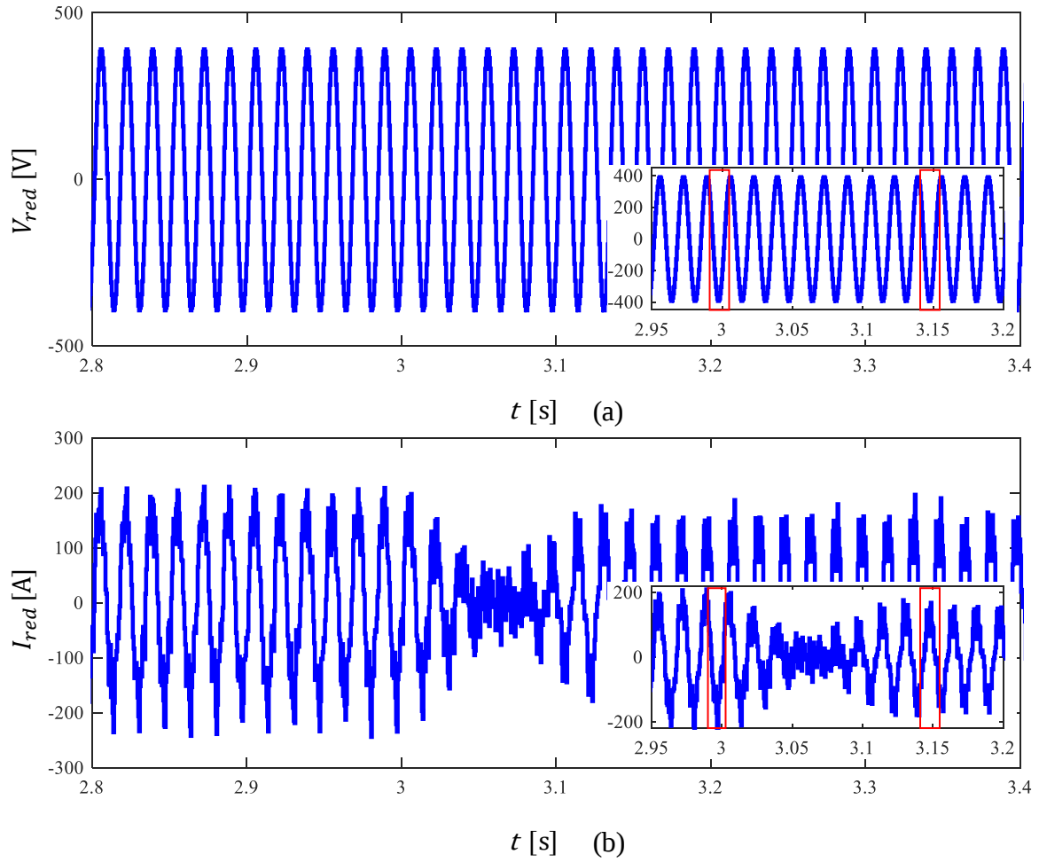
Fig. 4.8. (a) Voltaje trifásico de la Red y (b) Corriente trifásica de la Red.
