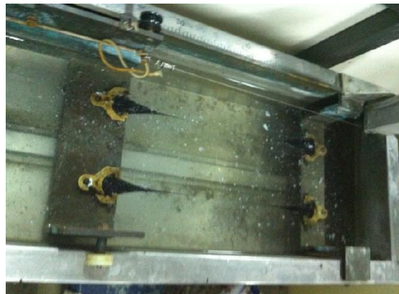
Fig. 2-33 Equipo para ensayo de Ductilidad
