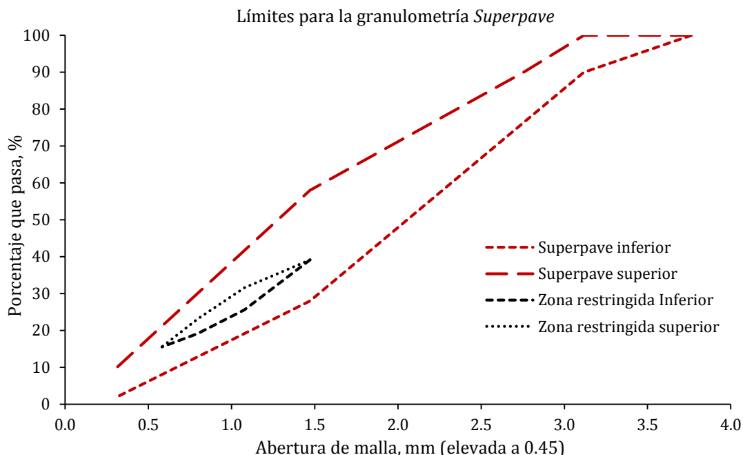
Fig. 4-2 Curvas de control (PC) y zona de restriccion (ZR), metodología SUPERPAVE
