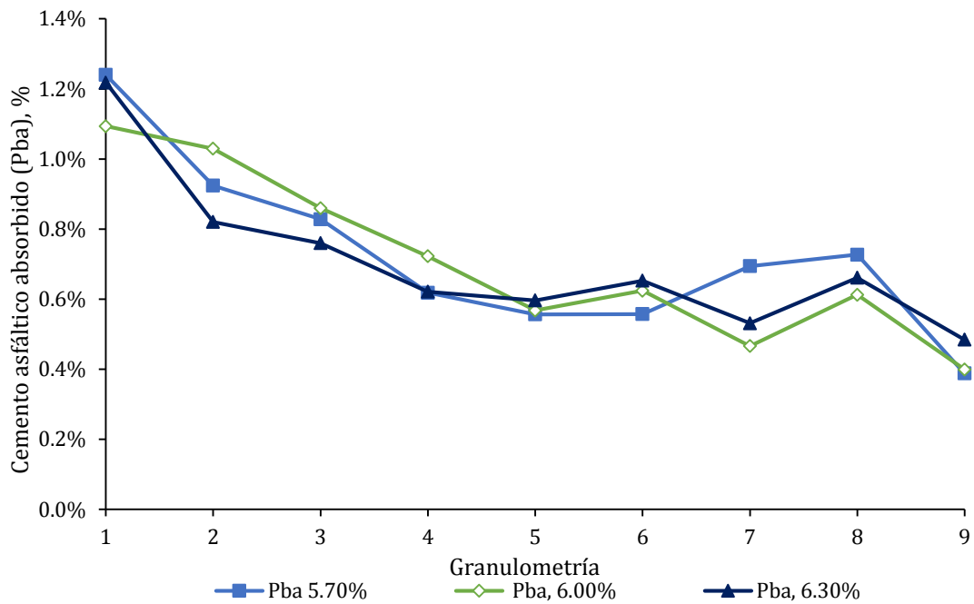
Fig. 4-19 Contenido de cemento asfáltico absorbido ( P_{ba} ) de los concretos asfálticos elaborados con el agregado Tipo 1
