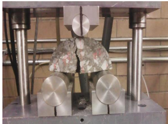
Fig. 4-29 Falla de probeta en ensayo SCB
