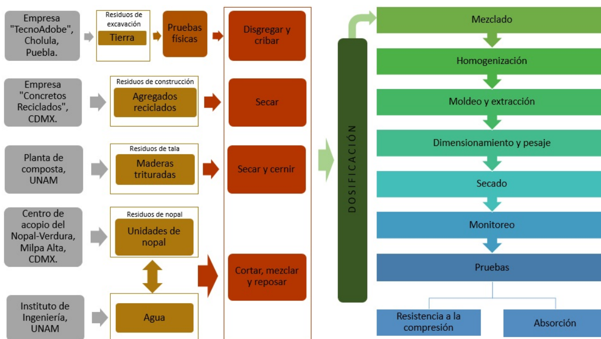
Figura 67. Proceso constructivo
