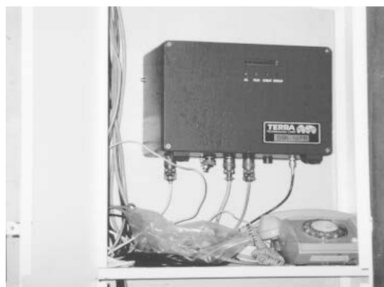
FIGURA 5.1.1. Acelerógrafo tipo usado para el registro de señales de vibración ambiental
