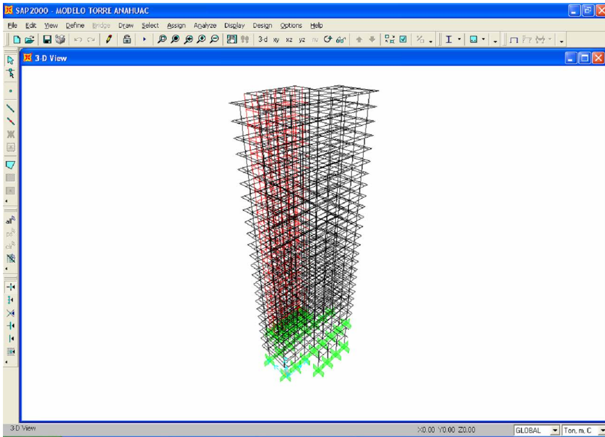
FIGURA 6.2. Modelo realizado en el programa SAP 2000 del edificio ubicado en Reforma N° 52
