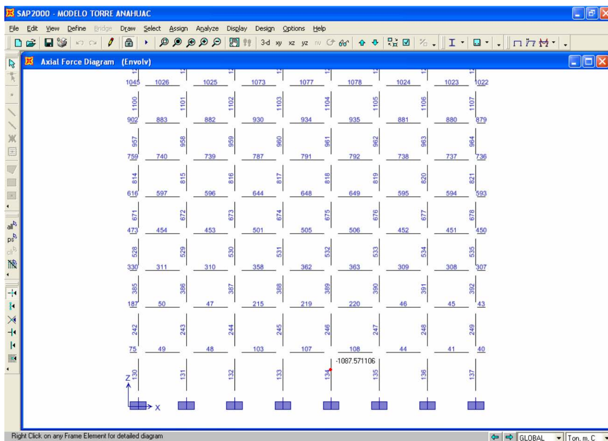
FIGURA 6.8. Elementos Mecánicos. Fuerza Axial del marco I (Envolvente)
