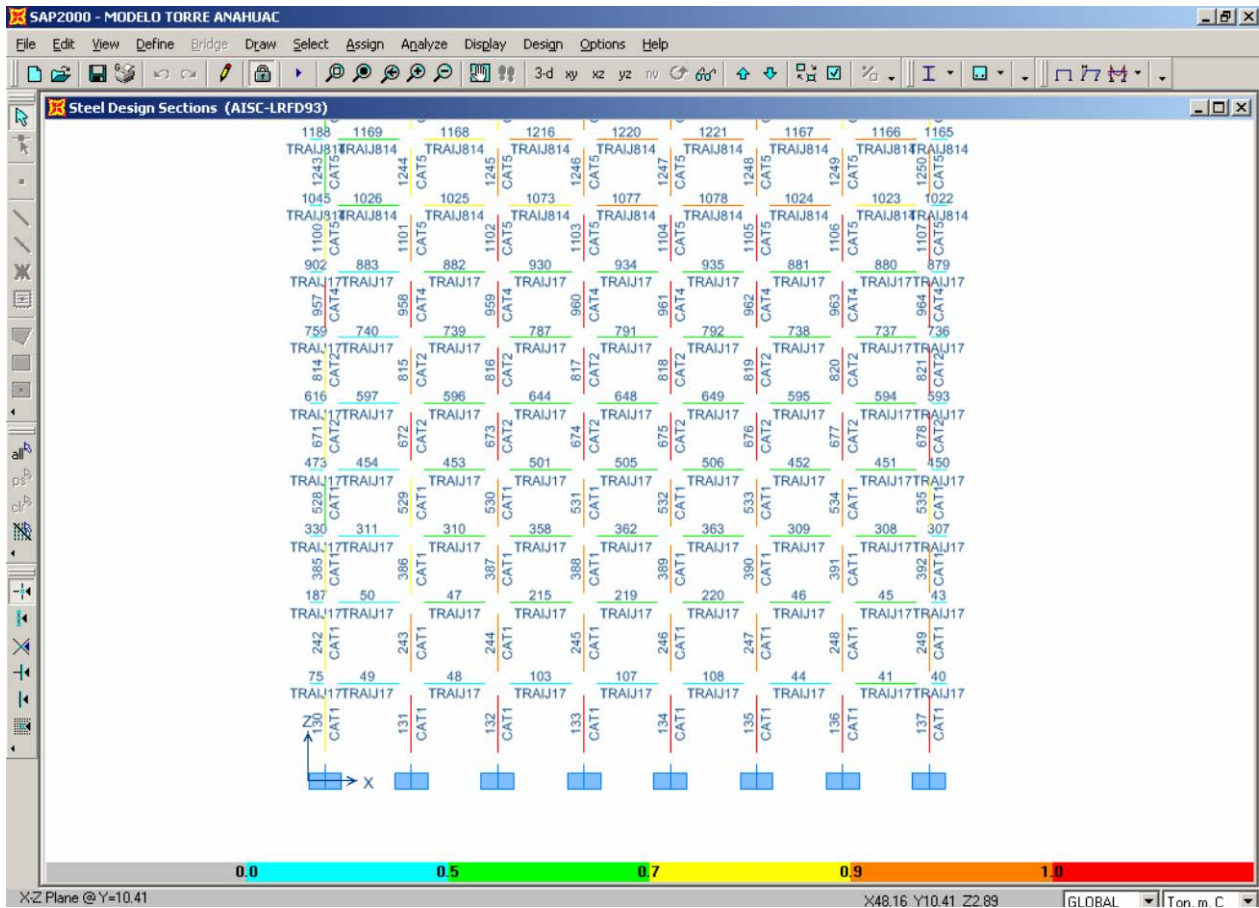
FIGURA 6.16. Nivel de esfuerzos en elementos del marco I parte A según AISC LRDF93
