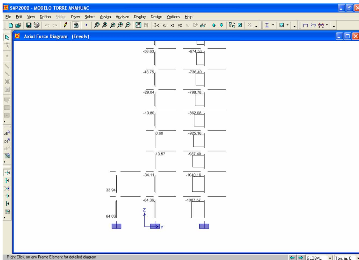
FIGURA 6.9. Elementos Mecánicos. Fuerza Axial del marco 8 (Envolvente)
