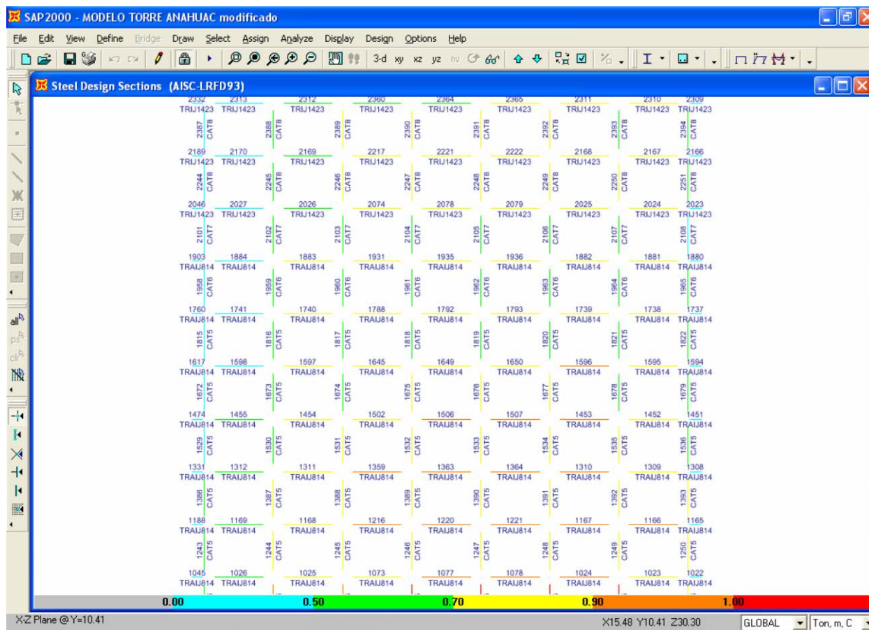
FIGURA 6.29. Nivel de esfuerzos en elementos del marco I parte B modificado según AISC LRDF93
