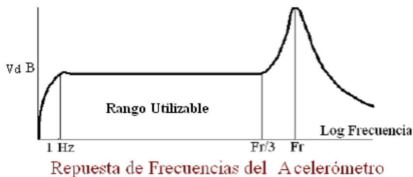
FIGURA 5.1.3. Respuesta de Frecuencias del Acelerómetro
