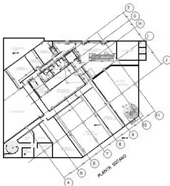
FIGURA 3.1.2. Sótano
