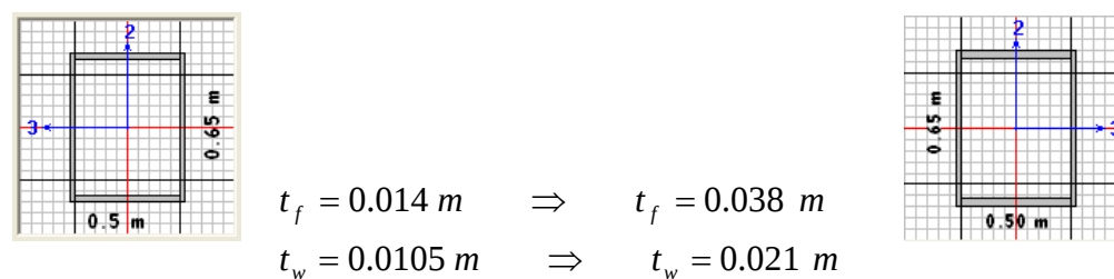
FIGURA 6.27. Reestructuración Columna CAT 6
