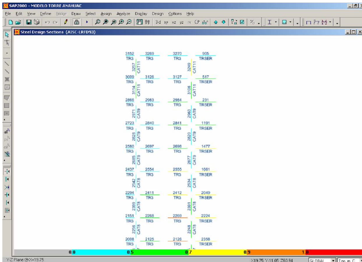
FIGURA 6.21. Nivel de esfuerzos en elementos del marco 8 parte C según AISC LRDF93
