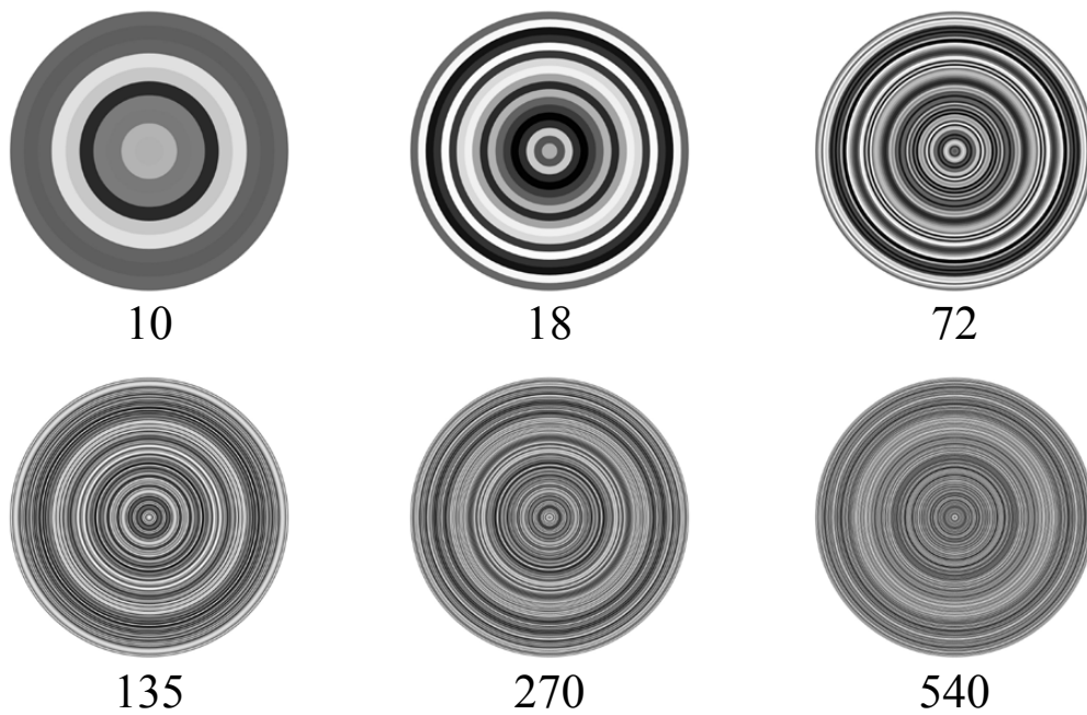
Figura 3.9: Pantallas de fase nula. Lente1 convexo-plana.
