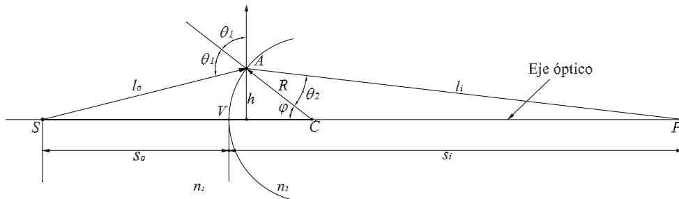
Figura 2.3: Convención de signos.
