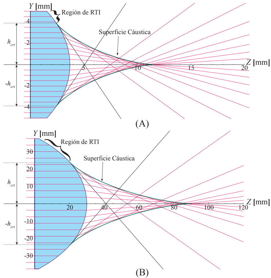
Figura 2.7: Caudísticas de lentes esféricas plano-convexas. (A) Lente 1, (B) Lente 2.
