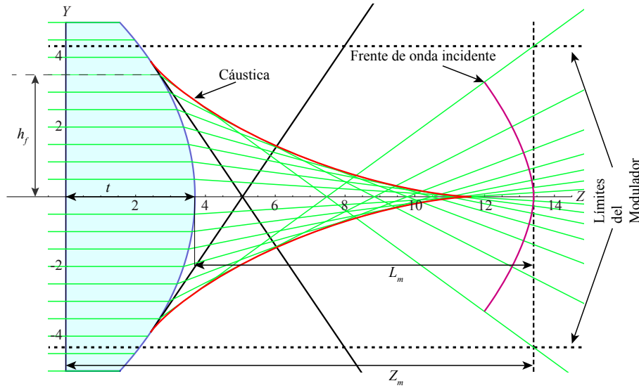
Figura 3.3: Posición del modulador de fase. Configuración plano-convexa.
