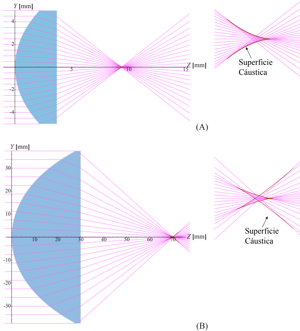
Figura 2.11: Cásticas en configuración convexo-plana.
