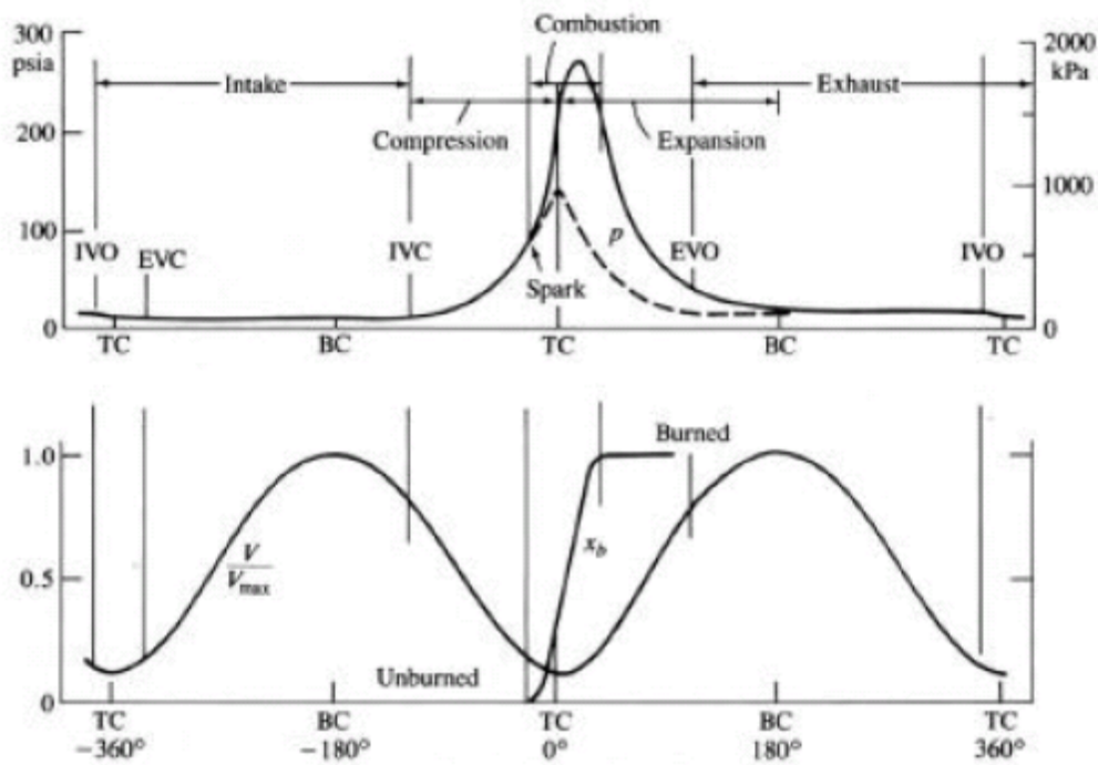
Fig. 2.2 Ciclo de trabajo en MECH.
