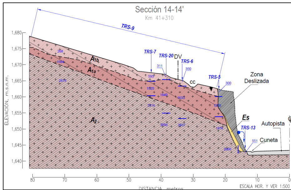
Figura 5.5 Sección geológica 41+310, integrando los datos de la exploración sísmica.
