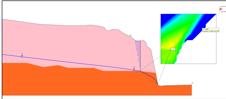
Figura 5.15 Grieta de tensión a 8.0 m del hombro y nivel piezométrico en el contacto
