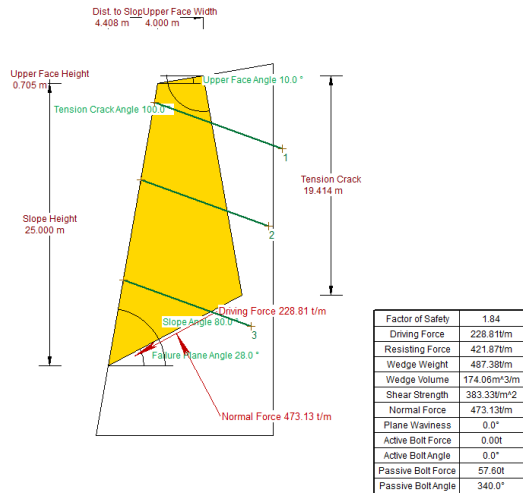
Figura 5.21 CASO 4. Condiciones naturales con anclaje pasivo.
