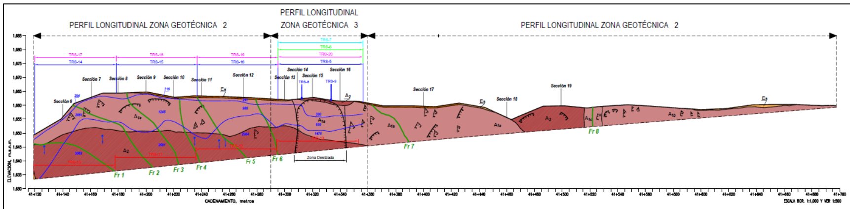
Figura 5.2 Condiciones geológicas de la Zona 2 y Zona 3 compuesta por Andesitas en bloques A 1 y en lajas A 2 .
