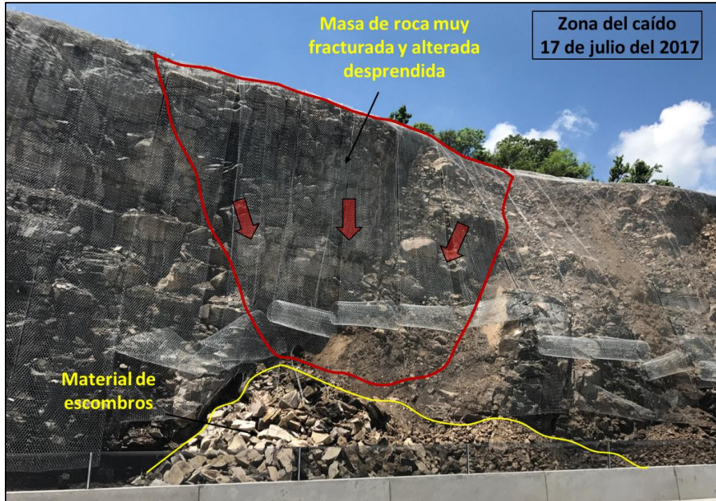
Figura 1.6 Zona del caído km 41+250 previo al deslizamiento de la masa de roca.
