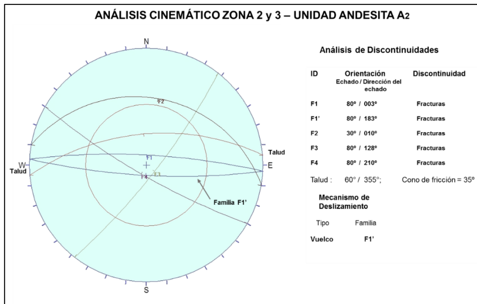
Figura 5.11 Análisis de estabilidad cinemático con el estereograma - Zona 2 Andesita en lajas A 2
