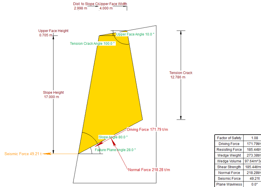
Figura 5.26 CASO 3. Análisis de estabilidad por falla plana ortogonal en bloque (peso propio y sismo), familia F1 y sección transversal crítica.
