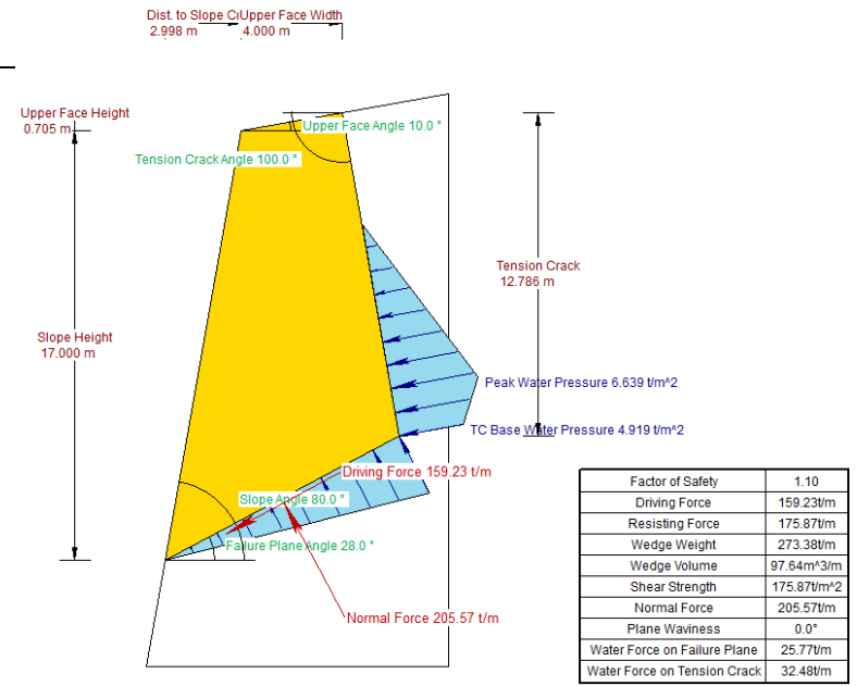
Figura 5.25 CASO 2. Análisis de estabilidad por falla plana ortogonal en bloque (peso propio y presión hidrostática), familia F1 y sección transversal crítica.
