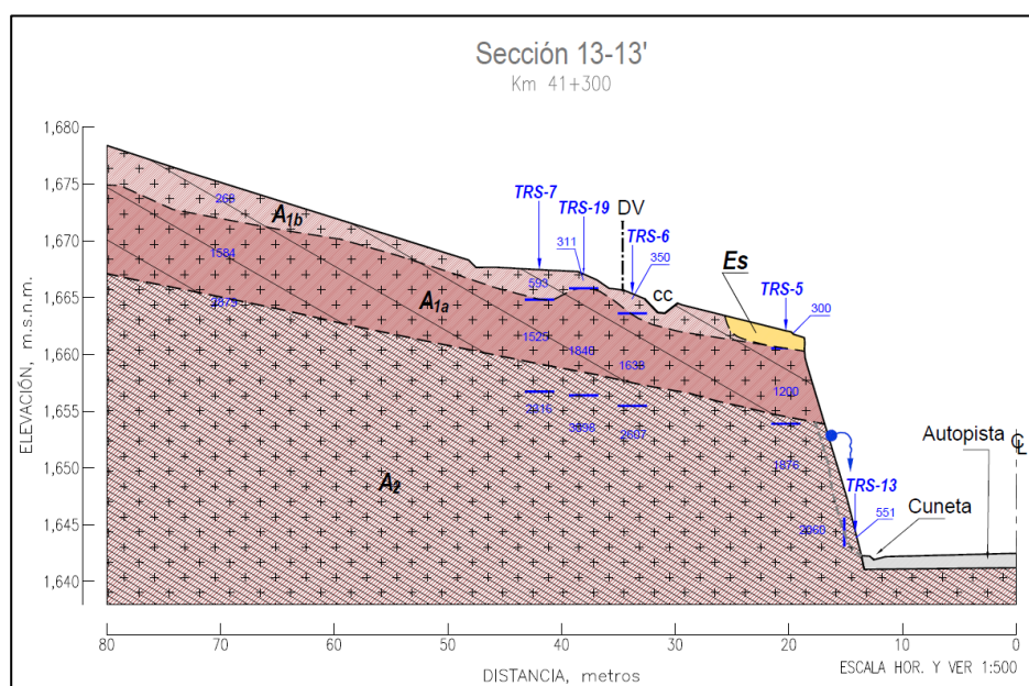
Figura 5.4 Sección geológica 41+300, integrando los datos de la exploración sísmica
