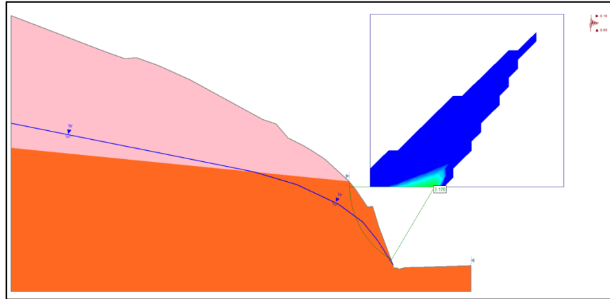
Figura 5.16 Análisis de estabilidad por falla circular en la sección 41+000
