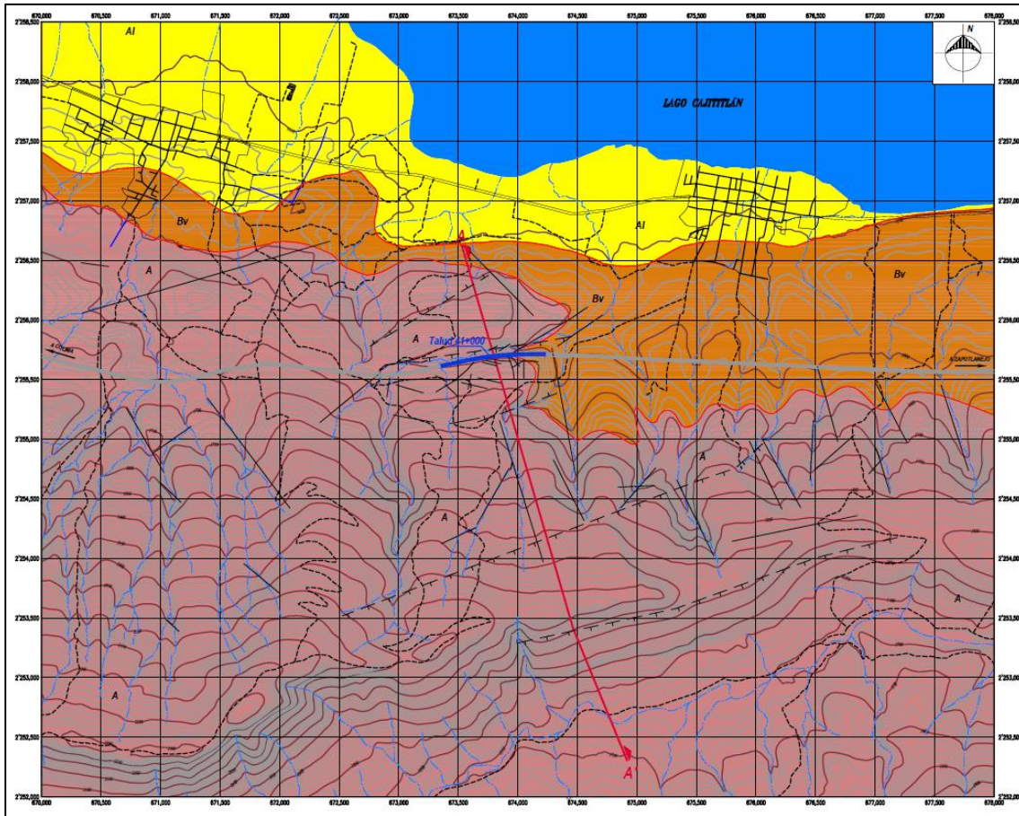
Figura 4.6. Mapa geológico a semidetalle que muestra las fallas geológicas existentes en las inmediaciones del talud 41+000.
