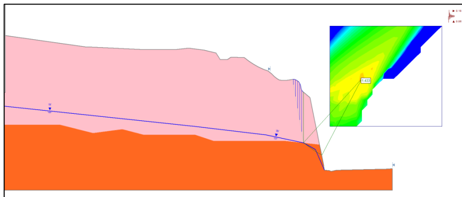
Figura 5.14 Grieta de tensión a 4.0 m del hombro y nivel piezométrico en el contacto
