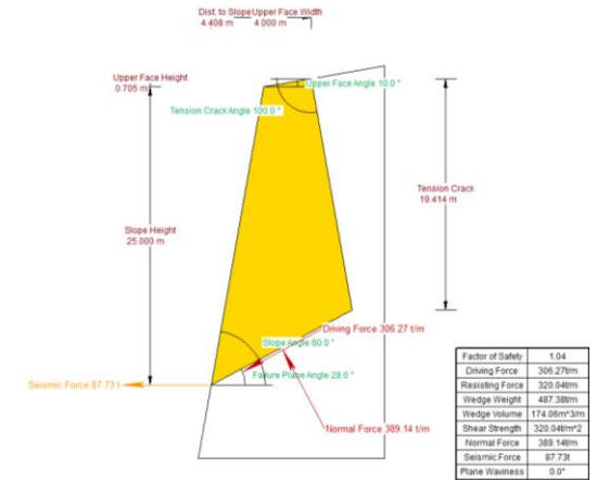
Figura 5.20 CASO 3. Condiciones naturales con sismo Cs=0.18g
