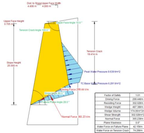
Figura 5.19 CASO 2. Condiciones naturales con agua en grietas al 75%
