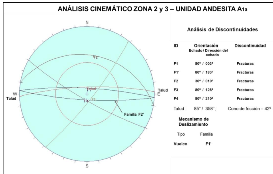
Figura 5.7 Análisis de estabilidad cinemático con el estereograma - Zona 2 Andesita en bloques sana A1a
