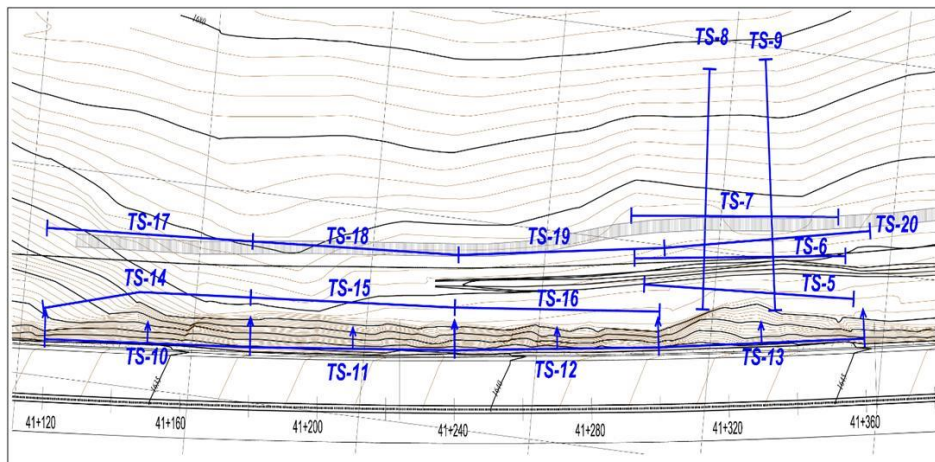
Figura 4.19 Ubicación de Tendidos Sísmicos en el tramo en Andesitas
