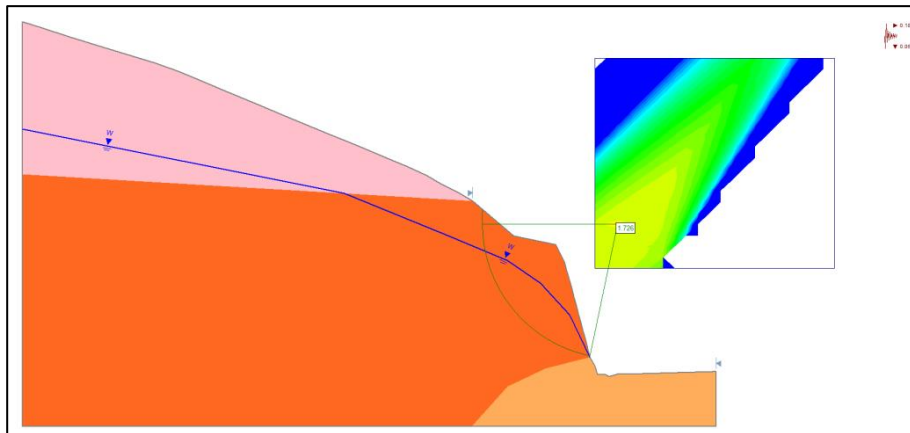
Figura 5.17 Análisis de estabilidad por falla circular en la sección 41+070
