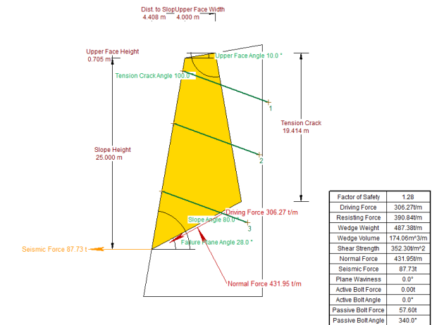
Figura 5.23 CASO 6. Condiciones naturales con anclaje pasivo, y con sismo de Cs=0.18g
