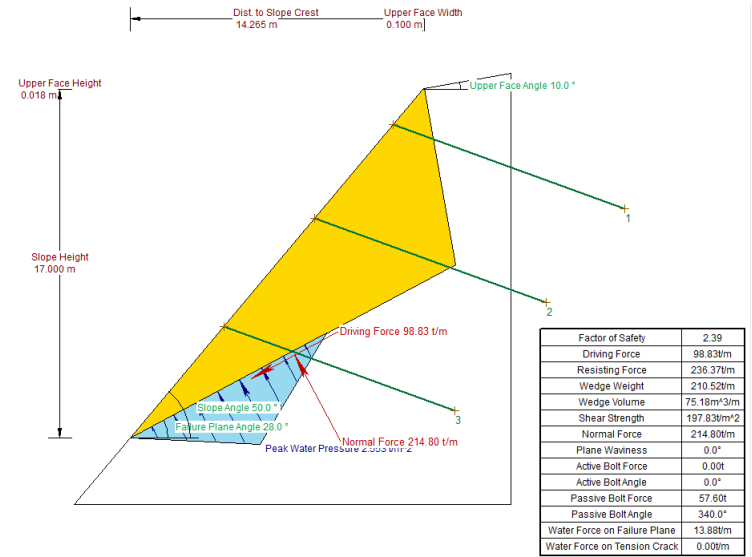
Figura 5.28 CASO 5. Análisis de estabilidad por falla plana ortogonal en bloque (peso propio), familia F1 y sección transversal crítica lado izquierdo considerando el abatimiento del talud de 0.5H : 1.0V (64º aprox.) a 0.70H : 1.0V (55º) y anclaje.
