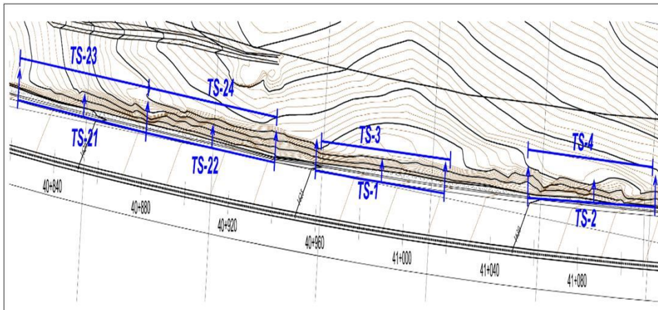
Figura 4.18 Ubicación de Tendidos Sísmicos en el tramo brechas volcánicas
