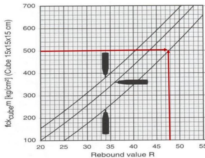
Figura 2.2 Calculo de la resistencia a través del Martillo de Schmidt.
