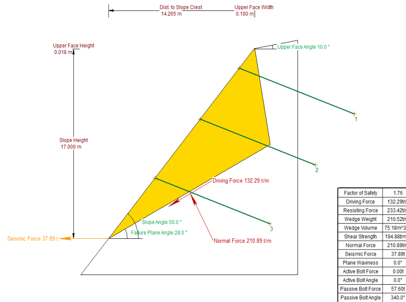
Figura 5.29 CASO 6. Análisis de estabilidad por falla plana ortogonal en bloque (peso propio), familia F1 y sección transversal crítica lado izquierdo considerando el abatimiento del talud de 0.5H : 1.0V (64º aprox.) a 0.70H : 1.0V (55º), drenes de penetración presión hidrostática, sismo y anclaje.
