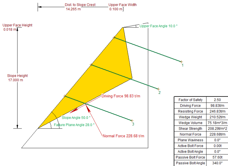
Figura 5.27 CASO 4. Análisis de estabilidad por falla plana ortogonal en bloque (peso propio), familia F1 y sección transversal crítica lado izquierdo considerando el abatimiento del talud de 0.5H : 1.0V (64º aprox.) a 0.70H : 1.0V (55º).
