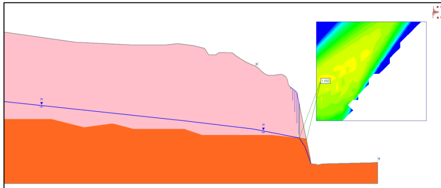
Figura 5.13 Grieta de tensión a 2.0 m del hombro y nivel piezométrico, en el contacto de Andesitas Tm A 1a y Brechas Tm Bv 1 .
