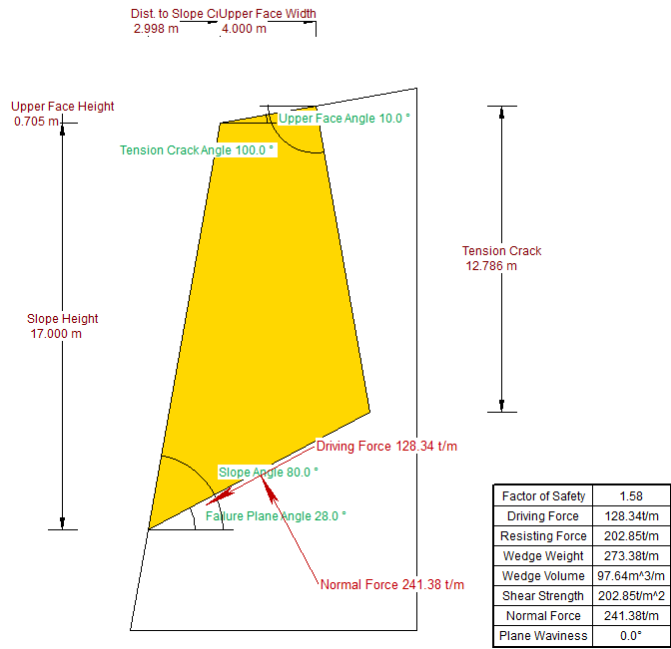
Figura 5.24 CASO 1. Análisis de estabilidad por falla plana ortogonal en bloque (peso propio), familia F1 y sección transversal crítica lado izquierdo.
