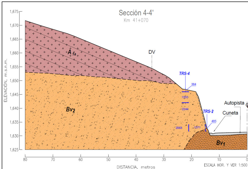
Figura 5.3 Sección geológica 41+070, integrando los datos de la exploración sísmica.
