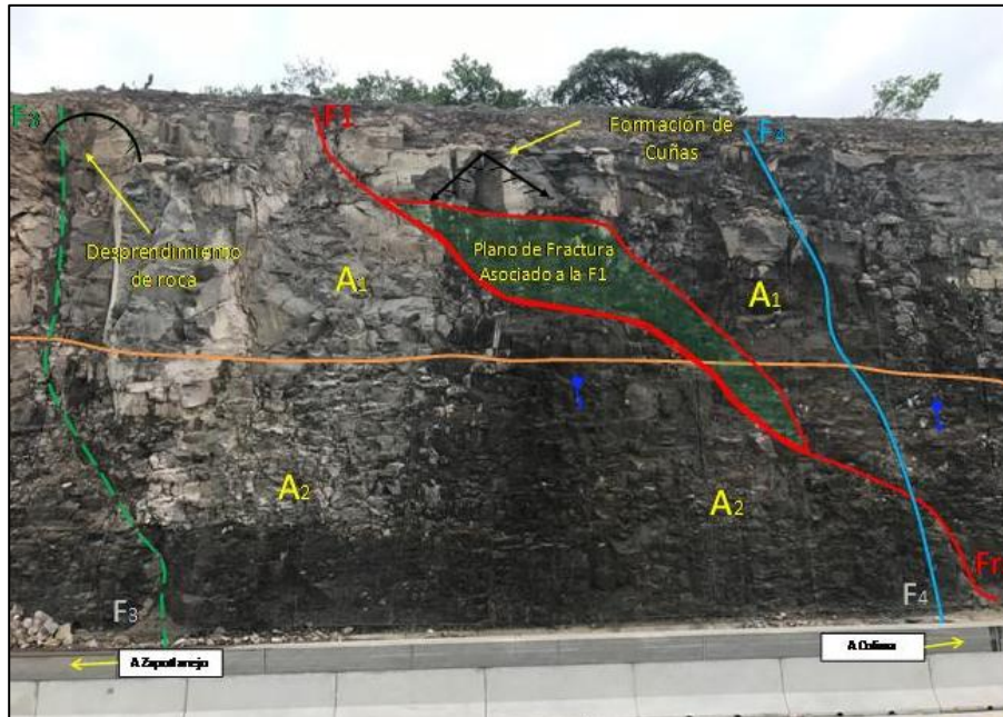
Figura 5.8 Evidencia de salida de bloques por falla plana y vuelco en la unidad Tm A 1a
