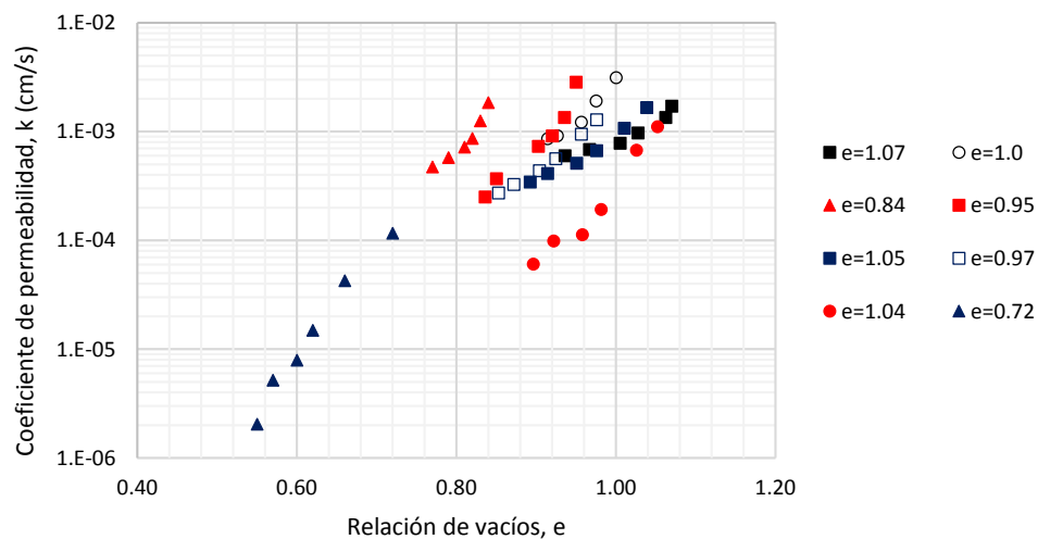
Figura 28. Influencia de la relaci n de vac os en el coeficiente de permeabilidad s lidos (modificado de Acevedo, 2017).
