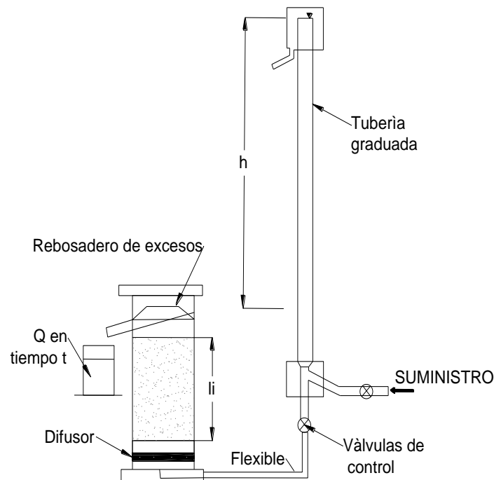
Figura 16. Esquema del permeámetro de carga constante (modificado de Bowles, 1981).
