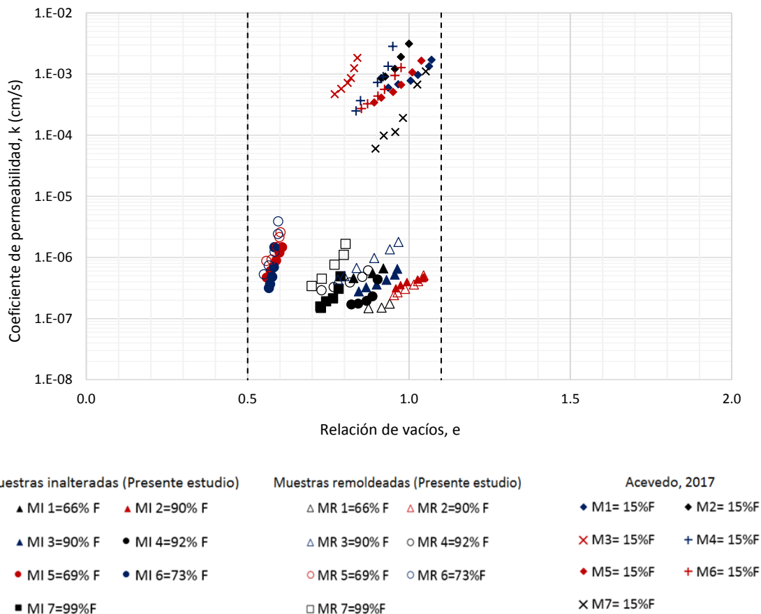
Figura 105. Permeabilidad en función de la relación de vacíos para jales con diferentes contenidos de finos.
