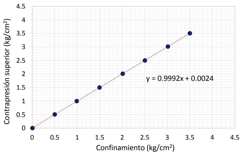
Figura 126. Curva de verificación cruzada confinamiento 2-contrapresión superior 2.
