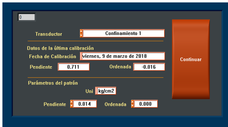
Figura 54. Módulo de calibración.
