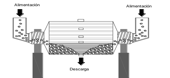
c) Molino con descarga central.
