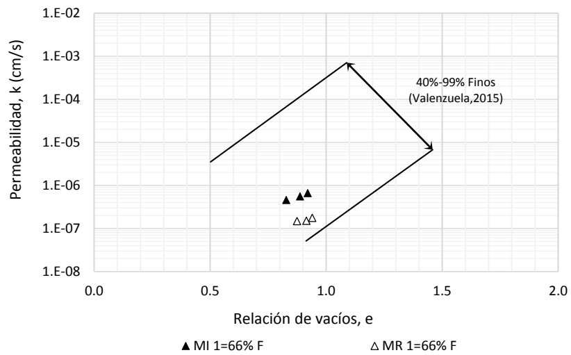
Figura 158. Permeabilidad en función del contenido de finos para ensaye M1
