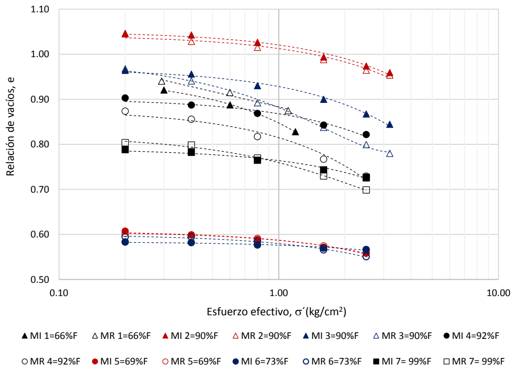
Figura 95. Curva de compresibilidad para las diferentes muestras inalteradas y remodeladas ensayadas.
