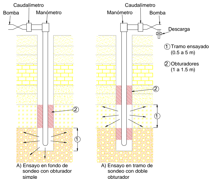
Figura 18. Dispositivo de ensaye de prueba Lugeon.
