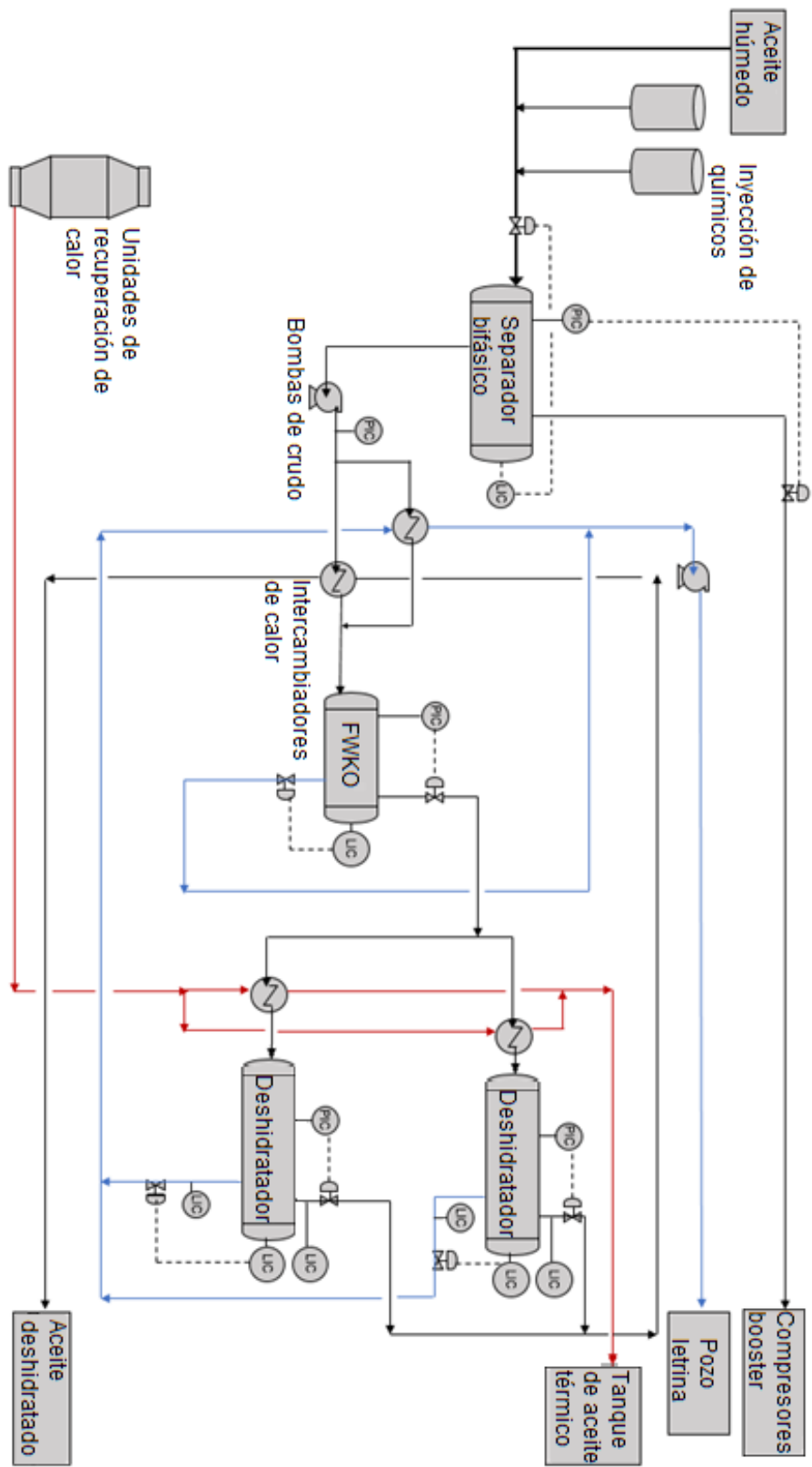
Figura 4.30 Esquema de planta de deshidratación después de su optimización.
