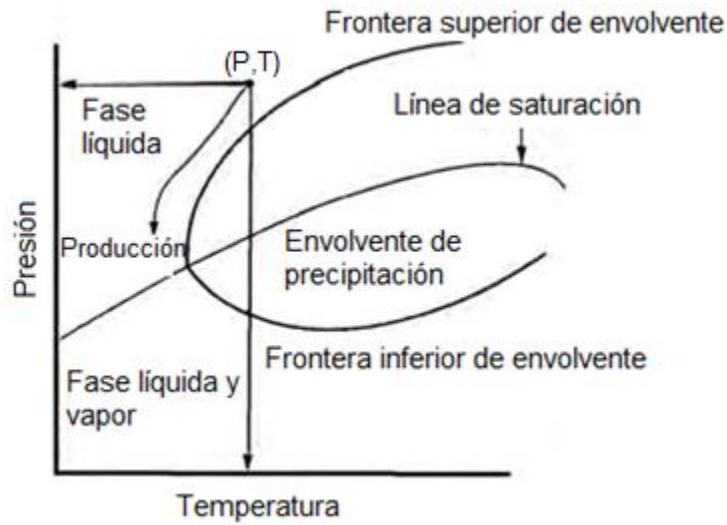
Figura 1.4 Envoltorio de precipitación de asfaltenos (Jasinski, 2007).
