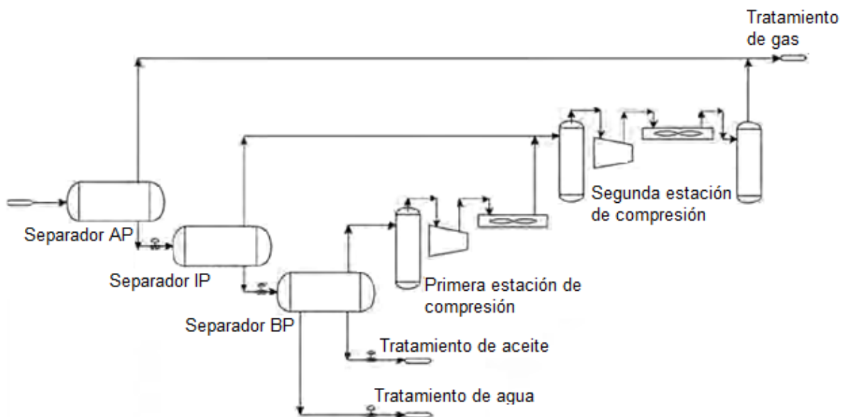
Figura 2.2 Separación con 3 estaciones o etapas (Thro, 2007).
