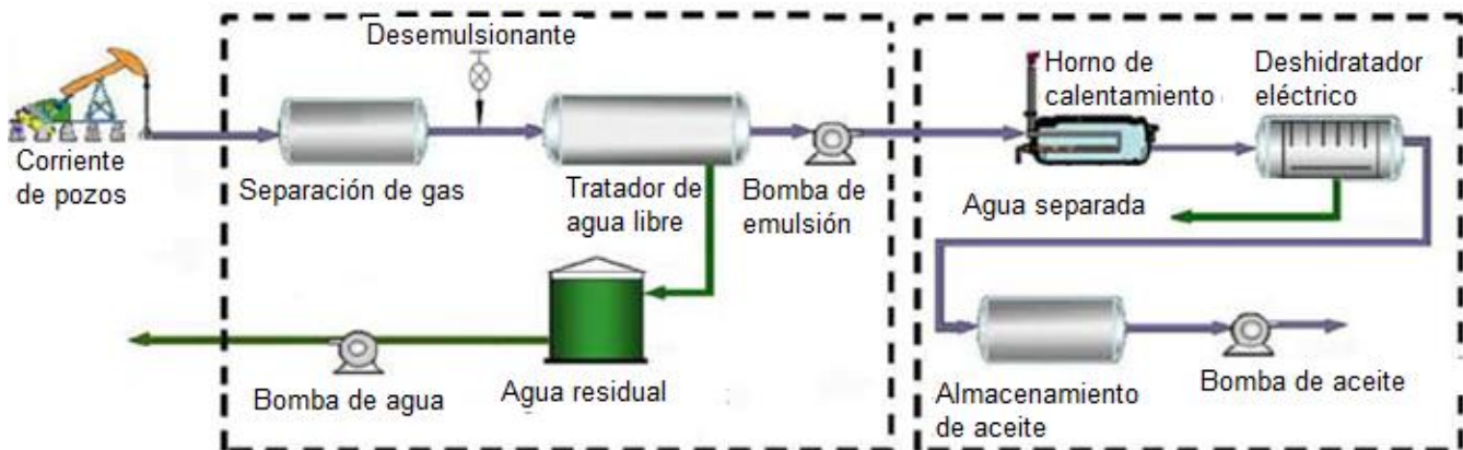
Figura 3.12 Esquema de la optimización del proceso de deshidratación (Wang et al., 2016).
