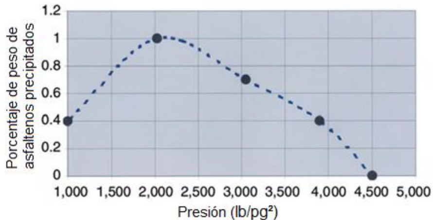
Figura 1.3 Relación de la presión con respecto a la precipitación de asfaltenos (Jasinski, 2007).
