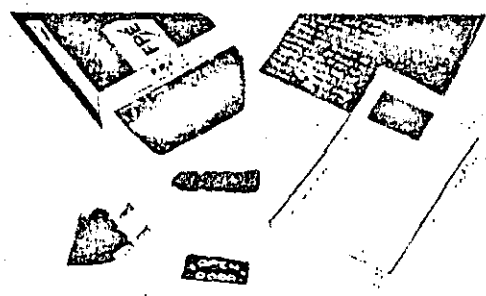
El Juego del entrelace mecánico consiste de un junta, una barra de enclavamiento, un tope, un inmovilizador y una placa de "puerta abierta"
