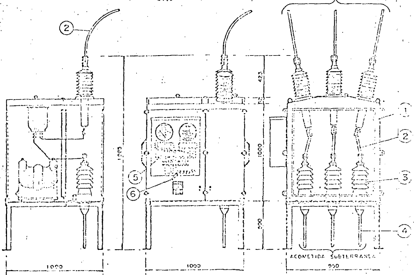
CORTE A-A
