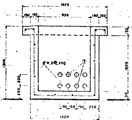
CORTE B-B
