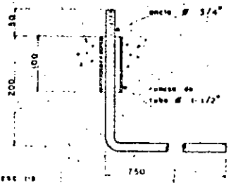
DETALLE DE ANCLAJE
