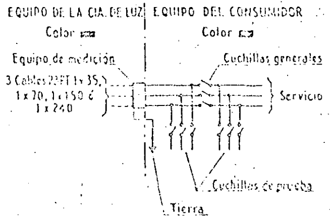
DIAGRAMA TRIFILAR DE CONEXIONES
