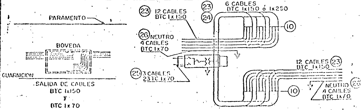
DIAGRAMA UNIFILAR DE LA S.E.
