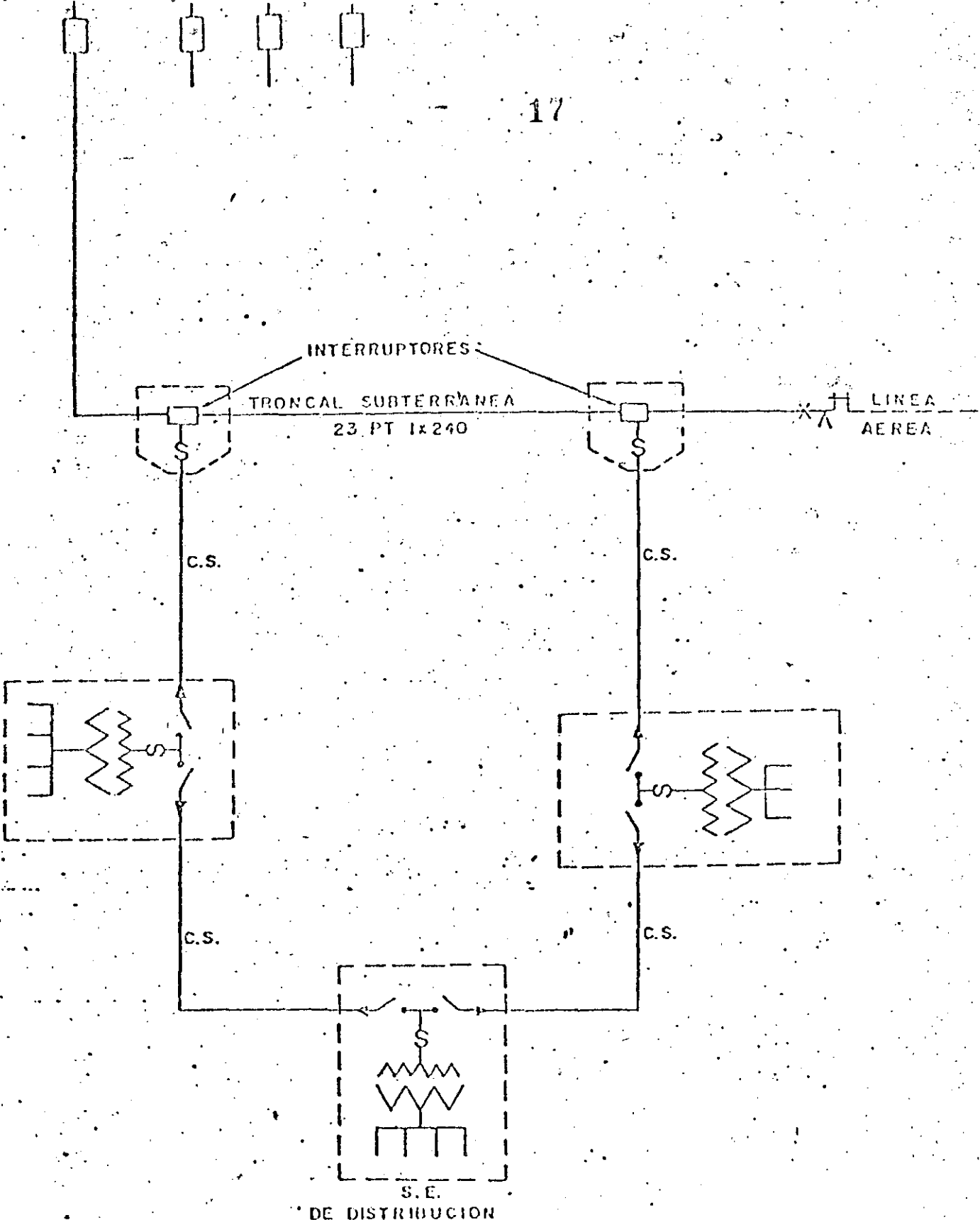
COMPANIA DE LUZ Y FZA DEL CENTRO S.A. EN LIQUIDACION DERIVACION DE UNA TRONCAL SUBTERRANEA PARA UNA ESTRUCTURA EN ANILLO ABIERTO FIGURA No. 6
