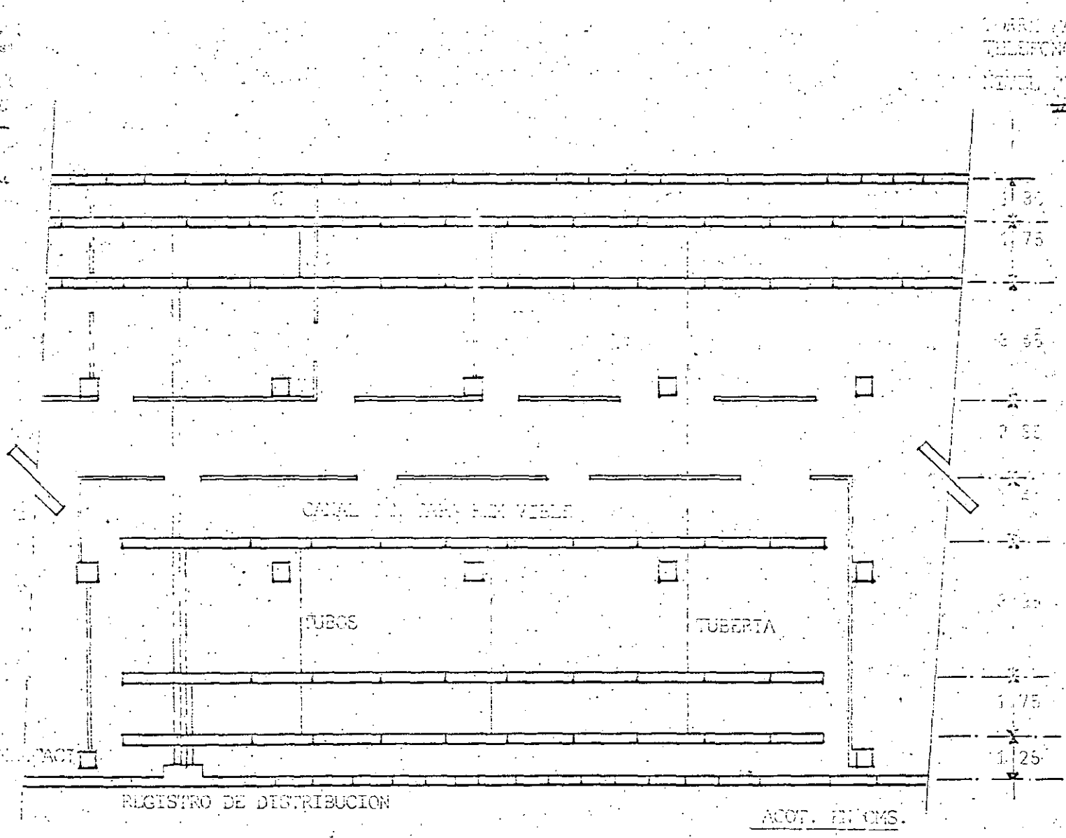
SISTEMAS DE CANALES PARA DISTRIBUCION HORIZONTAL.
