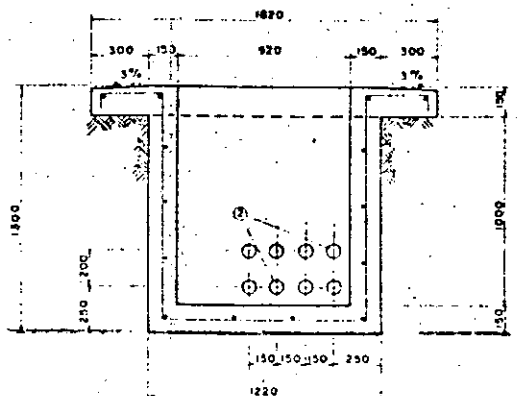
CORTE B-B (PARA CIMENTACION INTEMPERIE)
