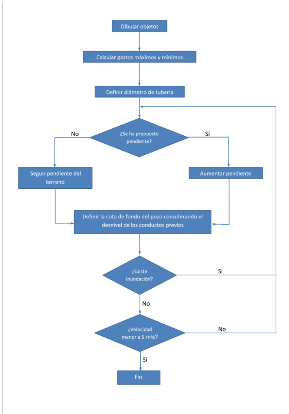
Fig. VI. 7 Metodología de equilibrio de la red de alcantarillado.
