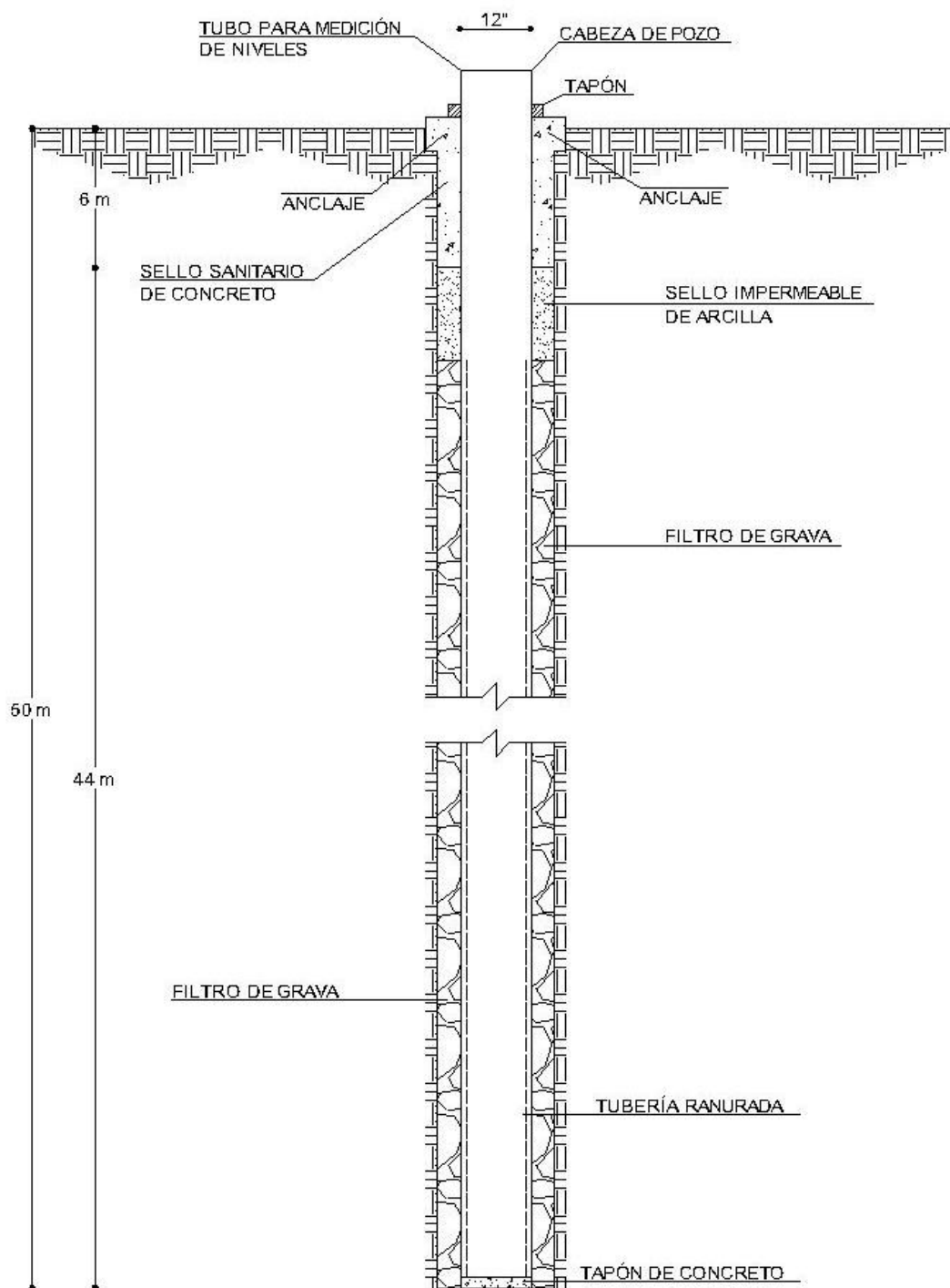
Fig. V. 3 Detalle constructivo del pozo. Elaboración propia
