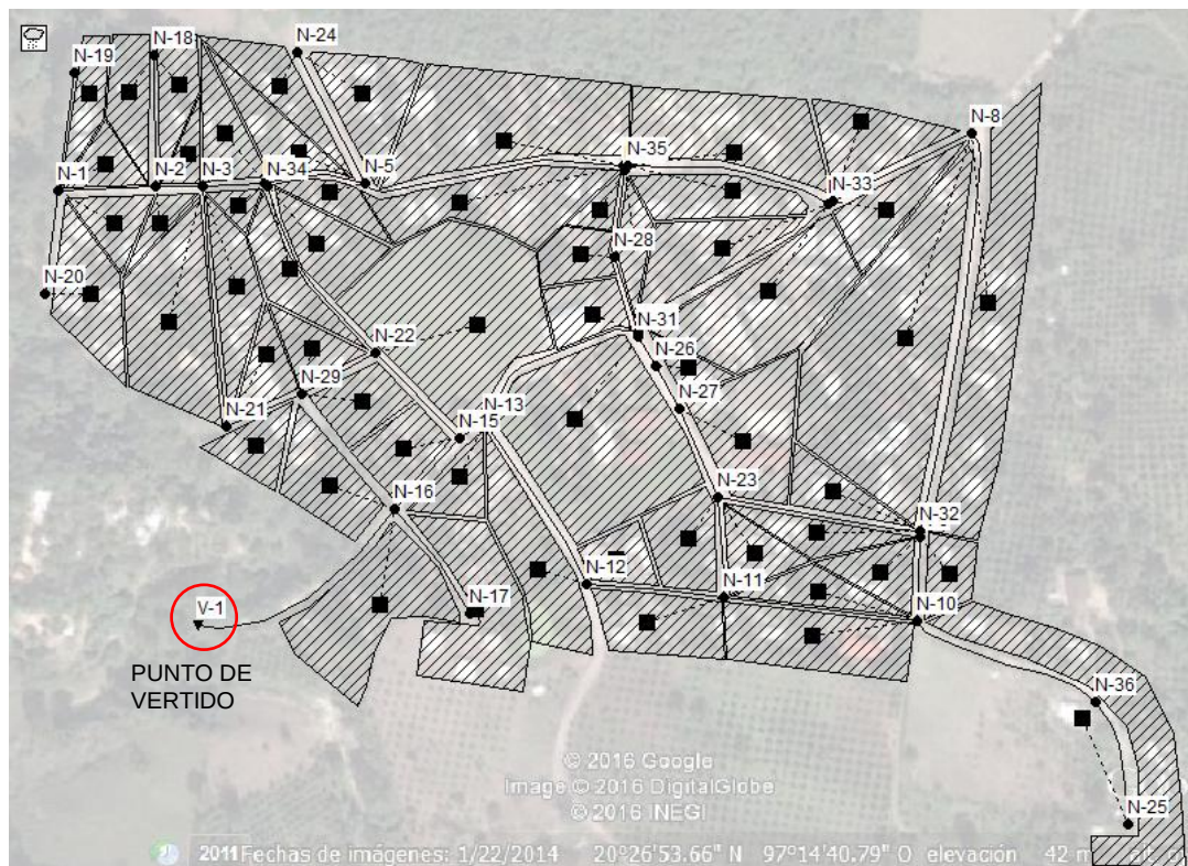
Fig. VI. 2 Ubicación de pozos de visita, punto de vertido y línea de conducción. Fuente: SWMM
