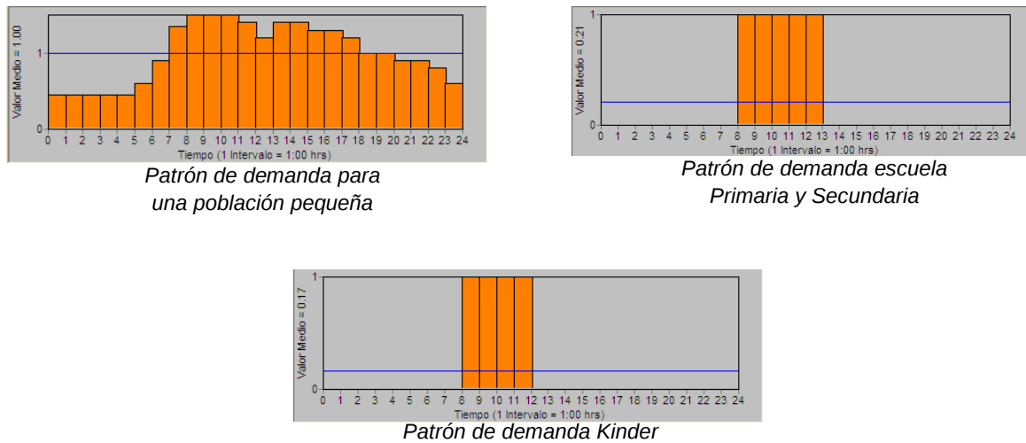
Fig. V. 13 Patrones de demanda. Fuente: EPANET
