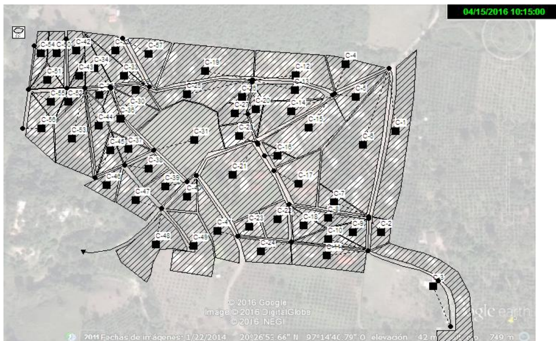
Fig. C- 3 Ubicación y numeración de las cuencas del sistema de alcantarillado
