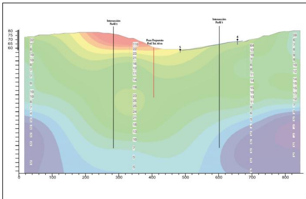
Fig. V. 1 Ubicación y profundidad del pozo profundo sobre la sección geoelectrica 4. Elaborada por la DICT, UNAM
