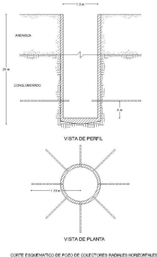
Fig. V. 4 Esquema constructivo de pozo con drenes radiales horizontales. Elaboración propia
