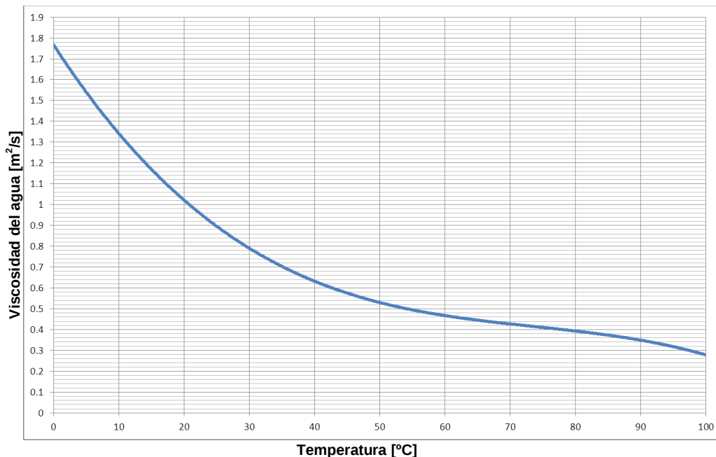
Fig. V. 9 Variación de la viscosidad cinemática del agua con la temperatura. Fuente: CONAGUA
