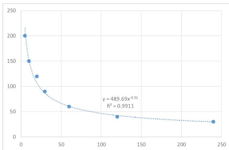
Fig. VI. 4 Curva Intensidad – duración. Elaboración propia utilizando datos de SCT (Anexo D)
