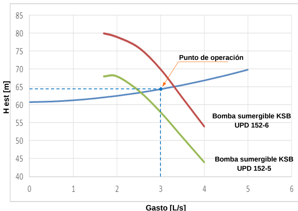
Fig. V. 5 Curva característica del sistema. Elaboración propia
