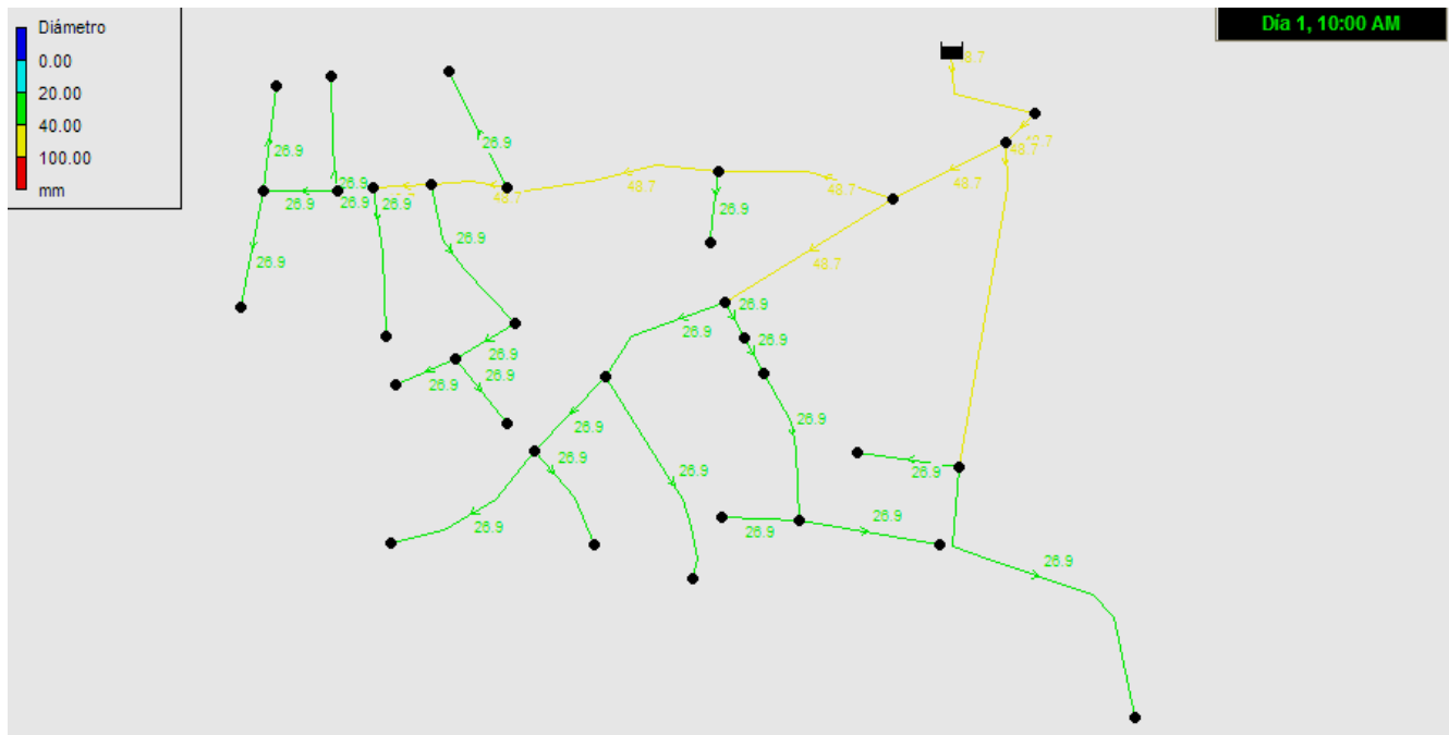
Fig. V. 15 Diámetros de tuberías al equilibrar a red. Fuente: EPANET
