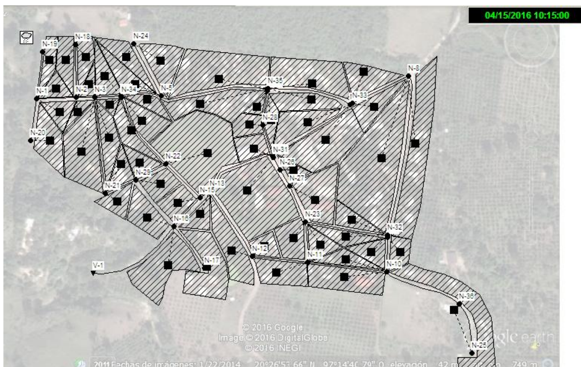
Fig. C- 4 Ubicación y numeración de los nodos del sistema de alcantarillado
