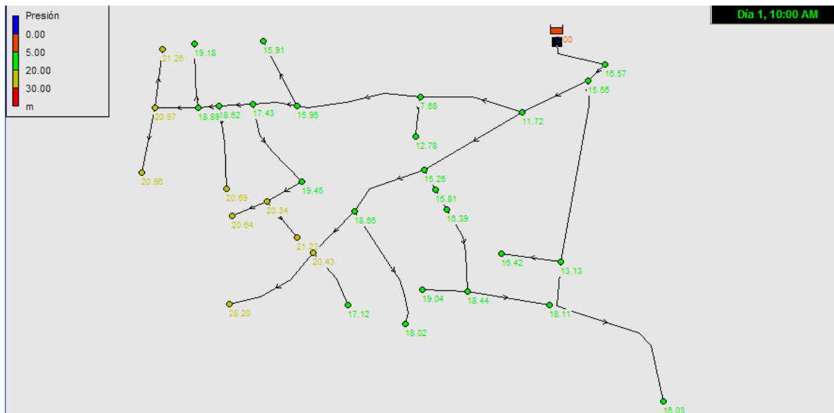
Fig. V. 14 Presiones en m.c.a para cada nodo. Fuente: EPANET
