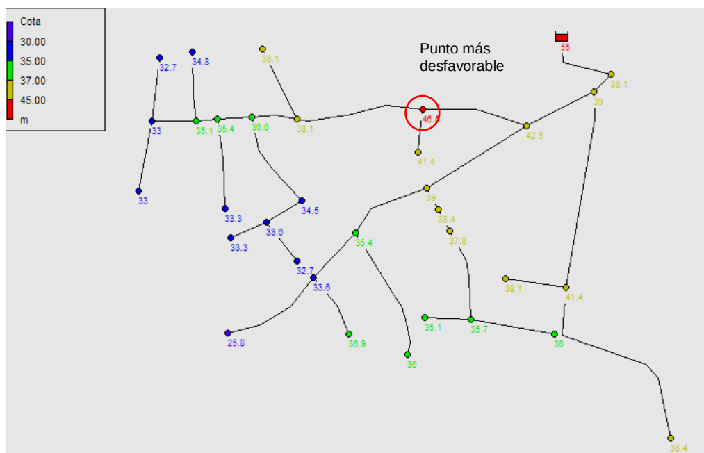
Fig. V. 12 Cotas de los nodos y ubicación del punto más desfavorable. Fuente: EPANET
