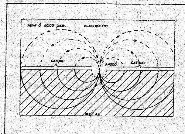
Fig. 23 Flujo de Corriente en un agujero corroído.
