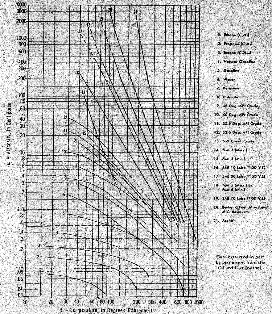
Graf. 1 VISCOSIDAD DEL AGUA Y PRODUCTOS LIQUIDOS DEL PETROLEO
