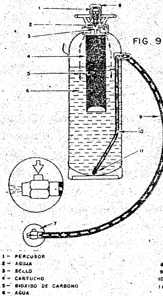
EXTINGUIDOR DE AGUA 9.5 L (2 1/2 GAL) DE CAPACIDAD CON CARTUJO A PRESION
