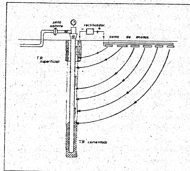
Instalacion Típica de Protección Catódica para una Tubería de - Revestimiento.
