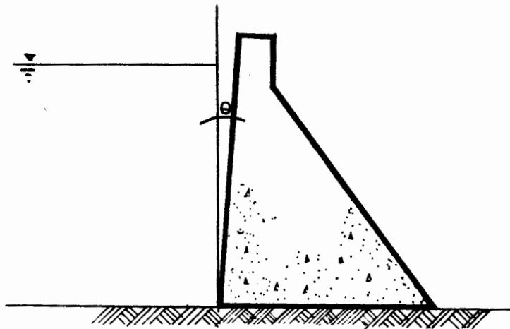
Fig. III.21 Angulo del paramento aguas arriba para cálculo de C_m .
