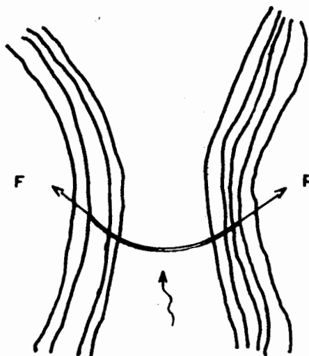
Fig. V.1 Transmisión de las cargas hacia los atraques en una presa de arco.
