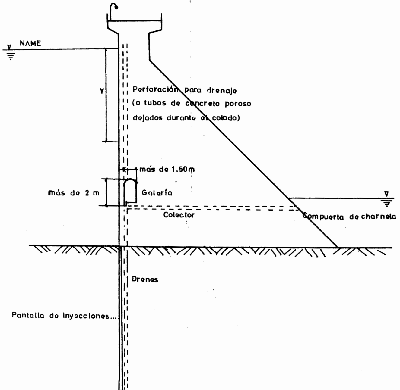
Fig. III.12 Detalles de un sistema de drenaje en una presa de gravedad.
