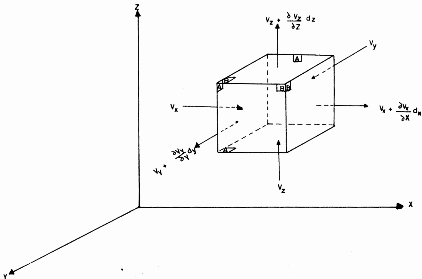
Fig II.30 Región sujeta a flujo tridimensional.
