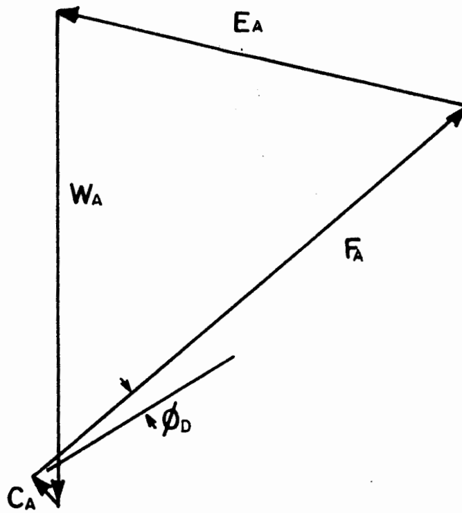
Fig II.52 Diagrama vectorial de la cuña activa.
