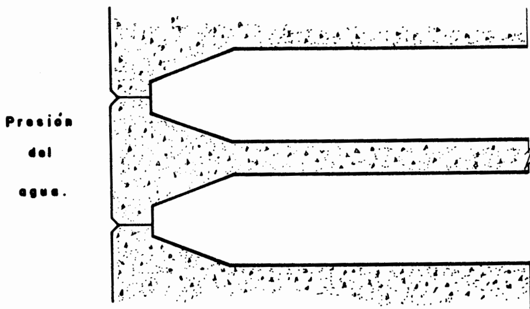
Fig. IV.15 Machones con cabeza en T
