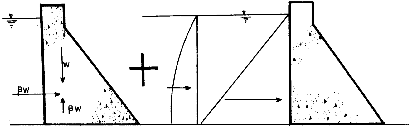
Fig III.18 Combinación de cargas producidas por sismo.
