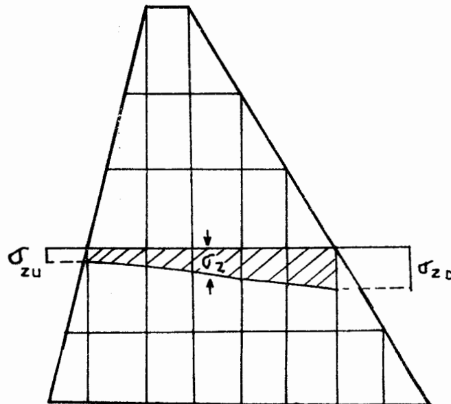
Fig. III.30 Esfuerzos normales en un plano horizontal.
