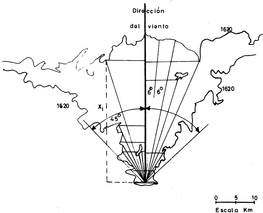
Fig II.25 Cálculo del fetch efectivo
