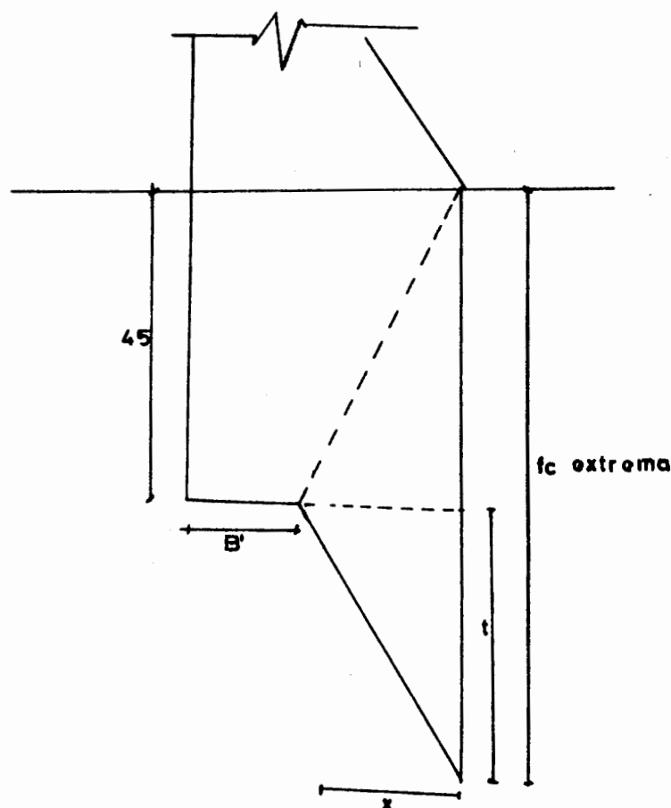
Fig. III.28 Diagrama de esfuerzos efectivos.
