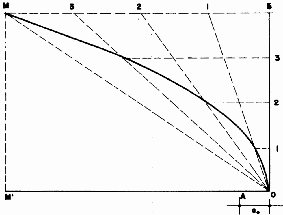
Fig II.37 Método para el trazo de la parábola básica de Kozeny (o de cualquier parábola).
