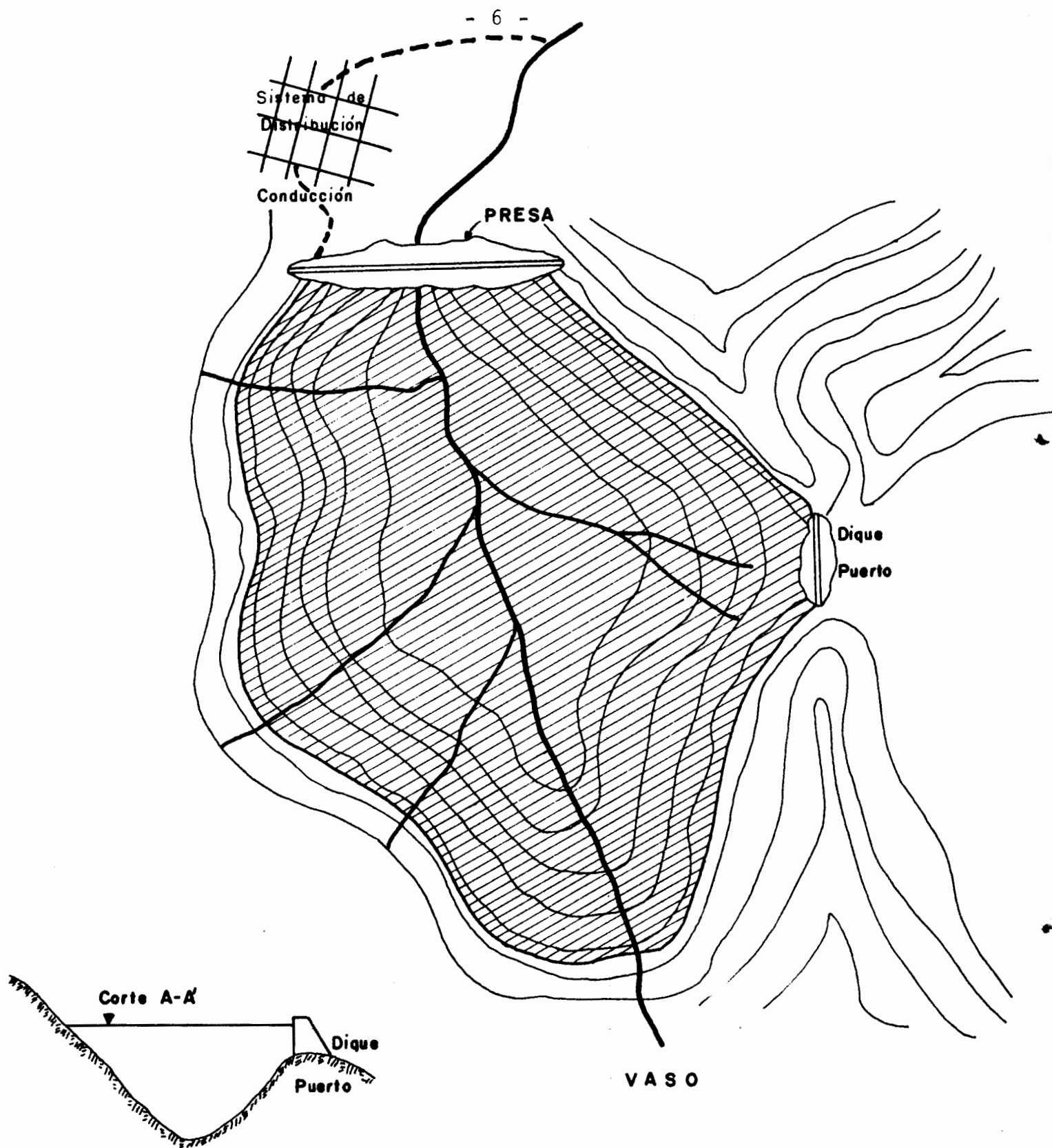
Fig I.I Elementos de un aprovechamiento hidráulico superficial y algunas estructuras de presas.
