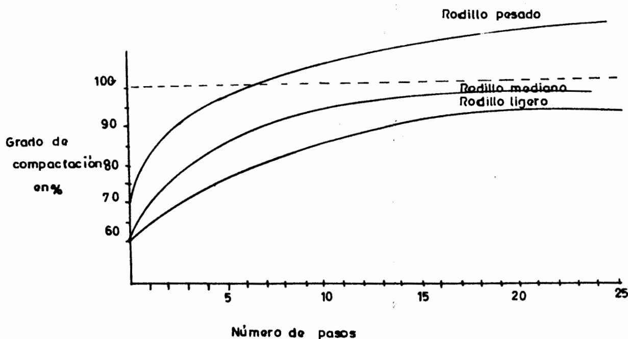
Fig II.41 Efecto del n\u00famero de pasadas de rodillo sobre el grado de compactaci\u00f3n.
