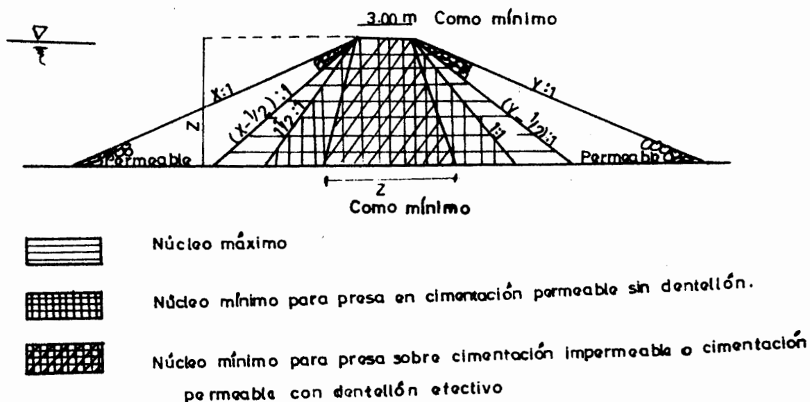
Fig II.11 Variación de tamaños de los núcleos impermeables en los terraplenes con puestos. U.S.B.R. (3)
