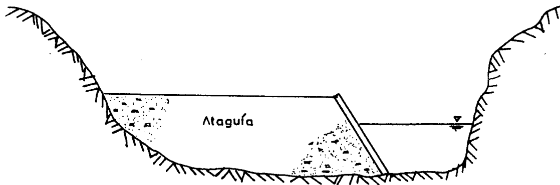
Fig II.55 Obra de desvío en tajo.
