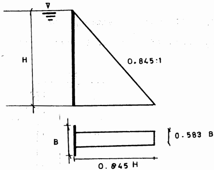
Fig. IV.4 Grueso de un contrafuerte, suprimida la subpresión.
