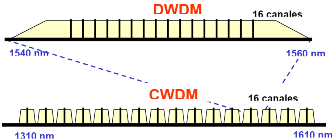
Figura 1.4.- Ejemplo de una distribución de canales en DWDM y CWDM
