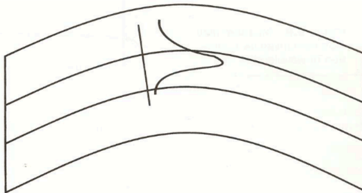
Figura 2.1.- Debido a la gran curvatura de la fibra, parte de la potencia de la señal sale del núcleo.
