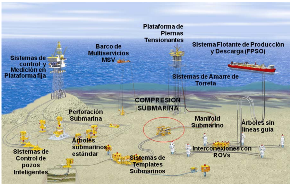
FIG. II.41 Ubicación del compresor submarino Propiedad CAMERON
