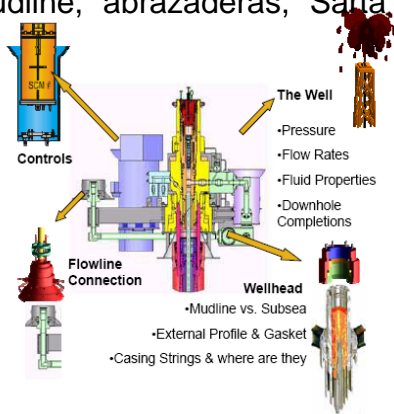
FIG. II.6 Consideraciones para el diseño de un árbol submarino Propiedad CAMERON
