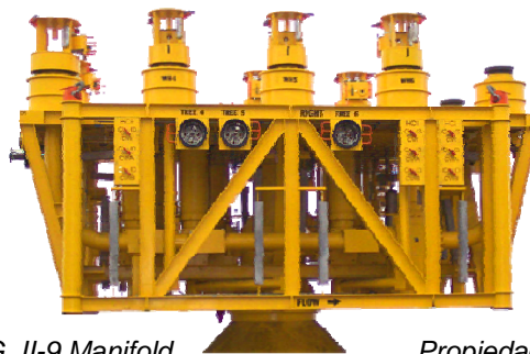
FIG. II-9 Manifold
