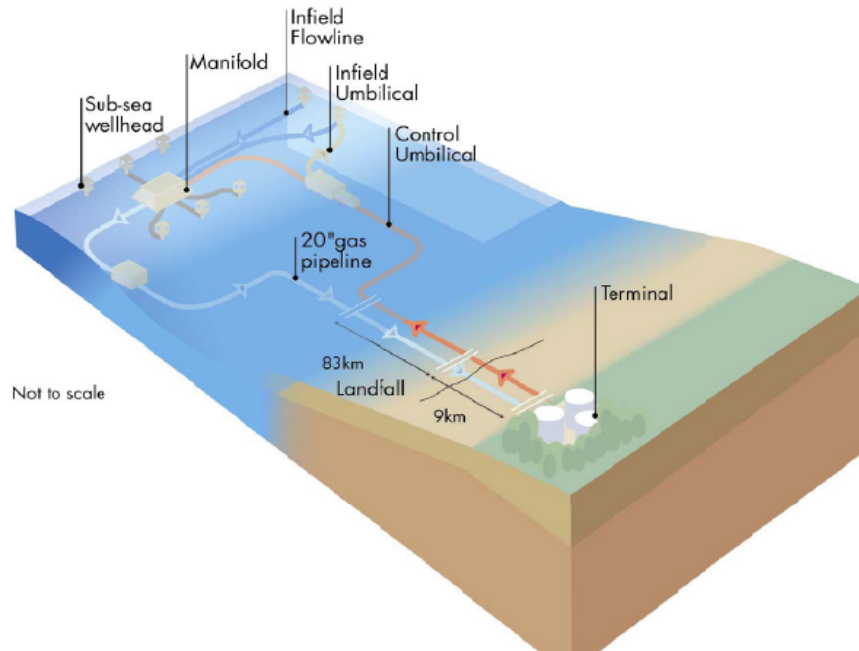
Fig VII.8 Subsea Tieback del campo corrió Propiedad Offshore magazine
