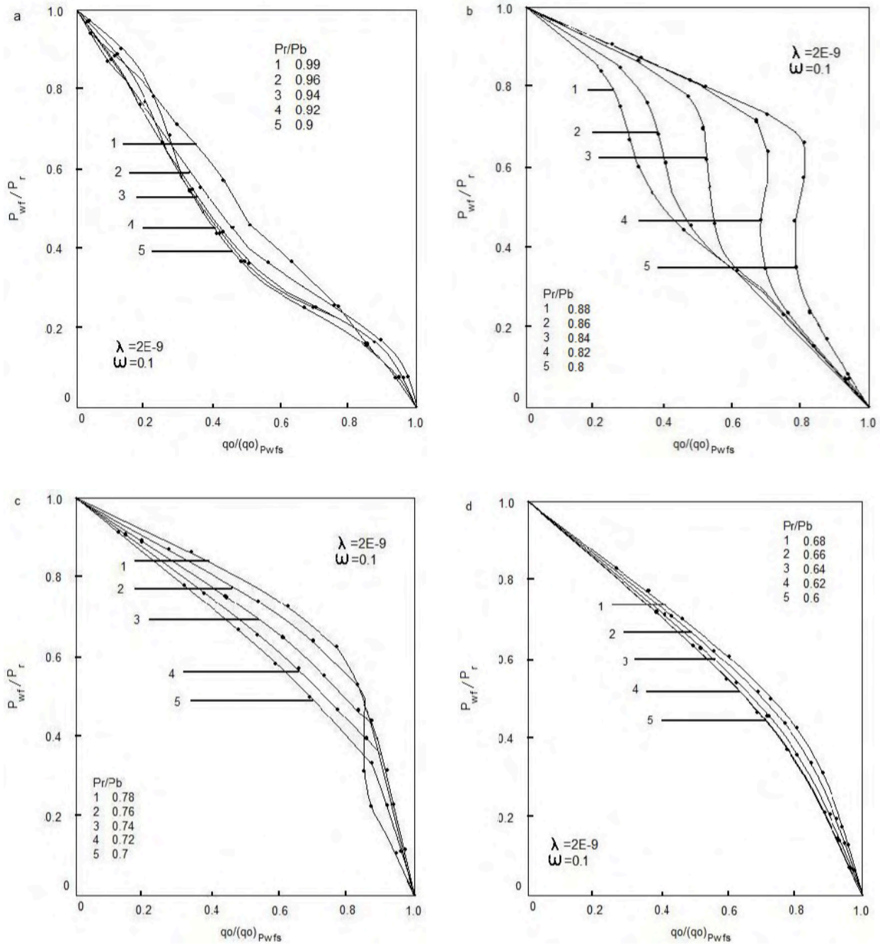
Figura (2.4) Curvas de IPR como función de la Presión Estática, para \lambda=2 \times 10^{-9} , k_m=0.001 , \omega=0.1 , y \text{°API}=45 (a) Pr/P_b=0.99 a 0.9 (b) Pr/P_b=0.88 a 0.8 (c) Pr/P_b=0.78 a 0.7 (d) Pr/P_b=0.68 a 0.6
