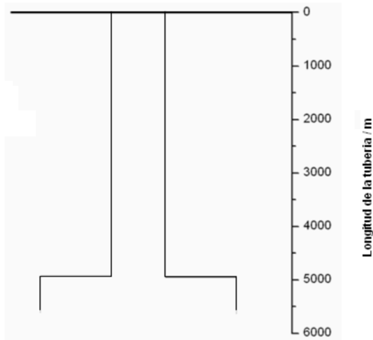
Figura (4.1) Estado mecánico del pozo estudiado.
