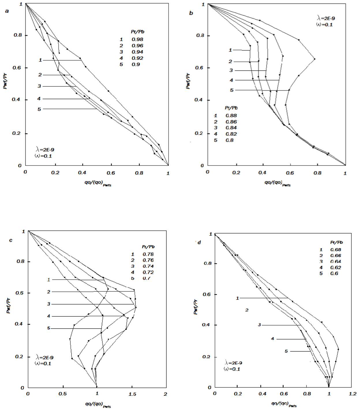
Figura (2.5) Curvas de IPR como función de la Presión Estática, para \lambda=2 \times 10^{-9} , k_m=0.001 , \omega=0.1 , y ^\circ \text{API}=35 (a) P_r/P_b=0.98 a 0.9 (b) P_r/P_b=0.88 a 0.8 (c) P_r/P_b=0.78 a 0.7 (d) P_r/P_b=0.68 a 0.6
