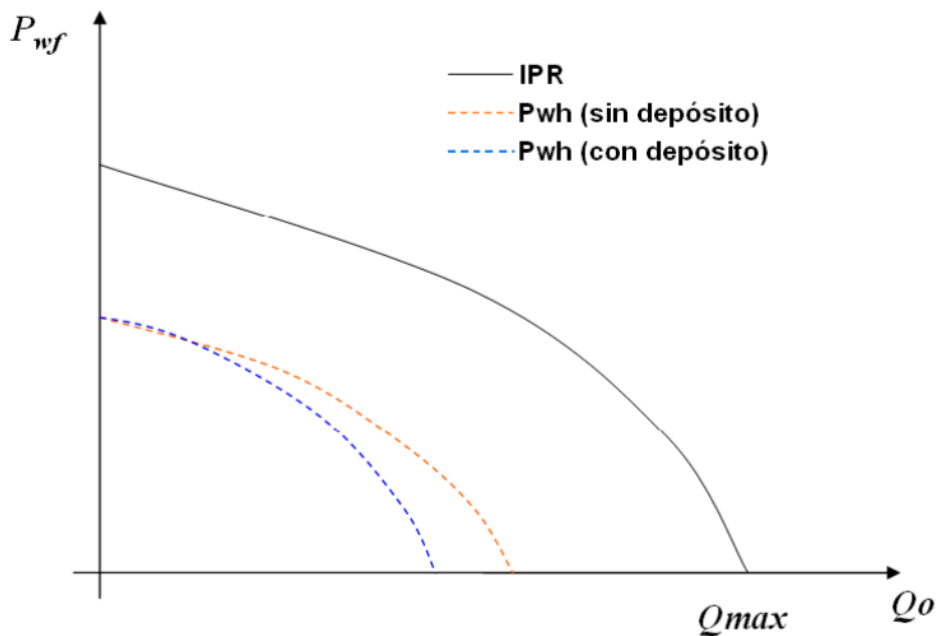
Figura (3.8). Cambio en la curva de presiones en la cabeza debido a la deposición de asfaltenos.
