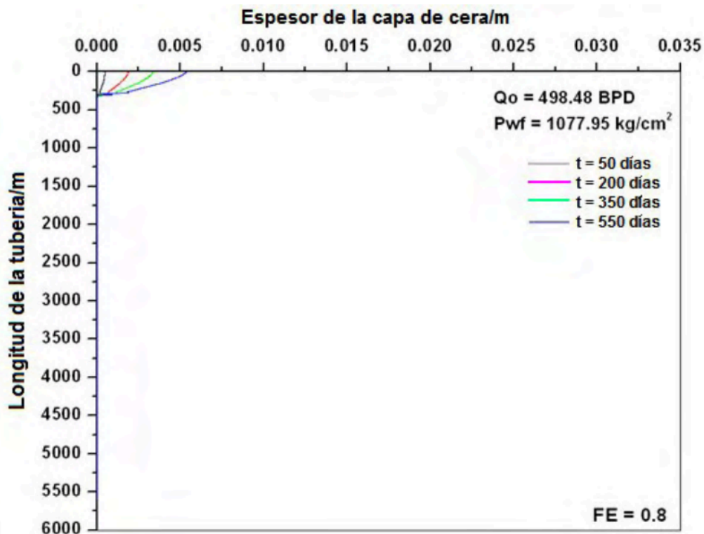
Figura (4.20) Perfiles de depositación de asfaltenos a lo largo de la tubería, para los diferentes tiempos de simulación, con los valores de 498.48 BPD y 1077.95 kg/cm 2 , tomando en consideración el daño a la formación.
