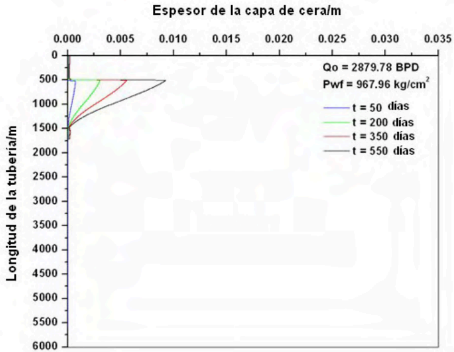
Figura (4.10) Predicción del grosor del depósito de asfaltenos para un gasto ( Q_o ) de 2879.78 BPD y una presión de fondo fluyendo ( P_{wf} ) de 967.96 kg/cm 2 considerando diferentes tiempos.
