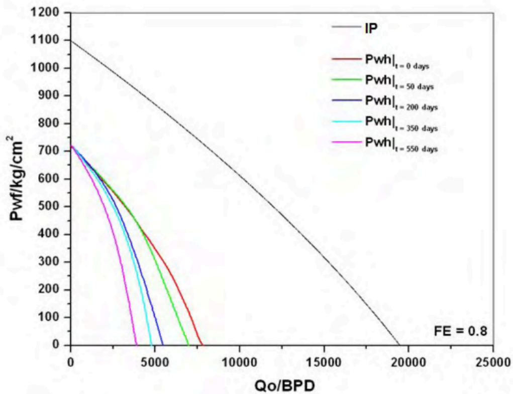
Figura (4.30) Reducción en el gasto de producción debido a la depositación de asfaltenos considerando los tiempos de simulación y el daño a la formación.
