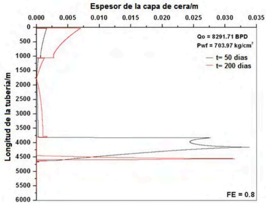
Figura (4.28) Perfiles de deposición de asfaltenos a lo largo de la tubería, para los diferentes tiempos de simulación, con los valores de 8291.71 BPD y 703.97 kg/cm 2 , tomando en consideración el daño a la formación.
