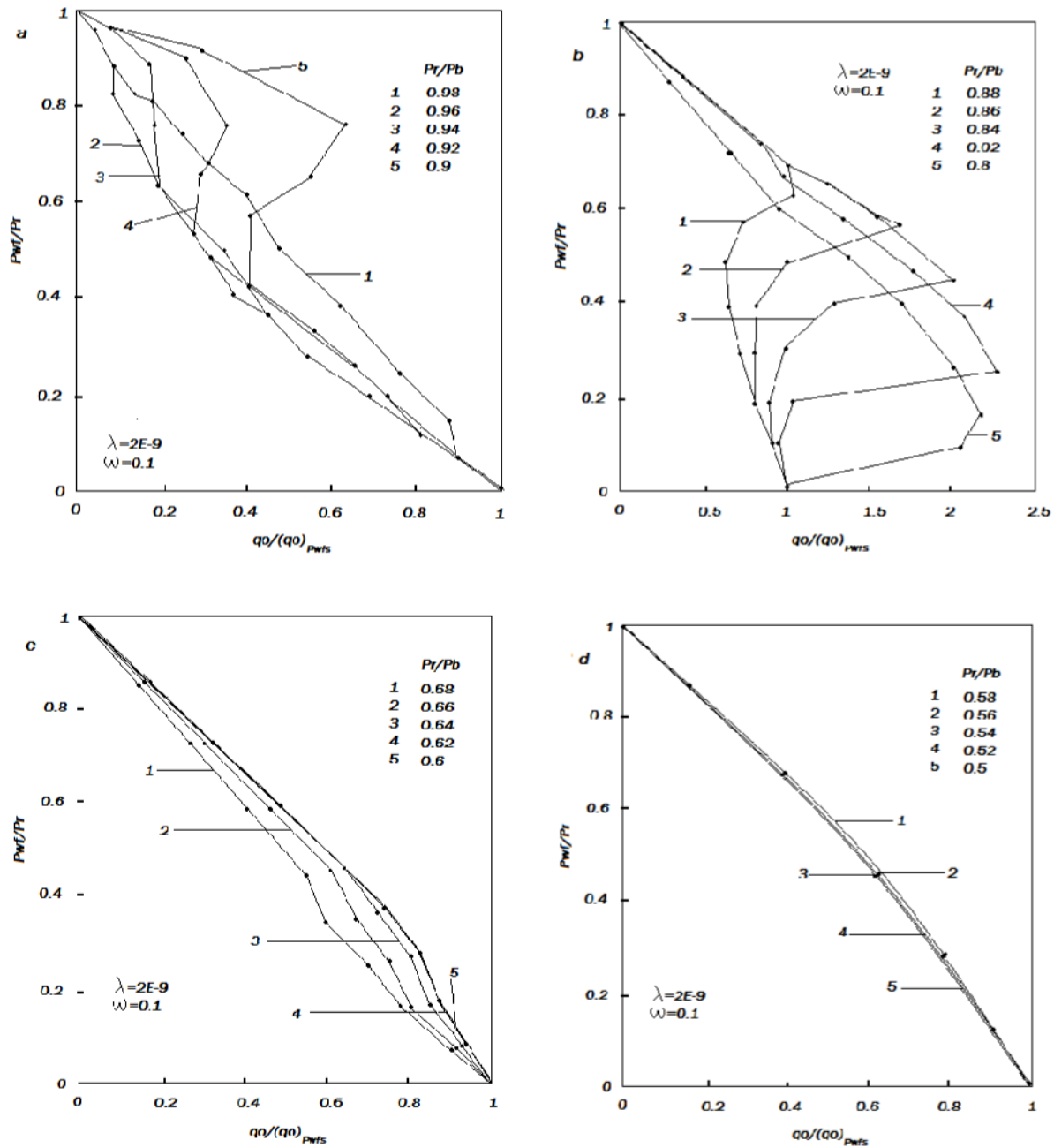
Figura (2.6) Curvas de IPR como función de la Presión Estática, para \lambda=2 \times 10^{-9} , k_m=0.001 , \omega=0.1 , y ^\circ\text{API}=25 (a) P_r/P_b=0.98 a 0.9 (b) P_r/P_b=0.88 a 0.8 (c) P_r/P_b=0.68 a 0.6 (d) P_r/P_b=0.58 a 0.5
