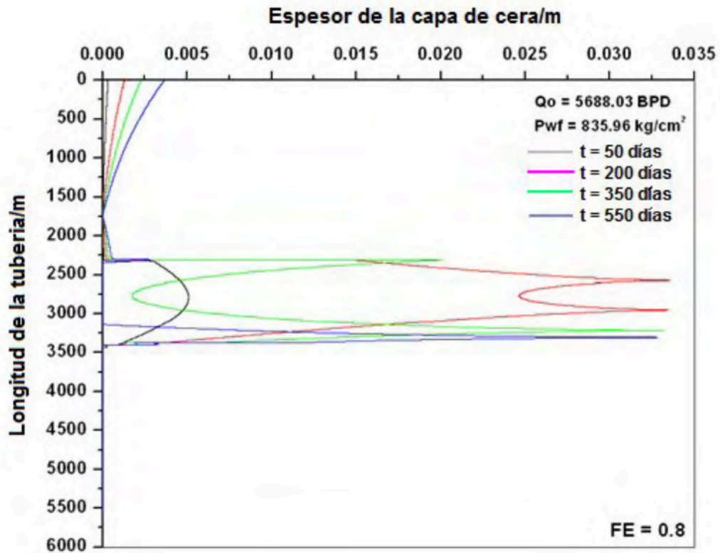
Figura (4.26) Perfiles de deposición de asfaltenos a lo largo de la tubería, para los diferentes tiempos de simulación, con los valores de 5688.03 BPD y 835.96 kg/cm 2 , tomando en consideración el daño a la formación.
