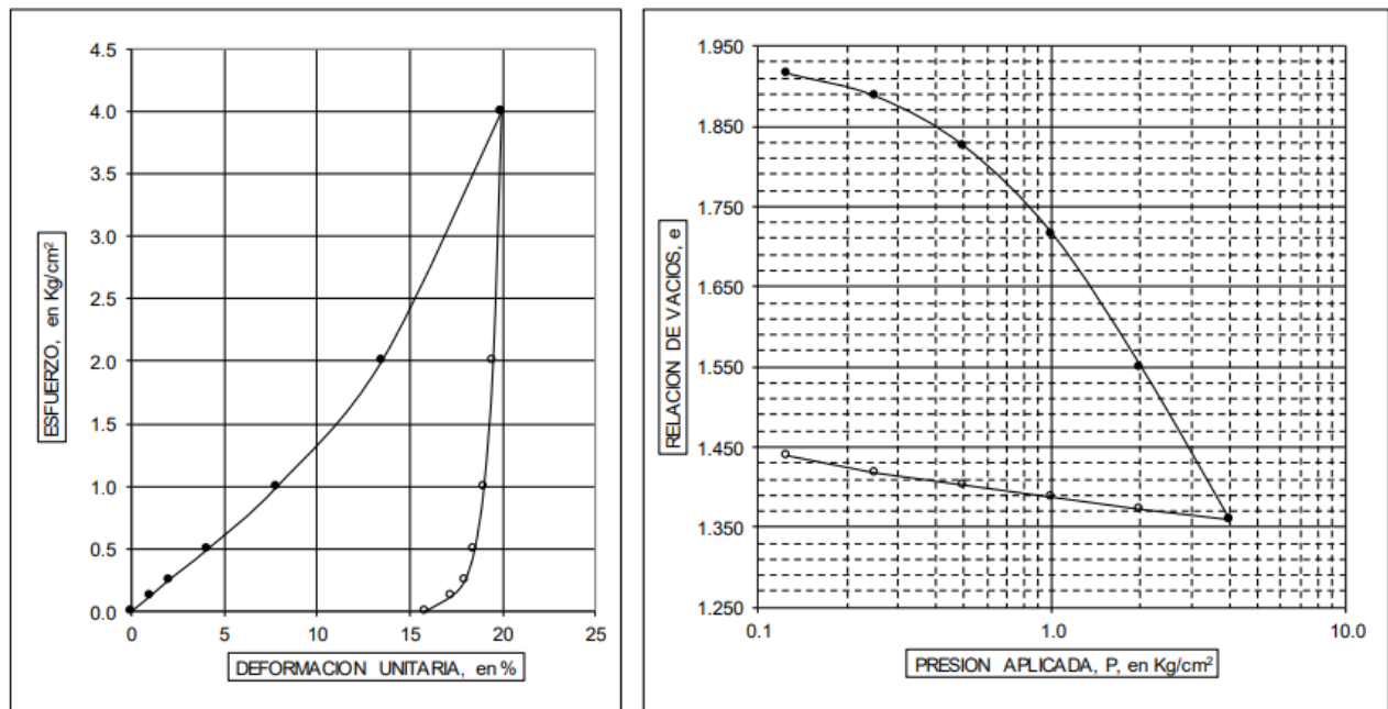
Figura 71. Consolidación unidimensional a 23.50-24.40 m
