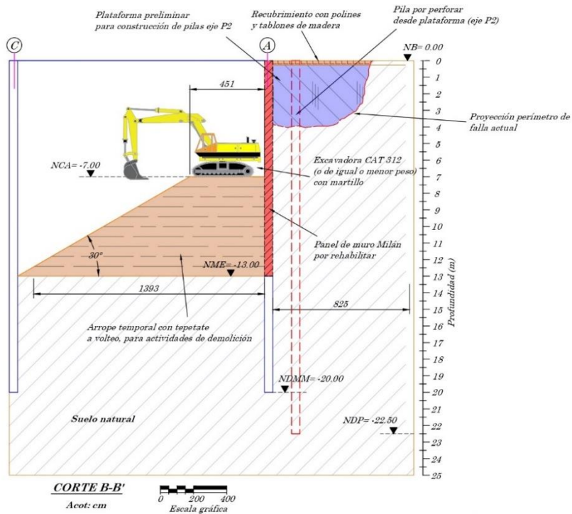
Figura 28. Arrope temporal frente a paneles colapsados para actividades de demolición mediante CAT 312 con martillo de 3 t.
