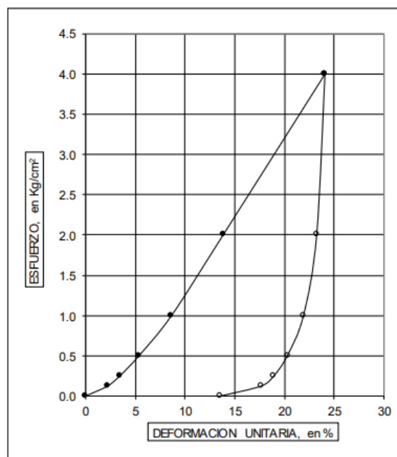
Figura 70. Consolidación unidimensional a 20.30-21.10 m
