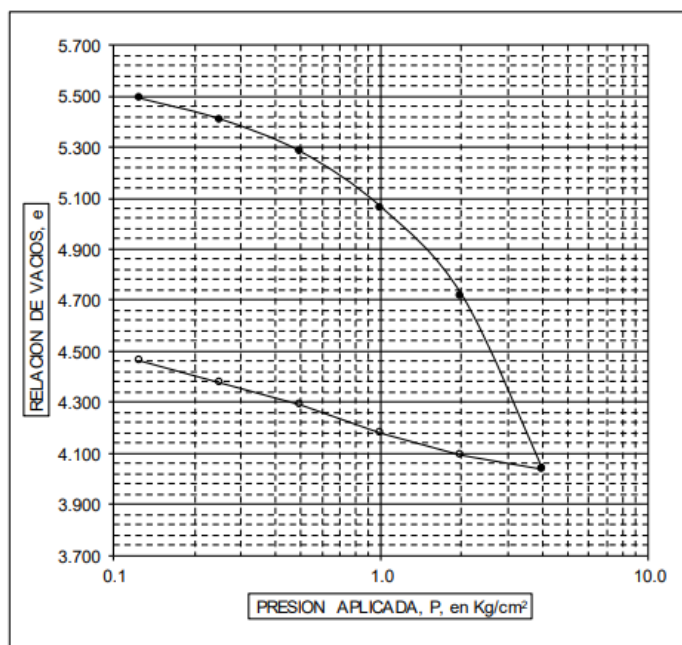
Figura 70. Consolidación unidimensional a 20.30-21.10 m
