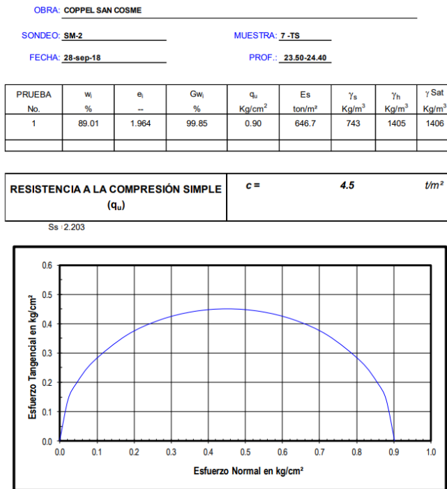
Figura 62. Compresión simple a 23.50-24.40 m
