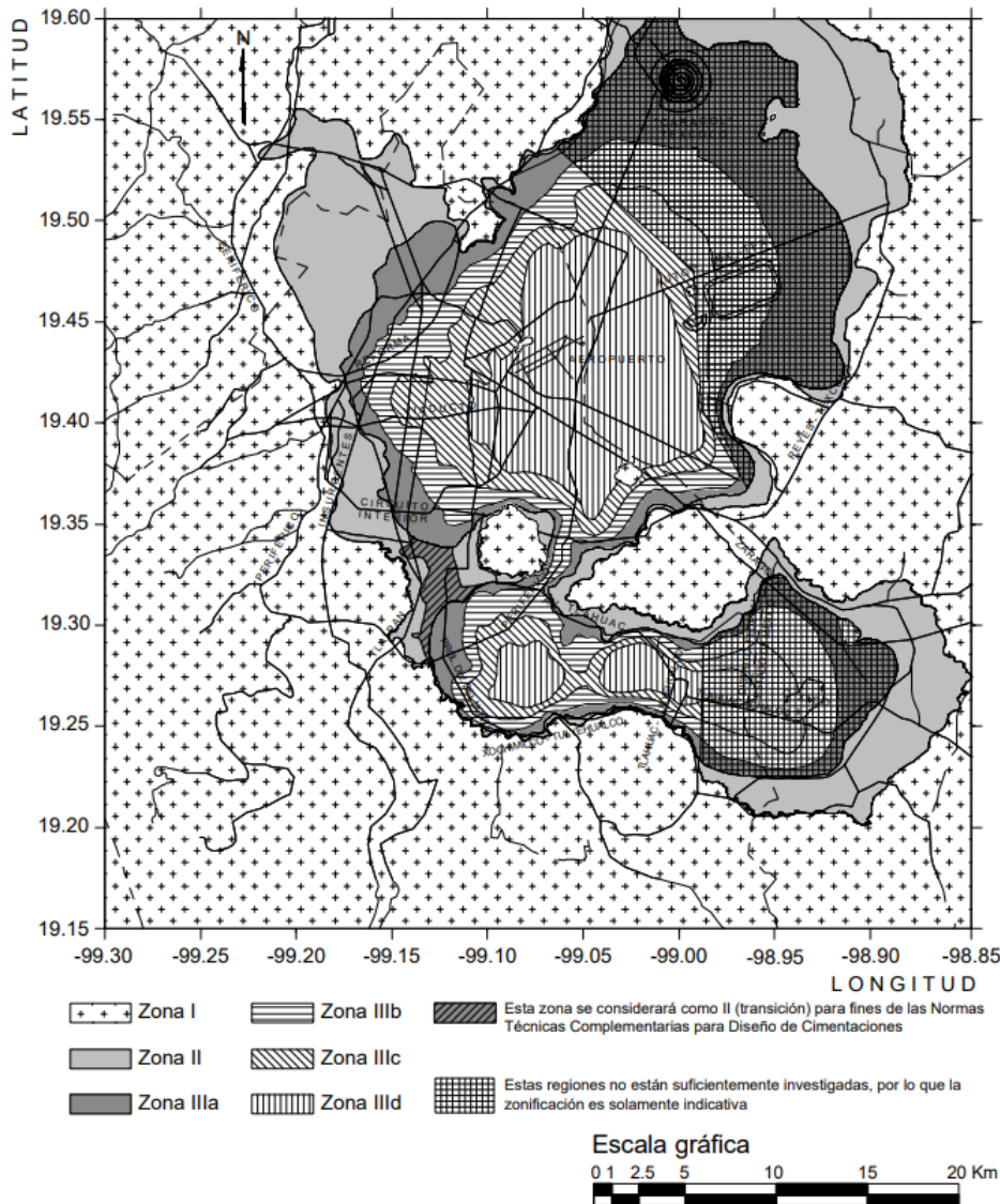
Imagen 3 Zonificación de CDMX para fines de diseño por sismo, obtenida de NTC-DS-2004
