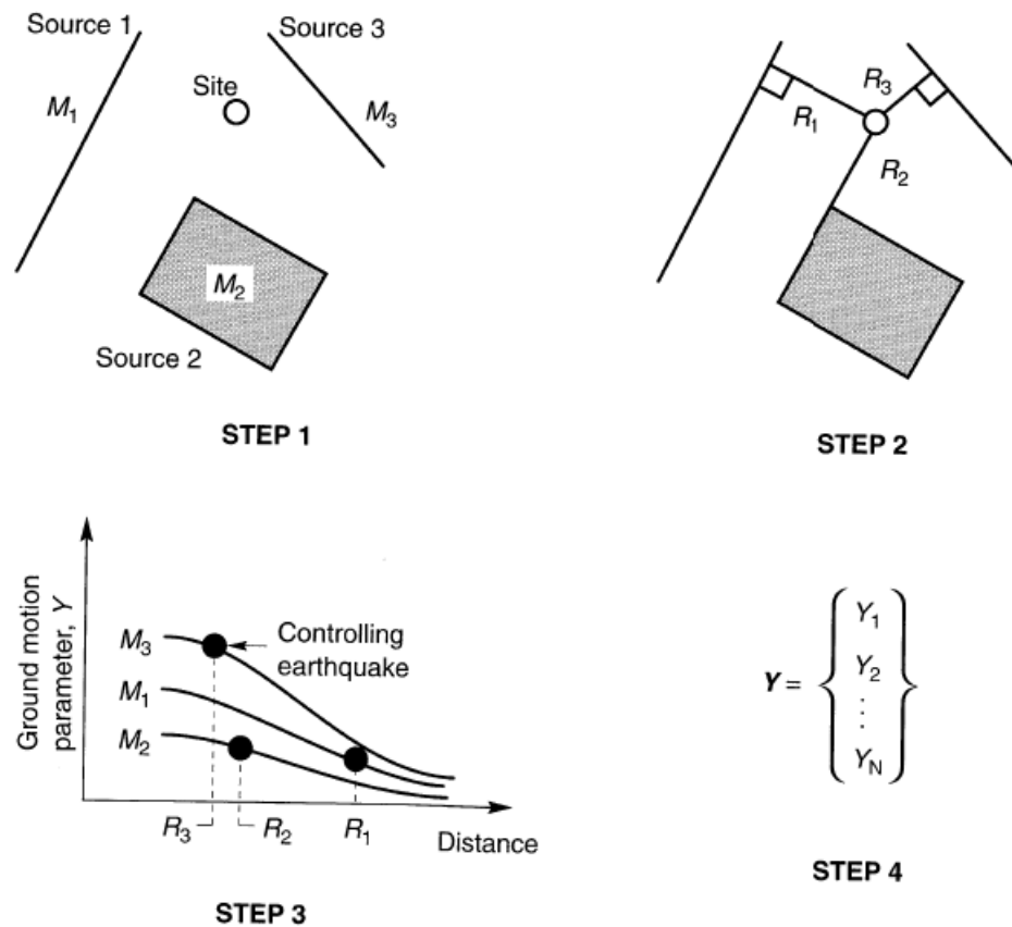
Imagen 1 Pasos del análisis determinista del peligro sísmico
