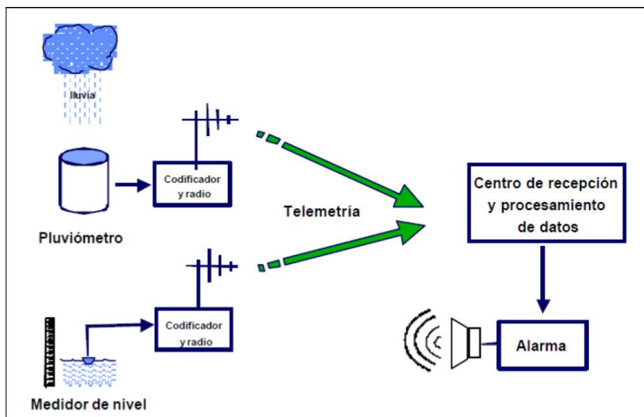
Imagen 7. Sistema de medición y alerta. Fuente: Rodríguez, 2012
