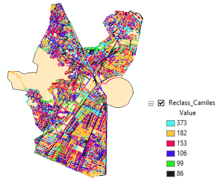
Imagen 57. Proceso e interpretación de la reclasificación de valores o pesos de importancia para las alternativas de los carriles que presentan las vías de comunicación terrestre en relación a las inundaciones en Ecatepec. Fuente: Elaboración propia.
