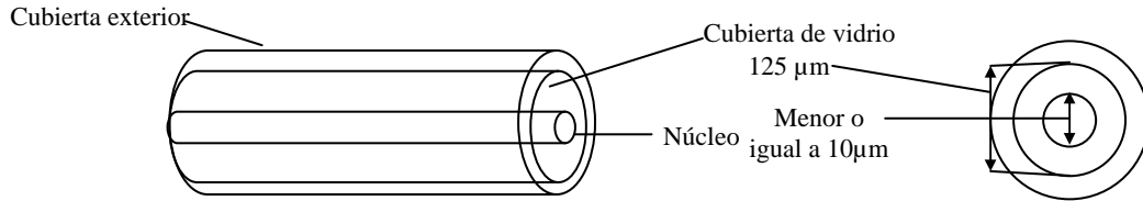
Fig. 1-19 Fibra óptica monomodo.
