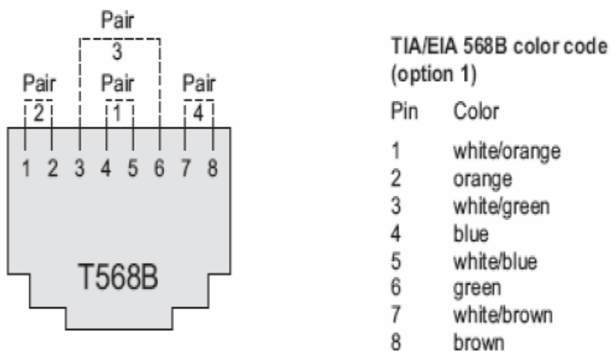
Fig. 3-10 Distribución T568B.
