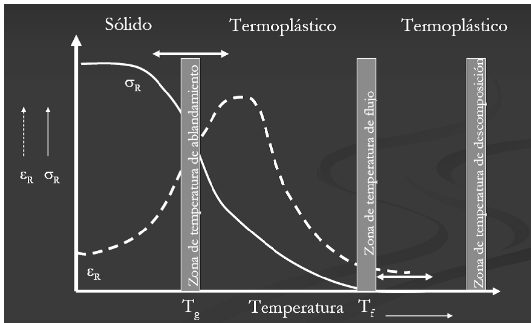
Fig. 5. Comportamiento térmico de plásticos amorfos.
