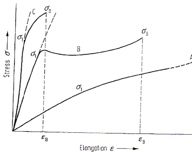
Fig. 10. Diagrama esfuerzo - deformación: A) elastómeros, B) termoplásticos y C) termofijos. vi
