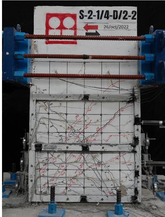
Fig. 3.3.130 Carga cero después de la distorsión del 3% - Columna C-2 (Instituto de Ingeniería, 2021 - 2023)
