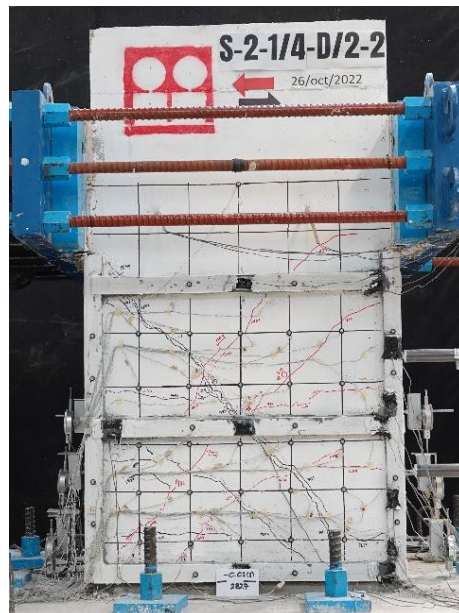
Fig. 3.3.120 Cara norte ( R=-2\%(2) ) - Columna C-2 (Instituto de Ingeniería, 2021 - 2023)
