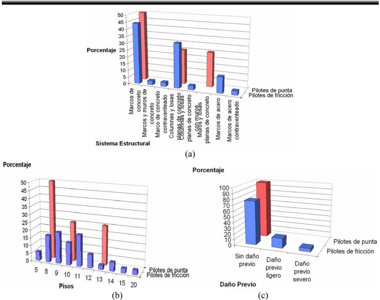
Figura 3.11 Estructuras dañadas en la delegación Cuauhtémoc por los sismos de septiembre de 1985 con cimentación profunda por: (a) Sistema Estructural, (b) Número de pisos, (c) Daño previo
