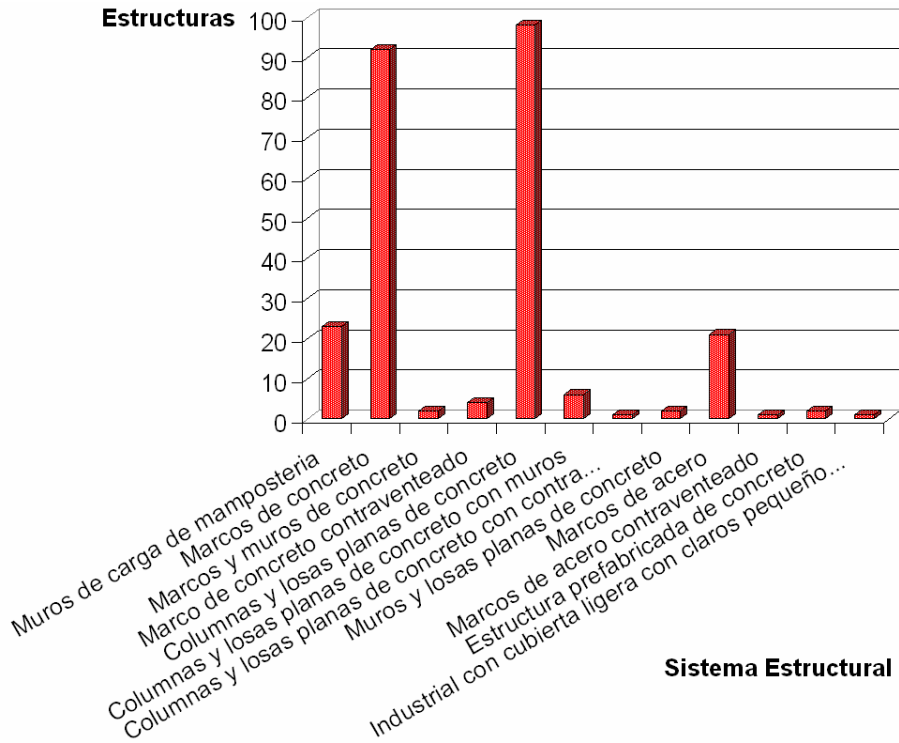
Figura 1.16 Estructuras dañadas en los sismos de septiembre de 1985 según el sistema estructural
