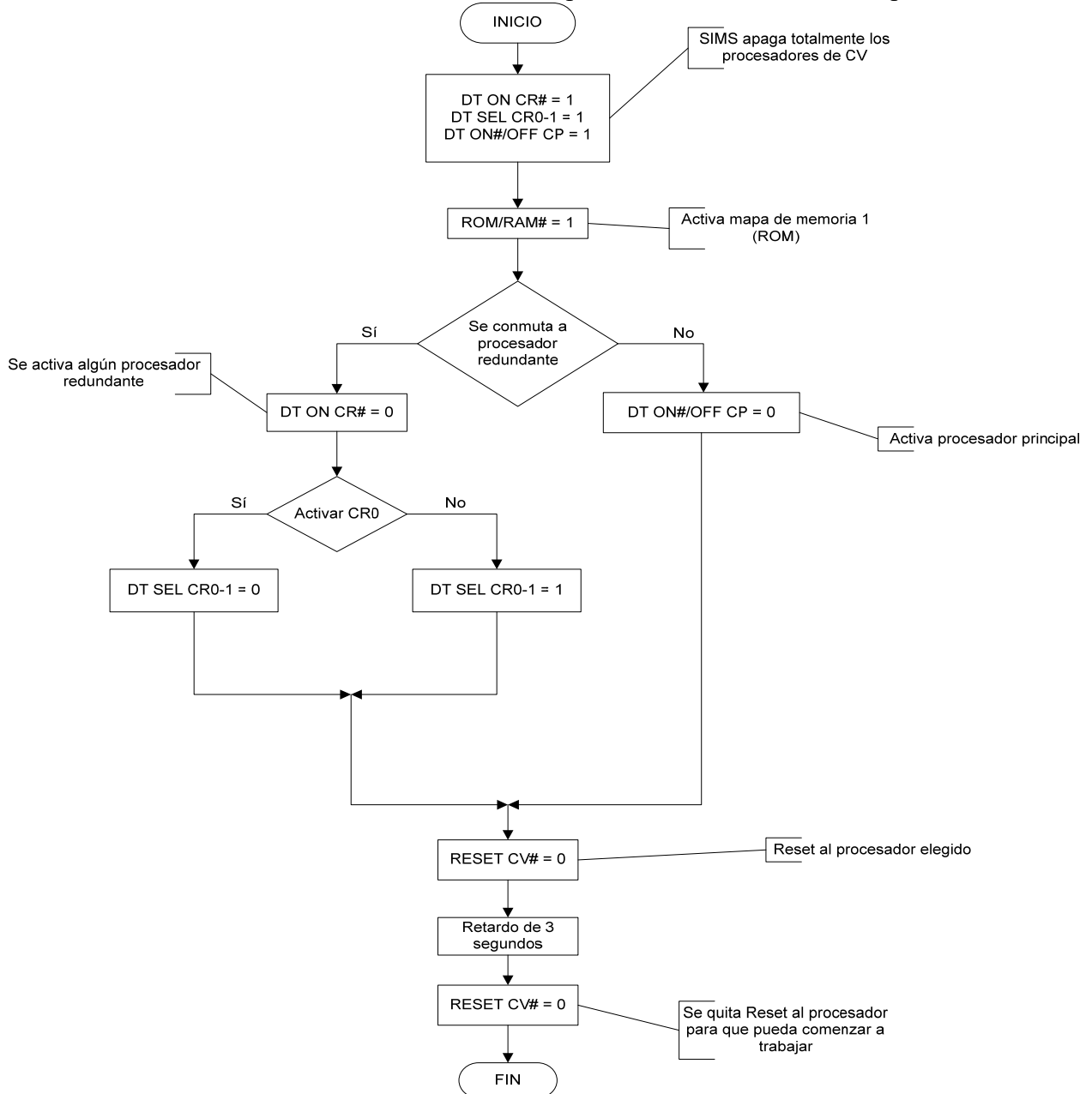
Figura 5.5 Conmutación de CV por parte del SIMS
