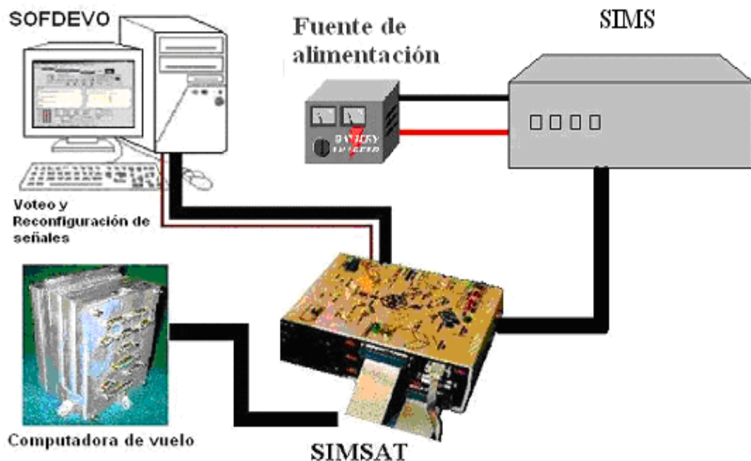
Figura 5.3 Equipo requerido para realizar pruebas de integración entre SIMS y CV
