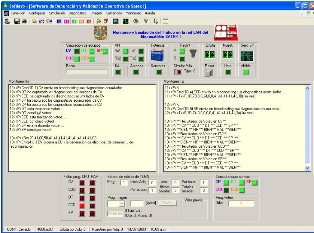
Figura 4.5 Resultado del proceso de voto en el experimento de MACV
