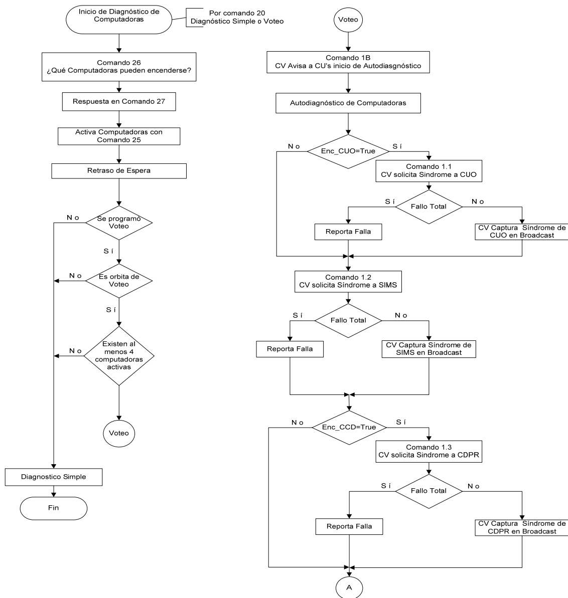
Figura 2.6.1 Diagrama de flujo del experimento de MACV
