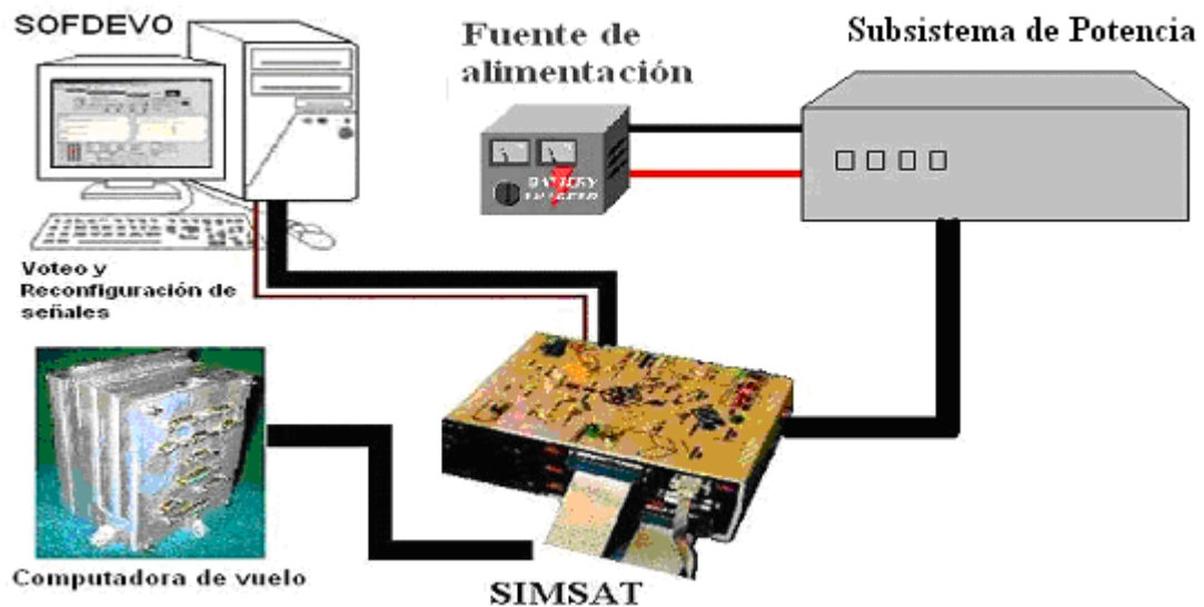
Figura 5.1 Equipo requerido para la realización de pruebas de comunicación entre los modelos de vuelo de subsistemas inteligentes del satélite y la computadora de vuelo.
