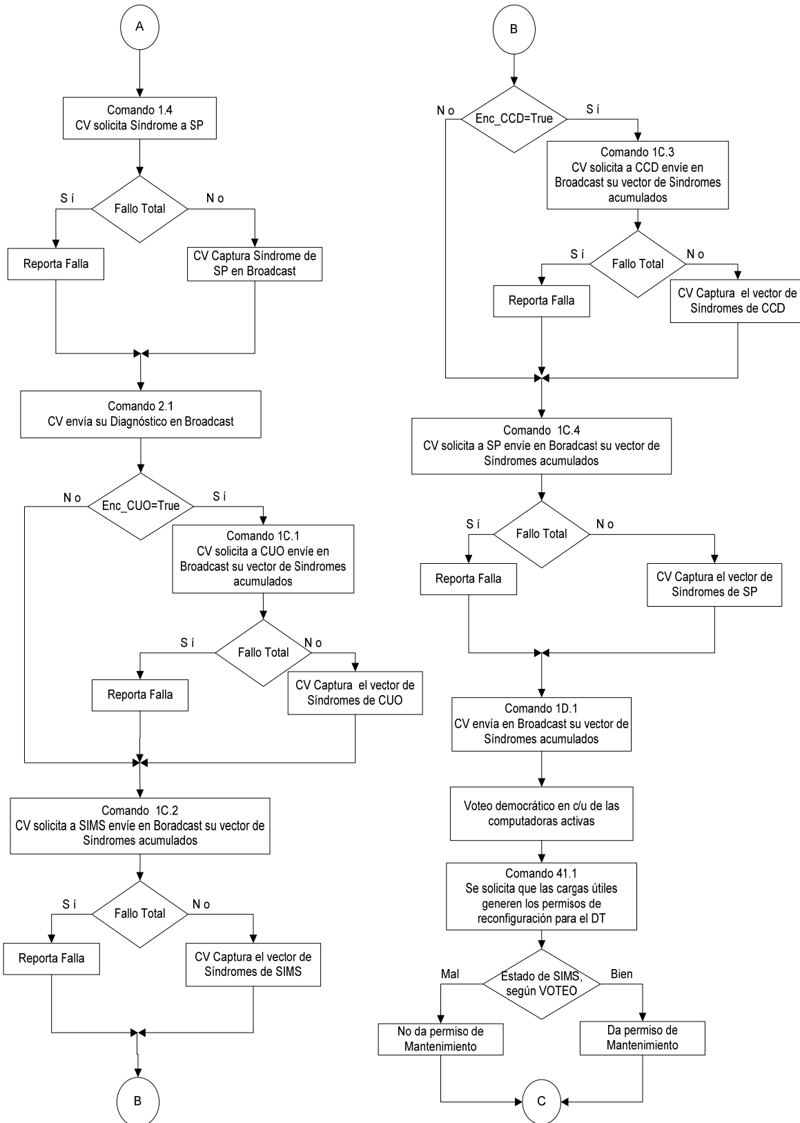
Figura 2.6.2 Diagrama de flujo del experimento de MACV
