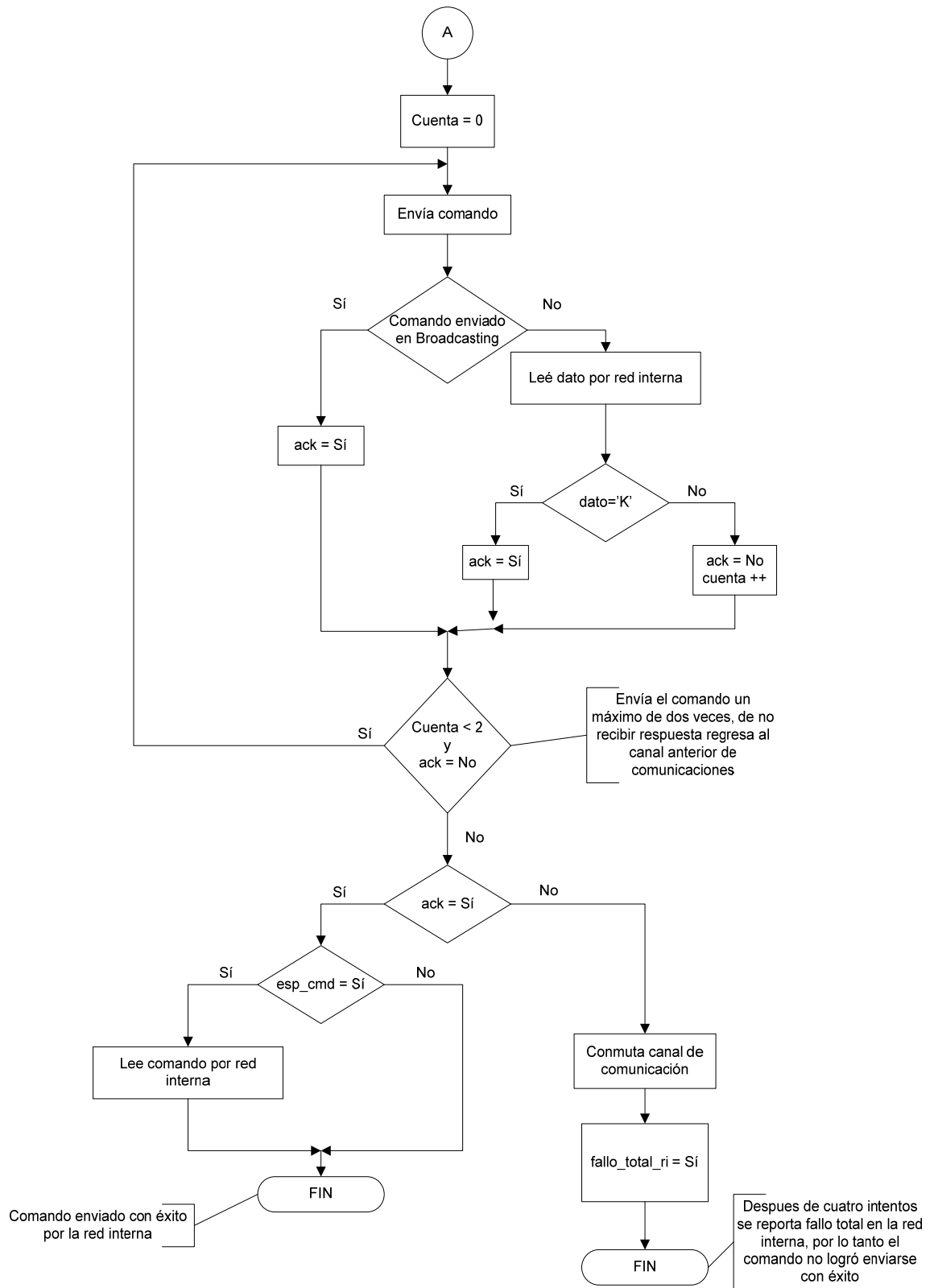
Figura 2.2.2 Protocolo de envío de información por red interna
