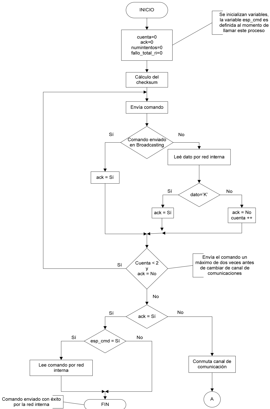
Figura 2.2.1 Proceso de envío de información por red interna
