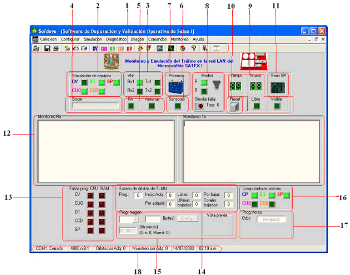
Figura 2.1 Pantalla principal de SOFDEVO
