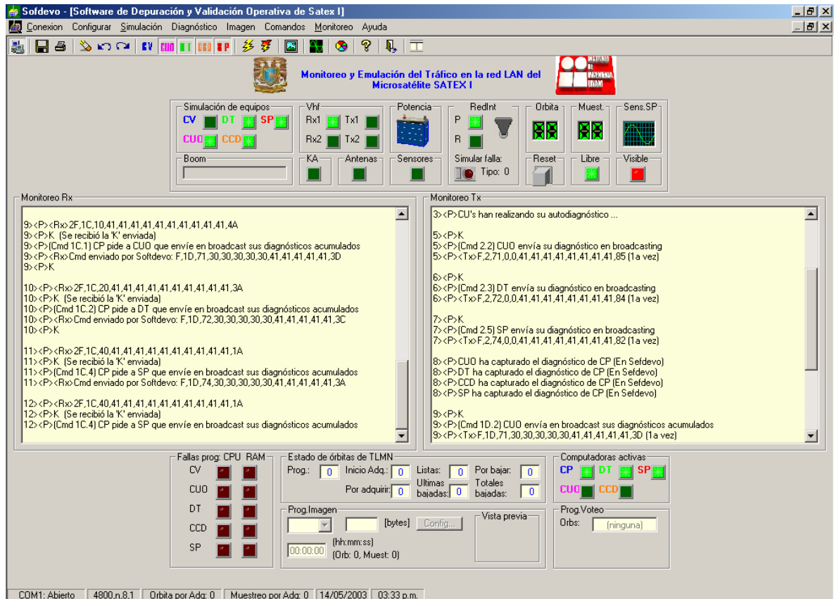
Figura 2.4 Respuestas automáticas de SOFDEVO asociados con el experimento de MACV
