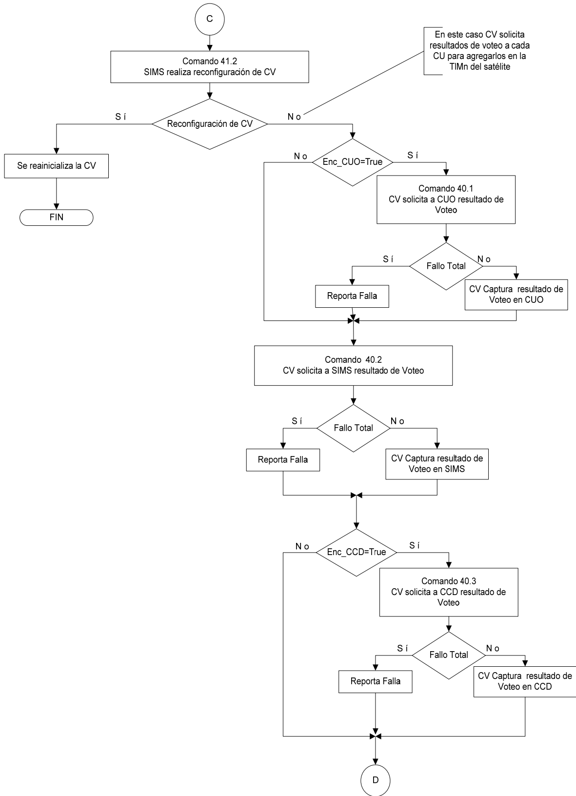
Figura 2.6.3 Diagrama de flujo del experimento de MACV
