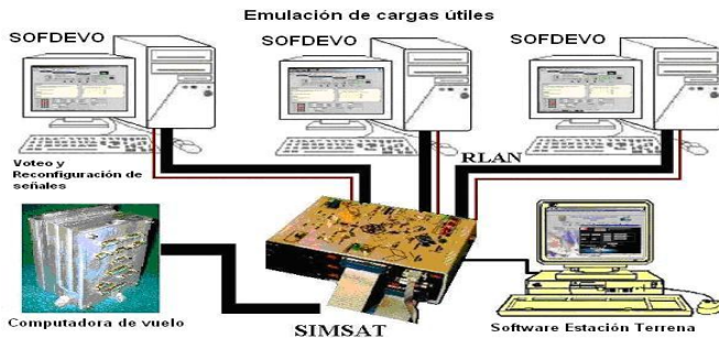
Figura 1.3 Equipo requerido para realizar el experimento de MACV
