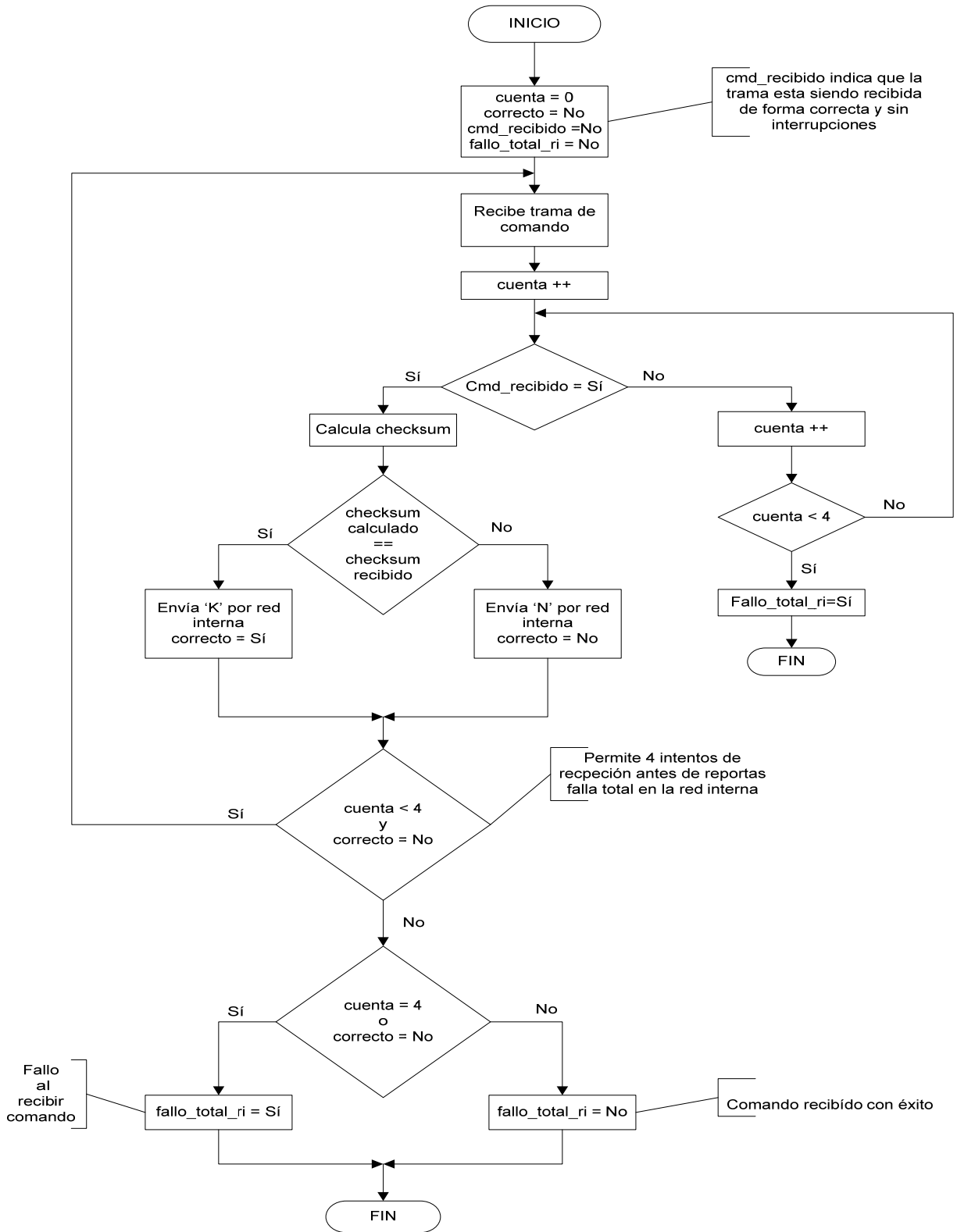
Figura 2.3 Protocolo de recepción de información
