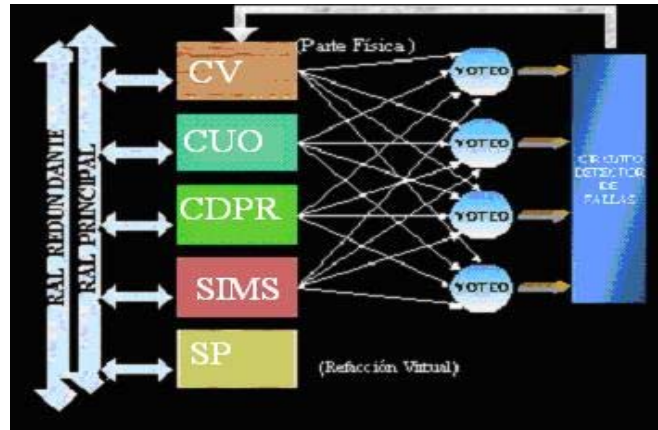
Figura 1.2 Arquitectura de cómputo semivirtual tolerante a fallas
