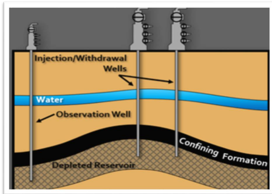
Figura 76. Tipos de pozos (underground-storages, 2022).
