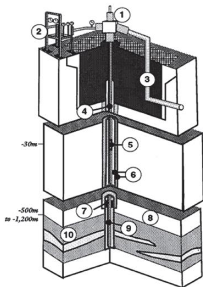
Figura 78. Acondicionamiento típico de un pozo de almacenamiento (Energía S. d., 2017).
