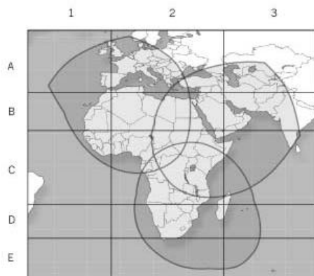
Fig. 6.6 Cobertura WorldSpace en Africa
