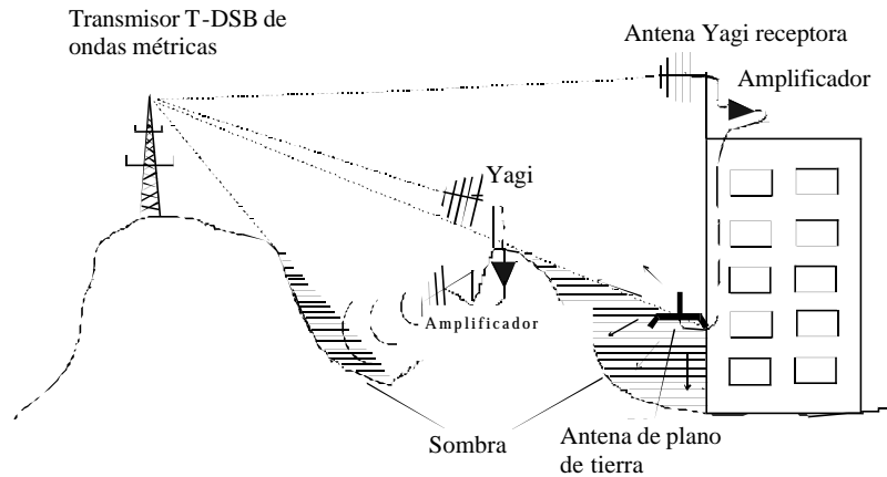
Fig. 1.11 Transmisor de relleno
