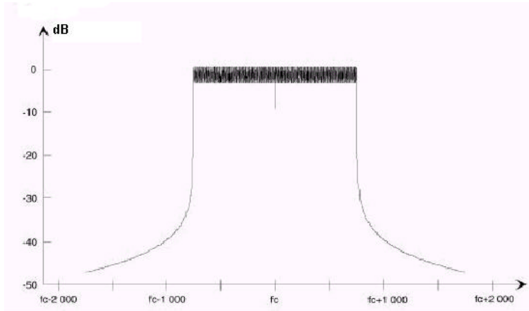
Fig. 1.5 Espectro del Modo I DAB, 1536 portadoras.
