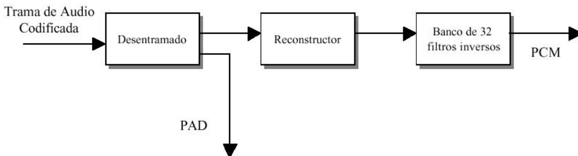
Fig. 1.3 Decodificador DAB
