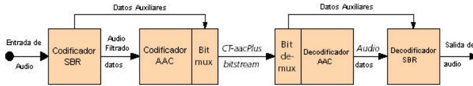
Fig.3.6 Sistema de codificación CT-aacPlus
