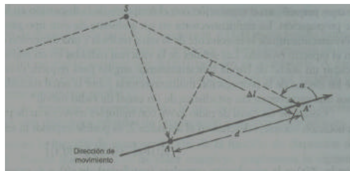
Fig.2.3 Corrimiento Doppler
