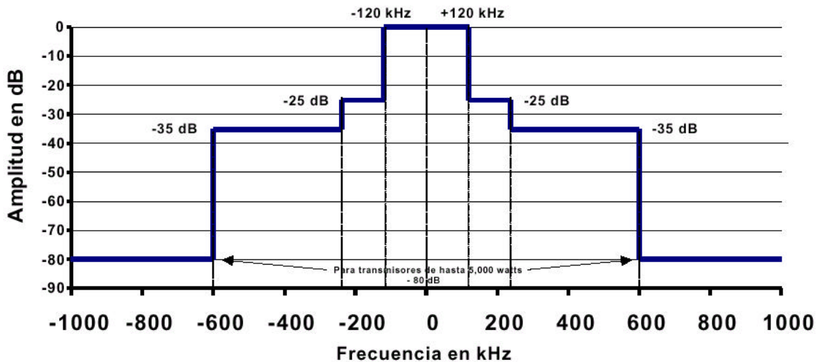
Fig. 2.4 Mascara para la Emisión de FM
