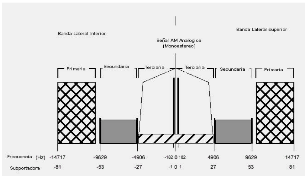
Fig. 2.5 IBOC Híbrido
