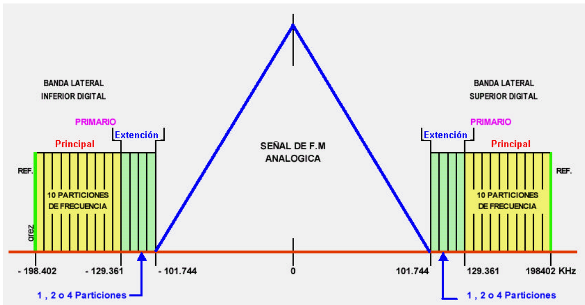
Fig.2.8 IBOC Híbrido Extendido
