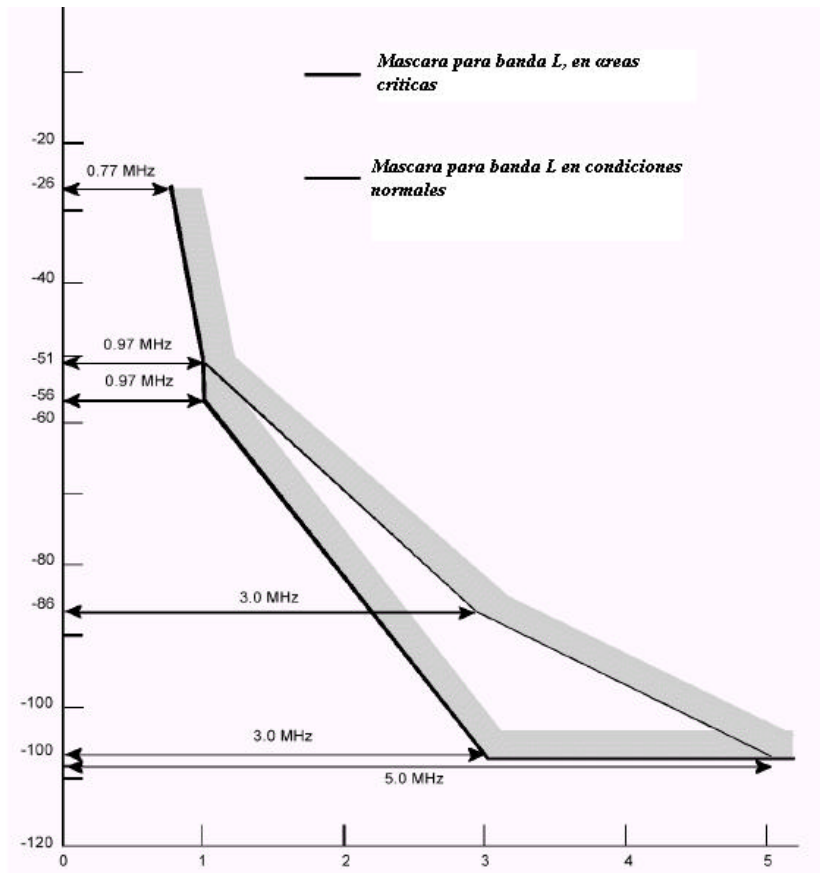
Fig. 1.6 Mascara Para Banda L
