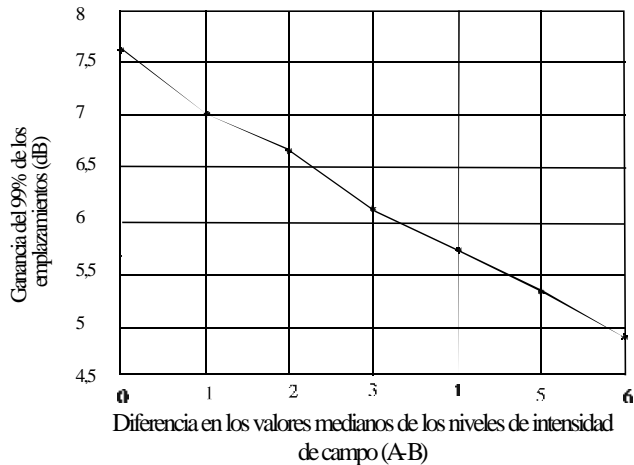
Figura 1.12 Ventajas de la Planificación de la SNF
