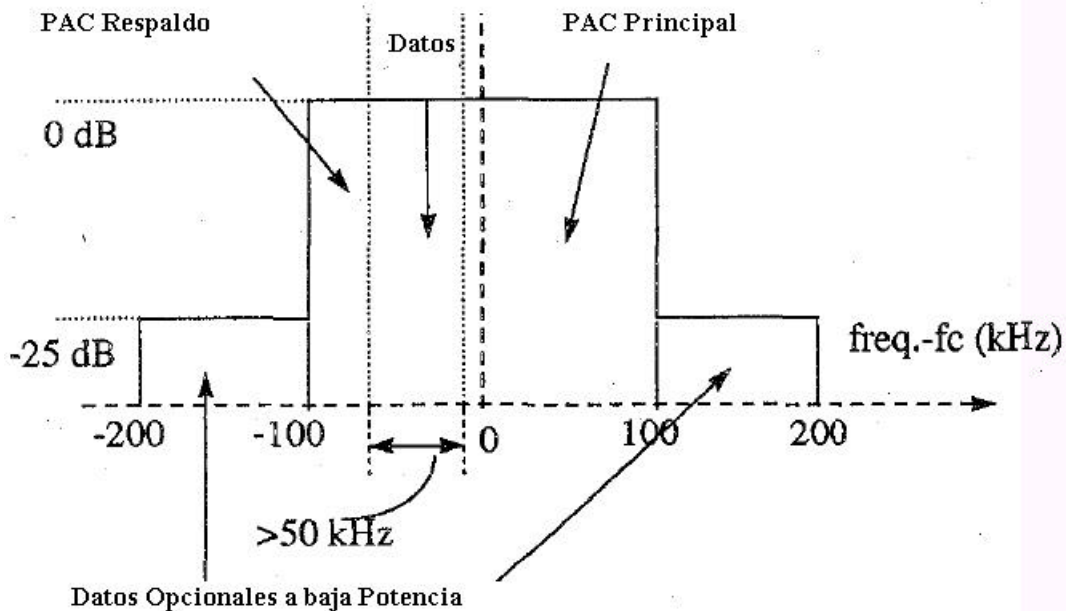
Fig. 2. 10. Mascara y Ancho de banda de FM IBOC Digital.
