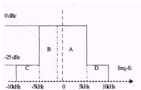
Fig. 2.2 Frecuencia digital AM-IBOC. División de la mascara y ancho de banda.
