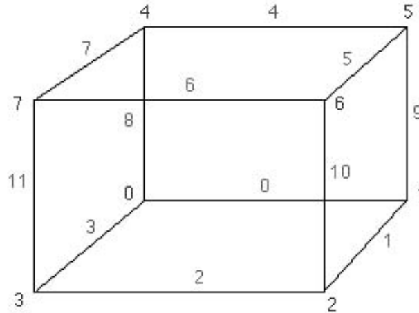
Figura 4.2.1 Notación para los vértices y aristas de los voxeles.
