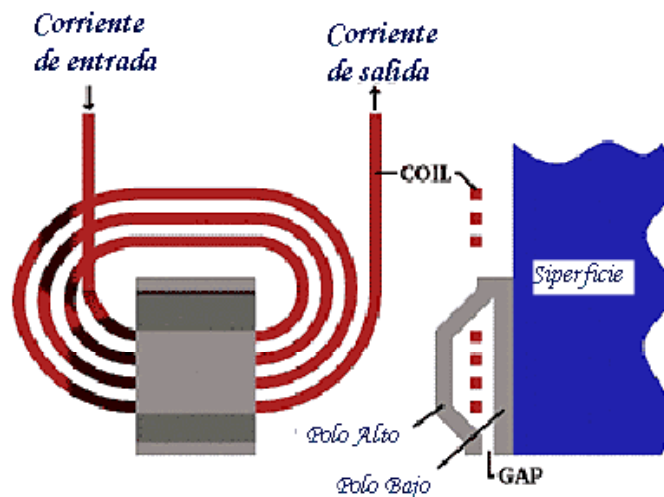
Fig. B.1 Una cabeza de escritura
