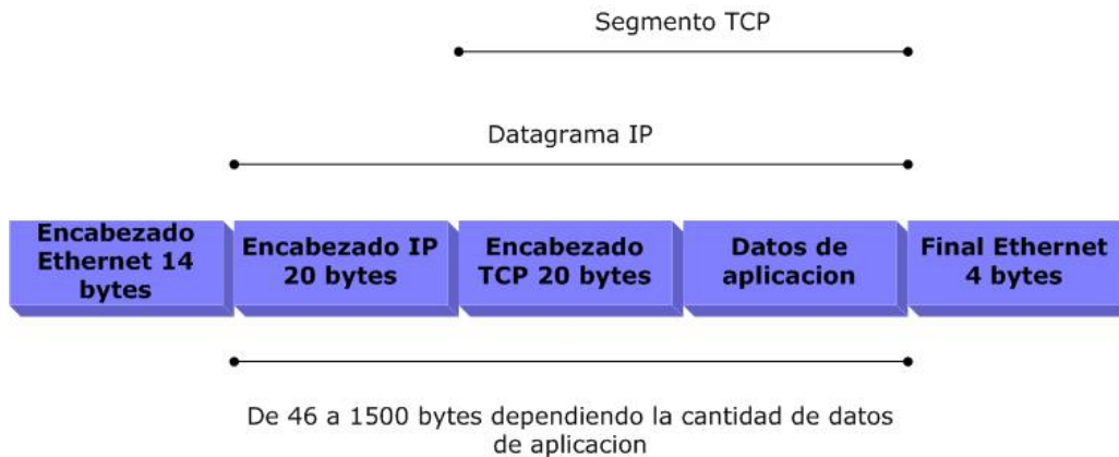
Un Frame Ethernet con los encabezados de todos los componentes de un paquete TCP
