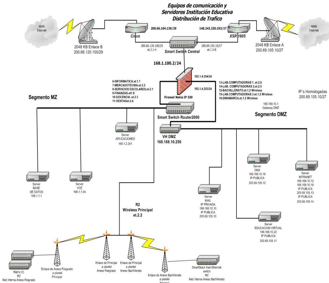
Figura 2.14: Diseño final.
