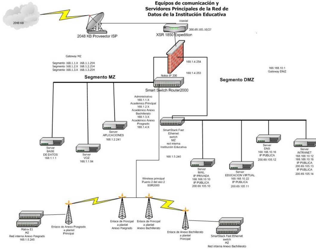
Figura 2.12: Red Institución Educativa con equipos de enlace de microondas de 11 Mbps.
