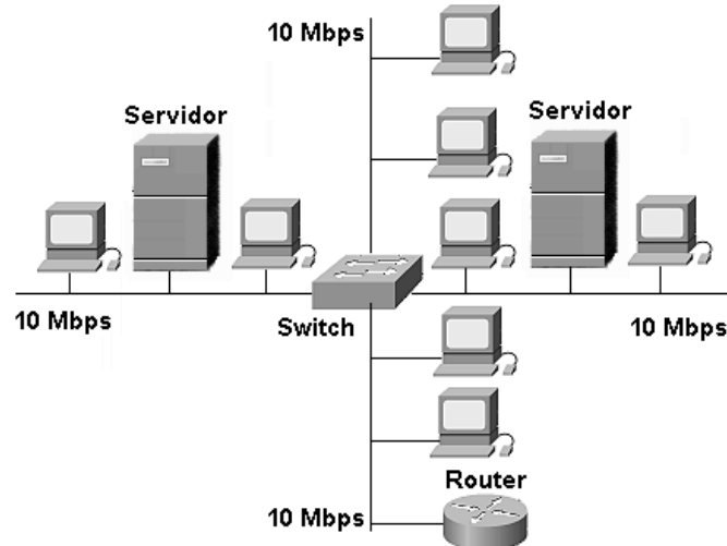
Figura 3.6 Conmutación simétrica
