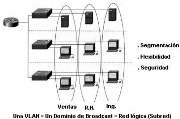
Figura 4.13 Vista global de una VLAN
