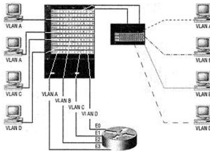
Figura 3.10 Asignación de puertos de uno mas switches a una VLAN
