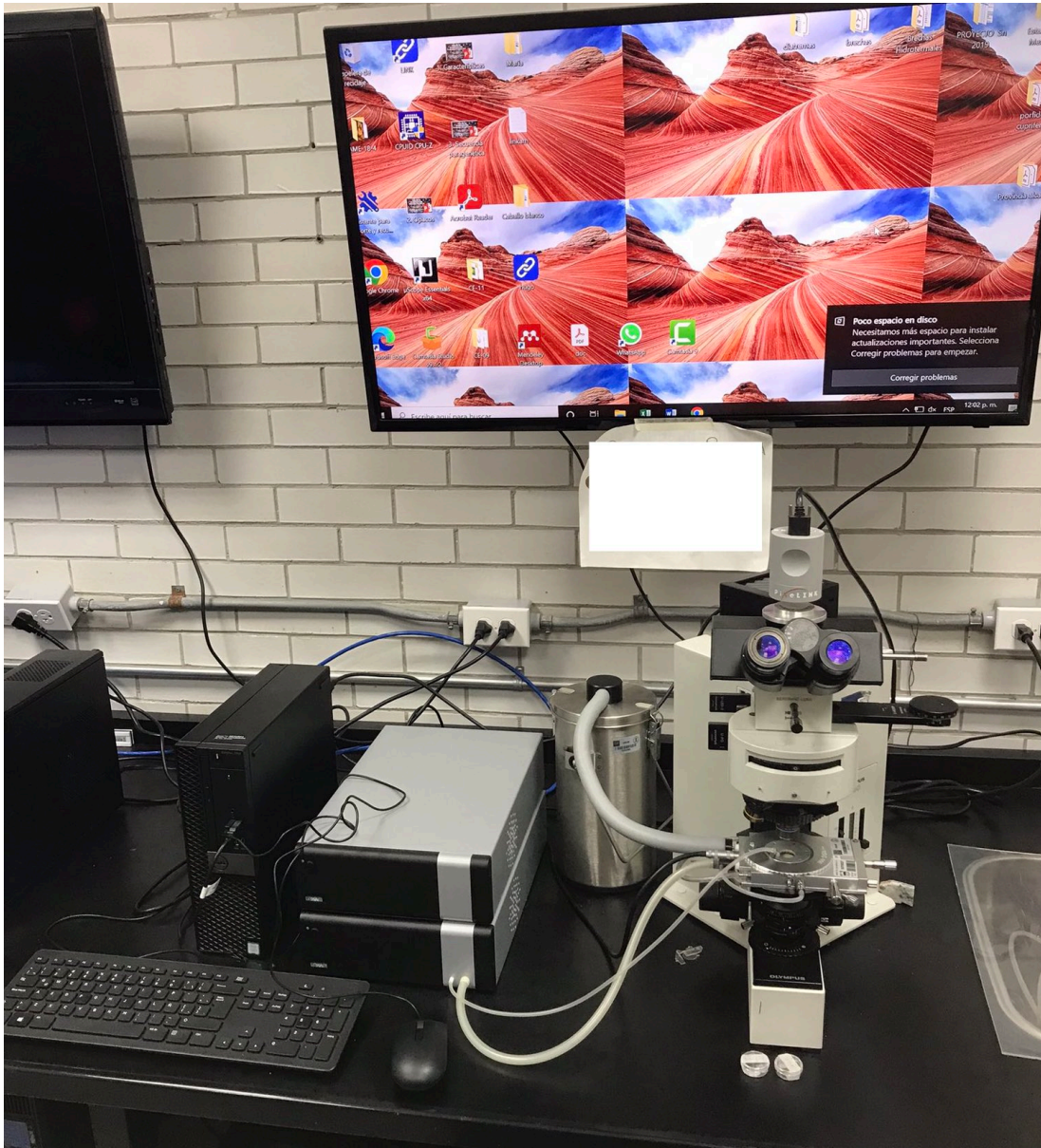
Figura 3.3. Platina microtermométrica Linkam THMSG 600 y microscopio Olympus.
