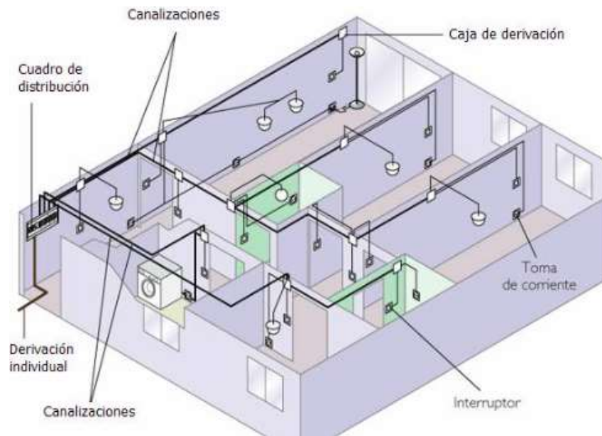
Figura 55 Instalación eléctrica
