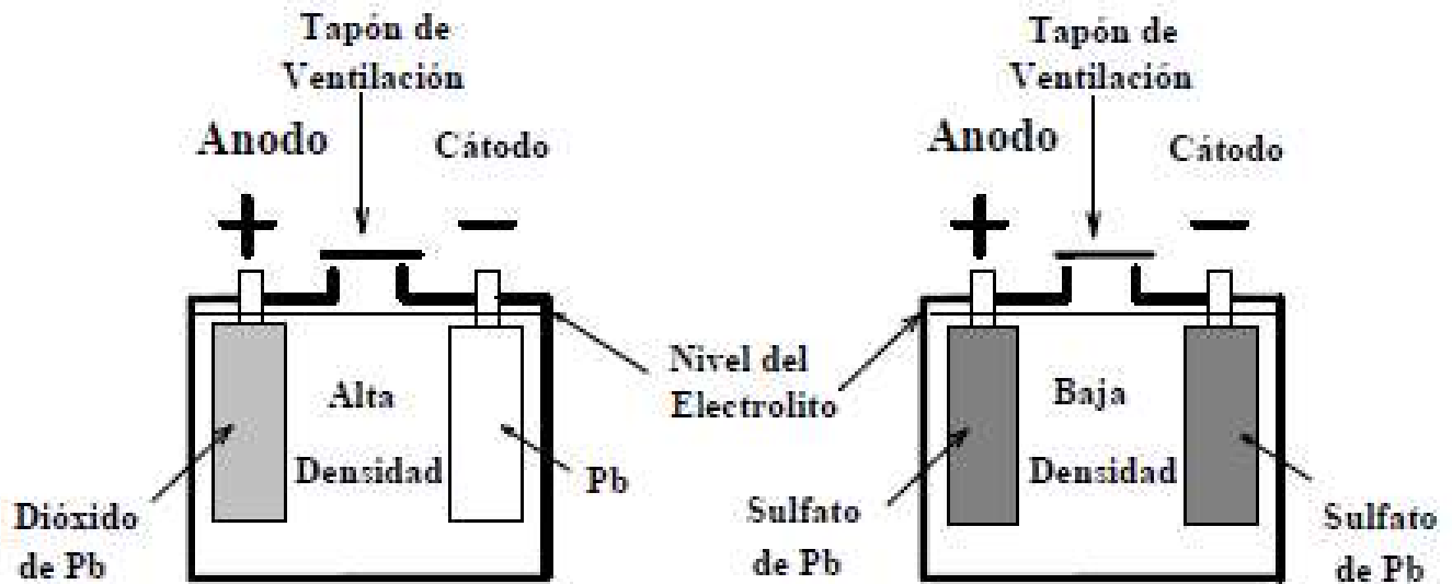
Fig. 5.1- Batería Cargada
